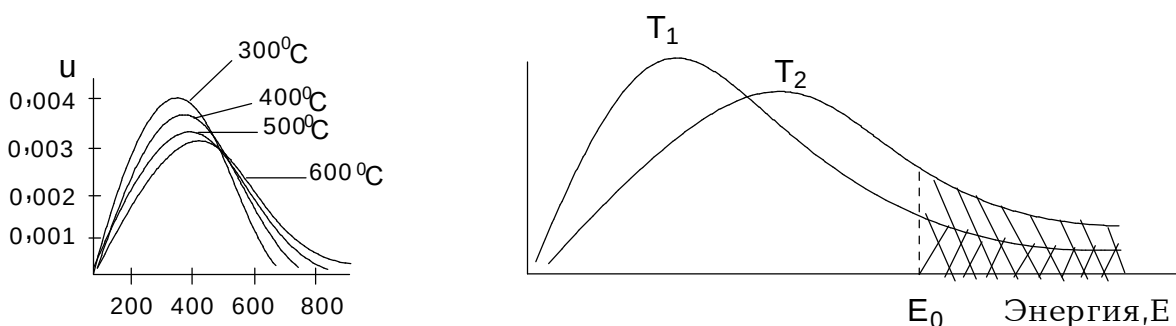
11 – расм. Ҳар хил ҳароратларда N_2O_5 учун молекулалар тезлигининг ҳарорат бўйича тақсимланиш эгриси, ( u – тезлиги ва V ва V+0,01 м/с оралиғида ётган молекулалар фоизи).
