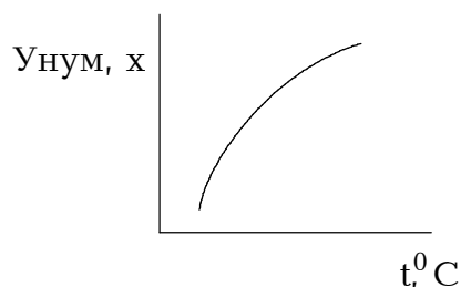
9 – Расм: Қайтар эндотермик реакция учун реакция маҳсулоти унумининг ҳароратга боғлиқлиги.
