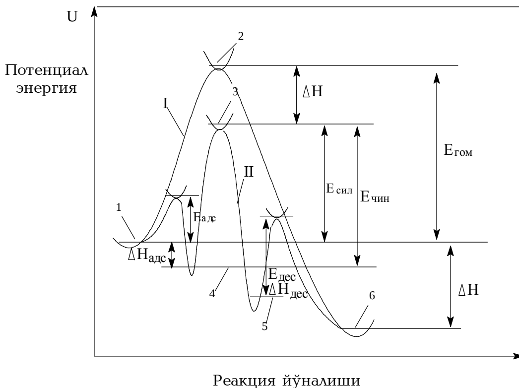
21 – рasm. Потенциал энергиянинг гомоген газ фазадаги реакция (1) ва гетероген – каталитик реакция (2) лар учун ўзгариш схемаси.
