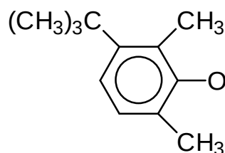
2,4,6-третертилфеноксил радикали
