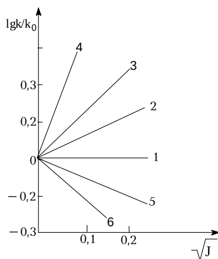
5.Расм. Эритмада борадиган реакция тезлик доимийси логарифмасининг ( \lg k/k_0 ) ион кучига ( \sqrt{I} ) боғлиқлик графиги Z_A Z_B қиймати қуйидагича:
