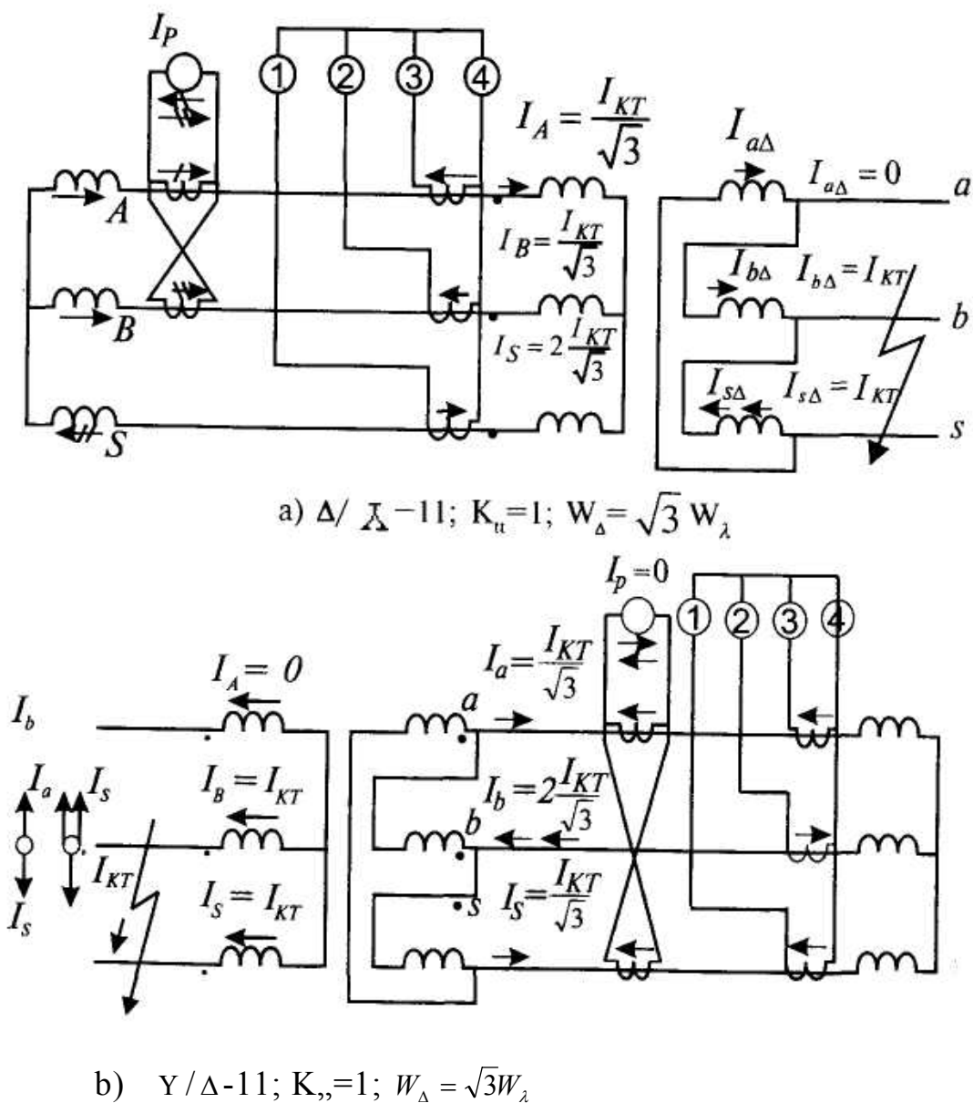
3.3.-rasm: a- \Delta/\Delta ; b- Y/\Delta ulangan transformatoridan keyin bo'ladigan ikki fazali qisqa tutashiv toklarning tarqalishi va vektor diagrammalari.
