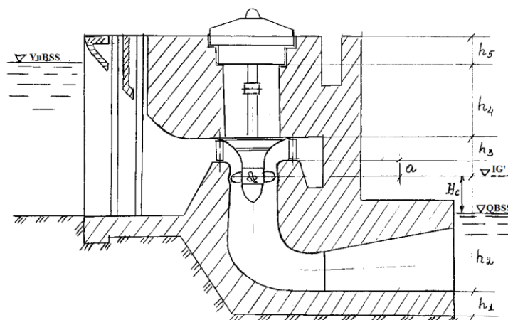
5.4-rasm. Binoning pastki qismi vertikal oʻlchamlari.
