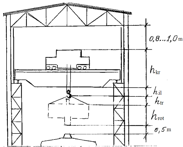
5.6-rasm. Bino yuqori qismi o'lchamlari.
