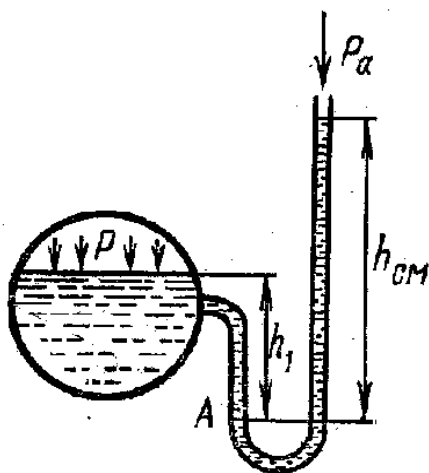
1.6-rasm. Suyuqlik manometri.
