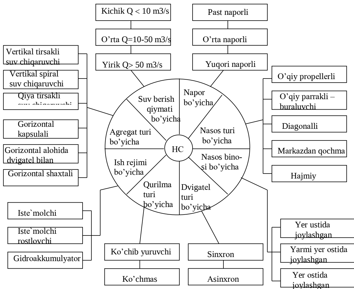
4.1-rasm. Nasos stansiyalarning sinfiy guruhlari.
