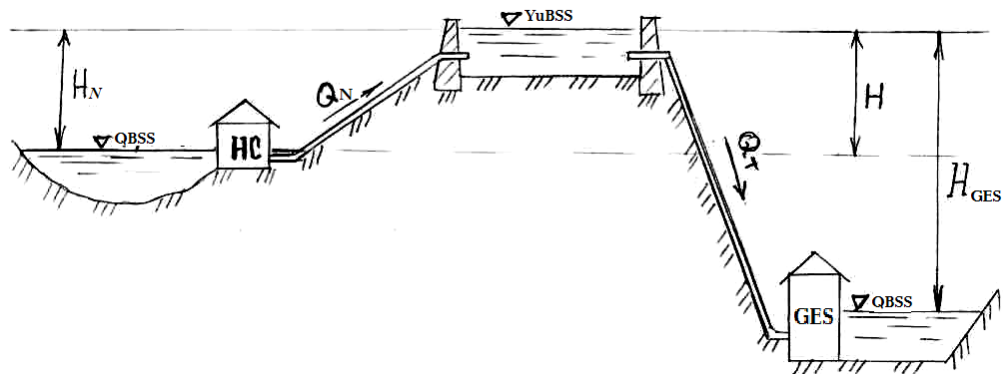
7.3-rasm. GES-NS sxemasi.
