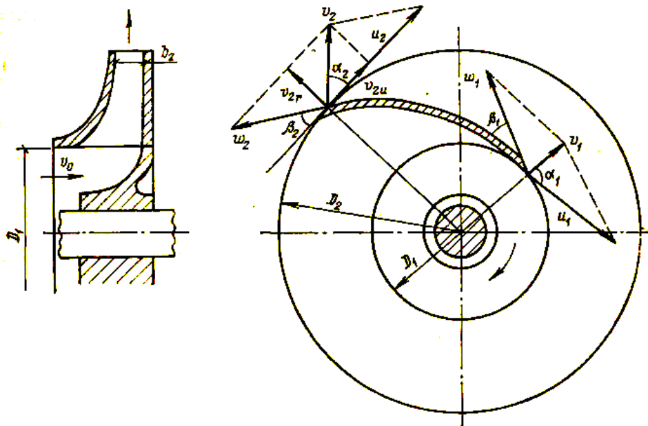
4.14-rasm. Suyuqlik oqimining markazdan qochma nasos ishchi g'ildiragidagi xarakati.
