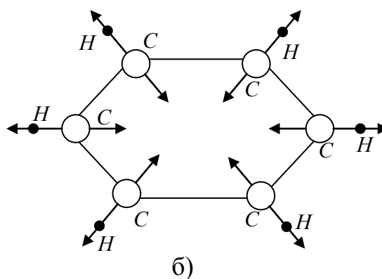
Расм 9. Бензол молекуласининг тўласимметрик тебраниши.
