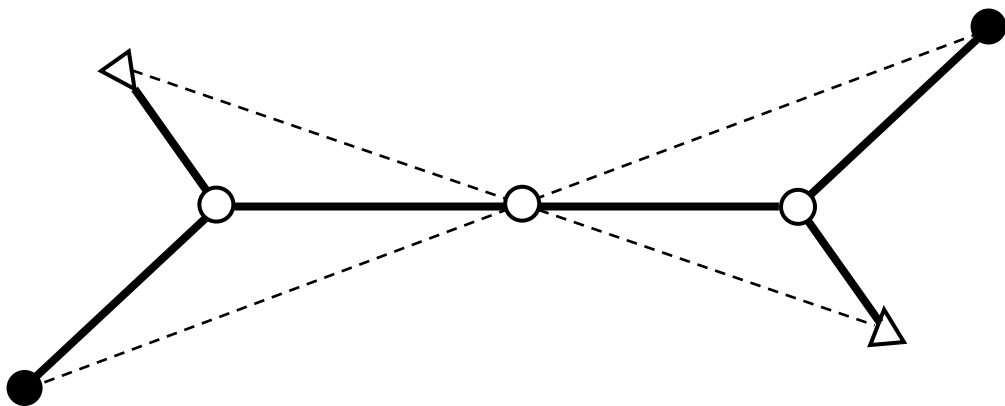
Расм 6. Симметрия марказига эга молекула.
