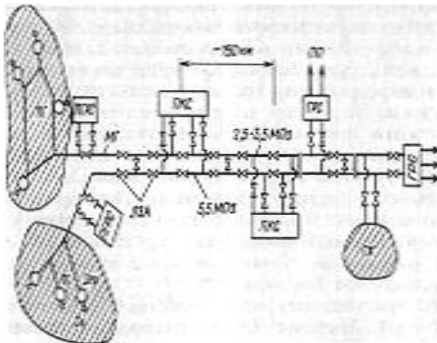
2.3. 1- расм: Газ етказувчи магистрал газ қувурининг асосий тасвири
