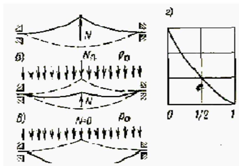
Мембрананинг нисбий эгилиши.
