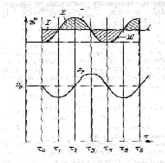
6.1.2.-расм. Ўз-ўзидан тенгланиш мумкин бўлмаганда астатик бошқарилиш тасвири
