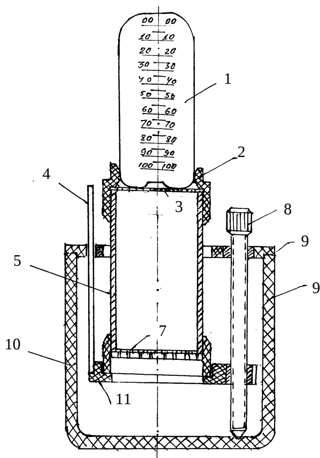
48–расм. Қумли грунтларнинг сизиш коэффицентини аниқлаш асбоби КФ–ООМ нинг схемаси: 1 – шишадан ясалган ўлчовли Мариотт баллони (ГП–32–06); 2 – грунт намунаси олинган (солинган) металдин ясалган цилиндр устига киргизилган қалпоқ (муфта); 3 – латундан ясалган тўр; 4 – босим градиентини ўлчаш учун махсус ўлчовли планка; 5 – қум солиш учун юзаси A=25 \text{ см}^2 бўлган металлдан ясалган цилиндр; 6 – металлдан ясалган цилиндрнинг остки қапқоғи, ичига латун тўр ўрнатилган; 7 – латундан ясалган тўр; 8 – махсус винт – грунт намунаси, керакли босим градиентини ўрнатиш учун хизмат қилади; 9 – телескопик мосламанинг устки қапқоғи; 10 – телескопик мосламанинг корпуси; 11 – грунт намунасини қўйиш учун мослама.
