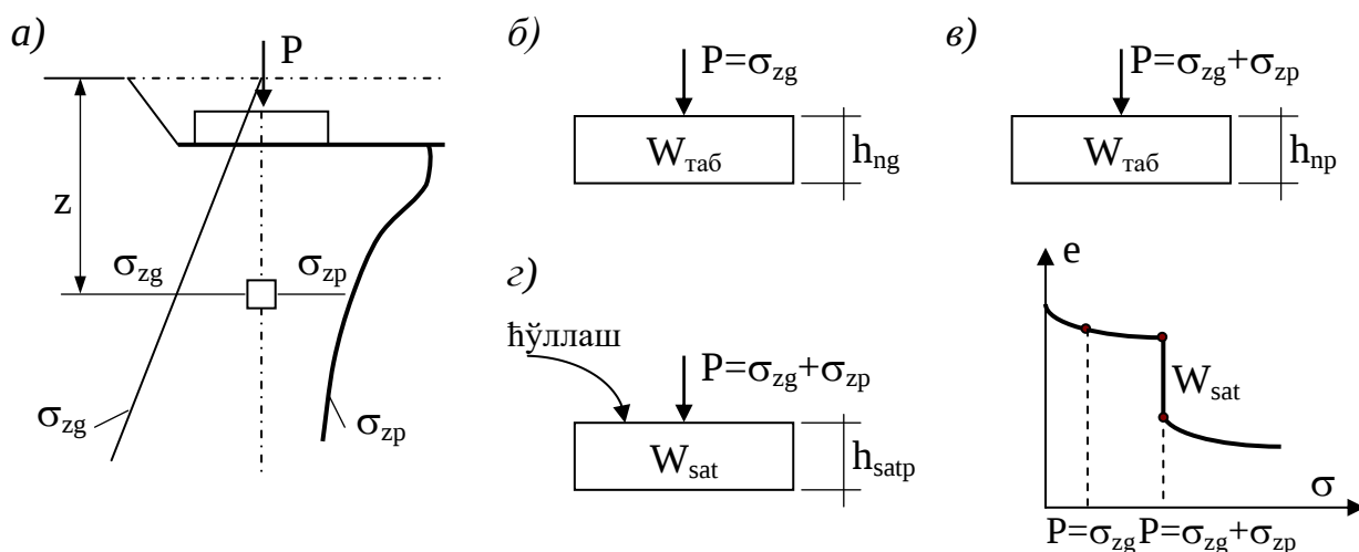
28-расм. \varepsilon_{sl} аниқлаш учун ҳисобий схемалар.
