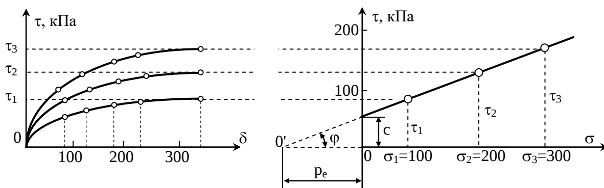
44–расм. Лойли грунтлар учун силжиш диаграммаси: а – силжитувчи кучланиш \tau билан горизонталь силжиш \delta орасидаги боғланиш графиги; б – чекли силжитувчи кучланиш \tau_{i,ч} билан нормаль сиқувчи кучланиш \sigma орасидаги боғланиш графиги.
