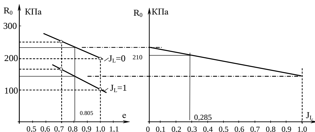
17 –расм. Лойли грунтнинг ҳисобий қаршилигини аниқлаш графиклари
