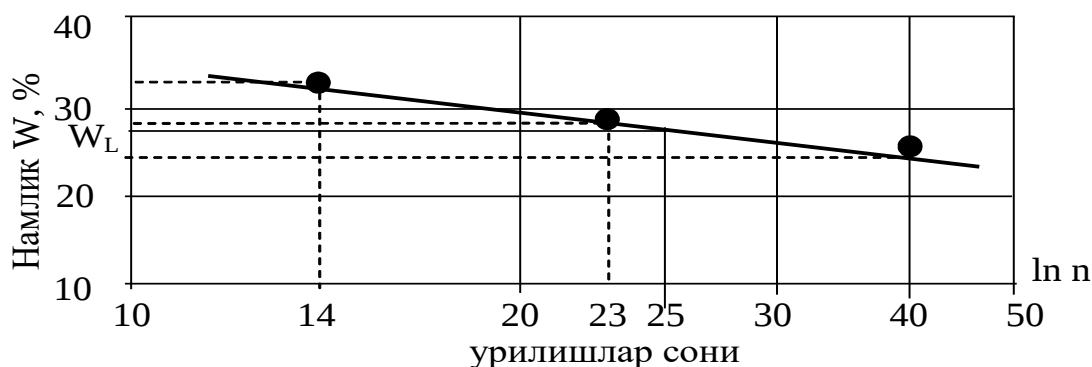
9-расм. "Оқувчанлик" эгри чизиғи (Казагранде бүйича)
