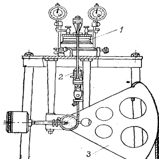
19-рasm. Компрессион курилманинг умумий кўриниши:
