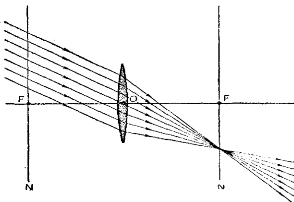
35- rasm. Linza va uning biror qo'shimcha optik o'qiga parallel bo'lgan nurlar dastasi
