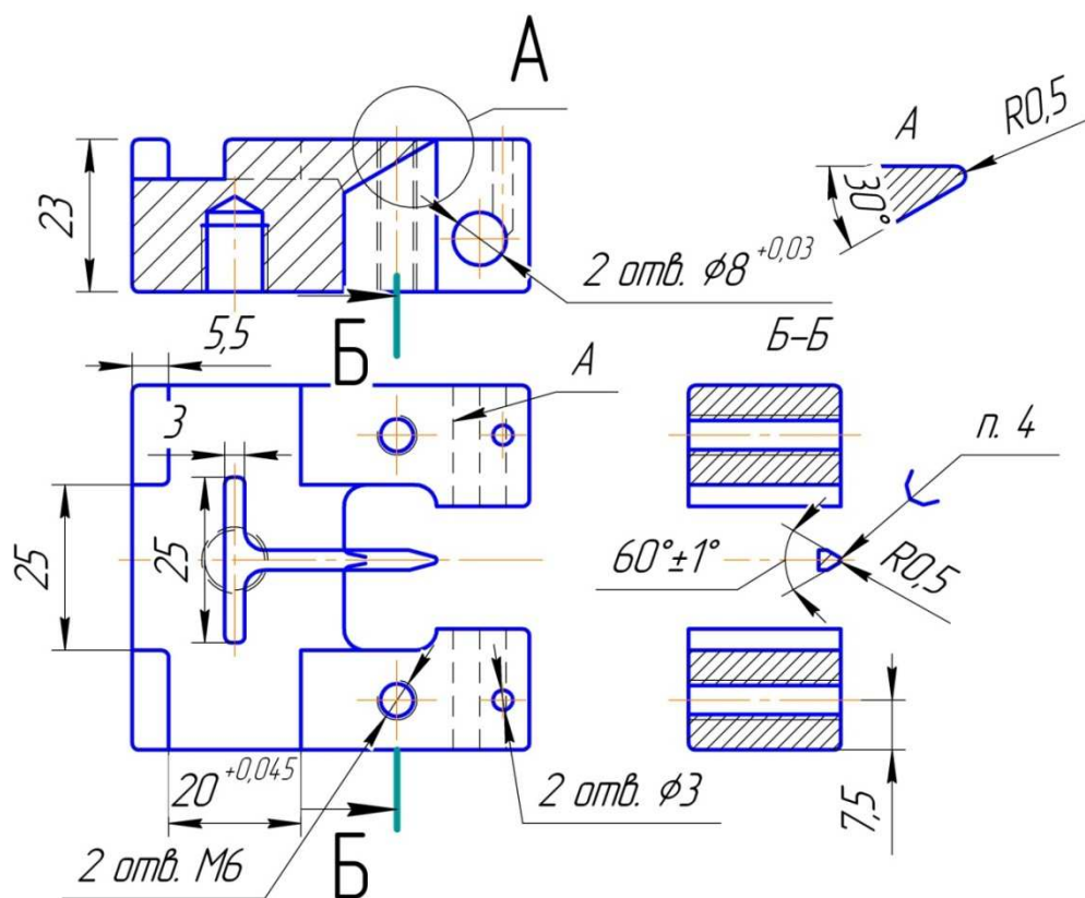
3.10-рasm. Пастки калодкани умумий кўриниши.
