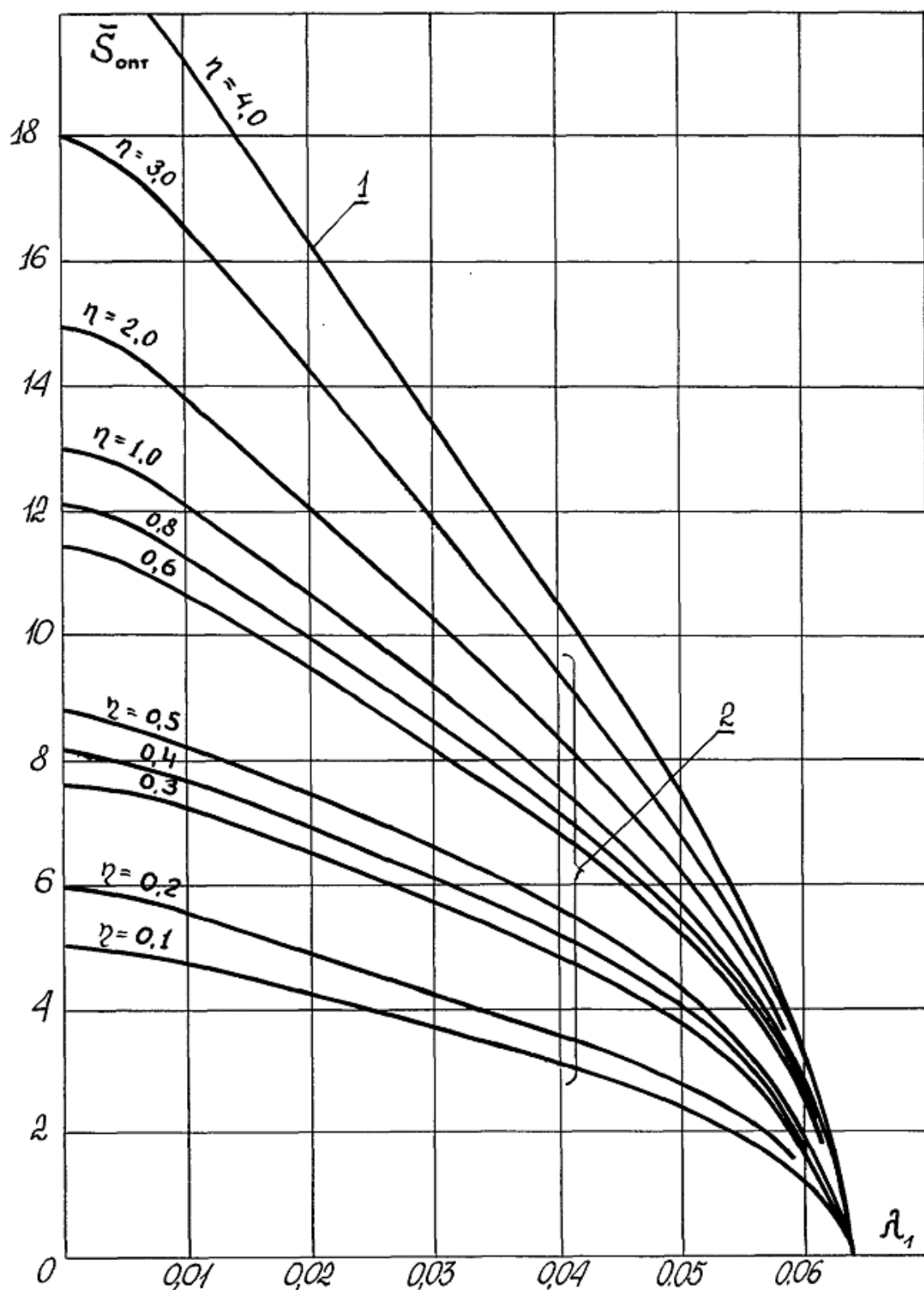
2.4-расм. \eta = \frac{\bar{a}}{b_0} нинг турли қийматларида лабиринт зичлагичлари оптимал параметри \bar{s}_{opt} нинг \lambda_1 коэффициентга боғлиқлиги. 1-эгри чизик \bar{s}_{opt} = f(\lambda_1) \bar{a} = \text{const} = 8\text{мм} ; 2-эгри чизиклар дастаси \bar{s}_{opt} = f(\lambda_1) \eta = (0.1 \div 4.0)b_0 да \bar{a} = \eta b_0 шароит учун.
