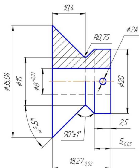
3.12-расм. 2-роликни умумий кўриниши.
