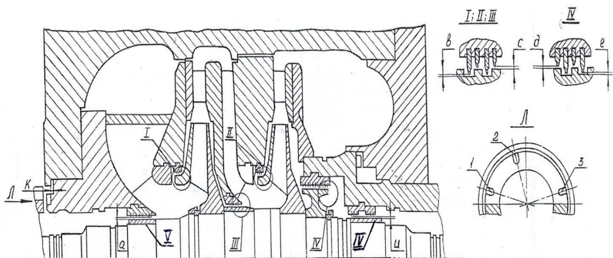
3.4-расм. 650-21-2 туридаги ЦБН лабиринт зичлагичлари.
