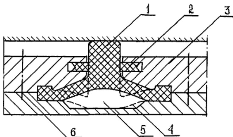
1.3-расм. 5-турдаги элементли ва 9-турдаги бир ёки икки манжетли деформатив-гидравлик бошқарилувчи зичловчи қурилма.
