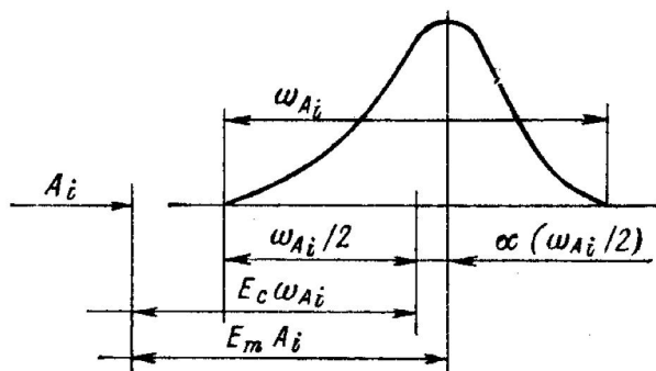
2.9-рasm. Ўлчамларнинг ёйилиш майдонининг ўртасига ω нисбатан тақсимланиш эгри чизиги
