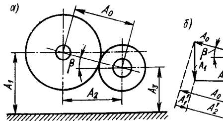
4.2-расм. Ясси ылчам занжирини чизи=пи ылчам
