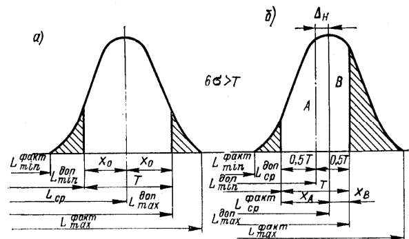
2.16-расм. Допуск майдонига нисбатан ёйилиш майдонининг симметрик (а) ва носимметрик (б) жойлашган яроқсиз деталлар
