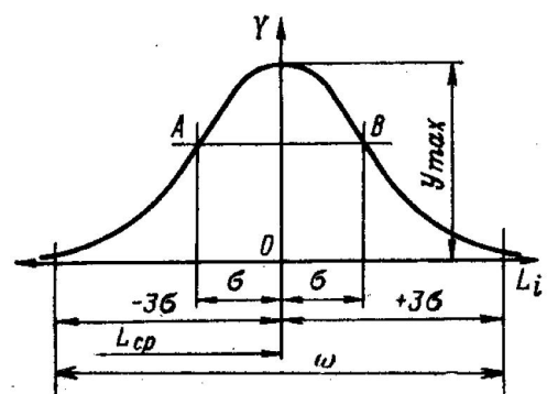
2.7-расм. Ўлчамларнинг нормал тақсимланишининг эгри чизиғи (Гаусс қонуни)
