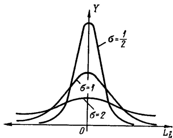
2.8-расм. Ўлчамларнинг нормал тақсимланиш эгри чизиги шаклига кўнча квадратик четга
