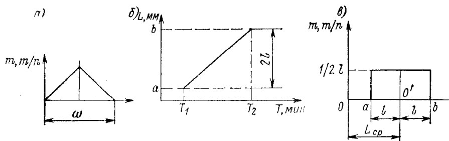
2.10-расм. Ишлов беришда хомакилар ўлчамларининг Симпсон қонуни (а) ва тенг эҳтимолли қонуни (б, в) бўйича тақсимланиши
