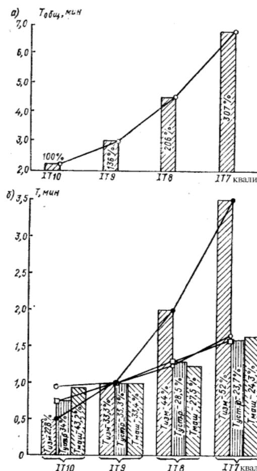
7.2-расм. Ишлов бериш иш шажмининг талаб =илинган ани=ликка бо\ли=лиги:
