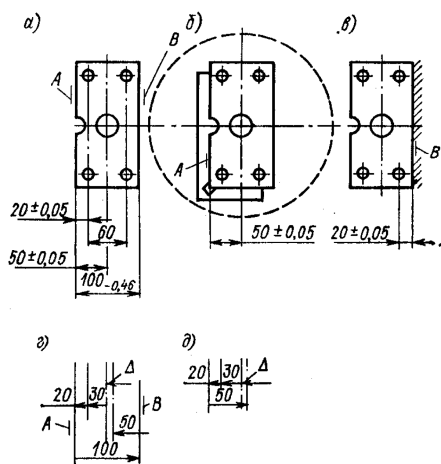
5.8-расм. Пармалаш ва ййниб кенгайтиришда
