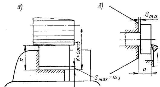
2.14-рasm. Фрезалашда (а) ва токарлик ишлов беришда (б) маҳкамлаш хатолиги \omega_{махк} = S_{махк}
