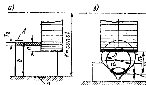
2.13-расм Базалаш хатолиги \omega_\Delta * \omega_\delta нинг келиб чиқиши
