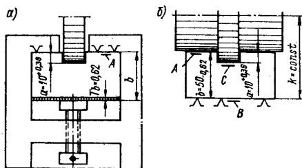
Расм 5.7. Конструкторлик база билан мос тушган технологик А базага
