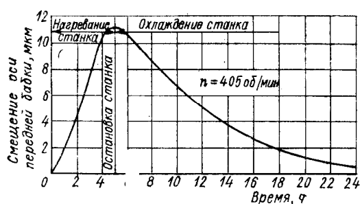
2.4-расм. Токарлик дастгоҳининг марказларида ишлов беришда олди бабканинг қизиши натижасида унинг йўналишнинг горизонтал йўналиш бўйича силжиши
