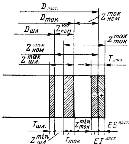
Расм 6.1. Валга ййниш ва жилвирлаш ор=али ишлов беришда =ййимларнинг ва допускларнинг жойлашиш схемаси
