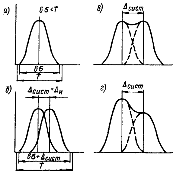
2.11-расм. Хомакиларнинг бир нечта партиясига дастгошни =айта созлаш билан ишлов беришда \Delta_{\text{сист}} таъсири натижасида тасодикий
