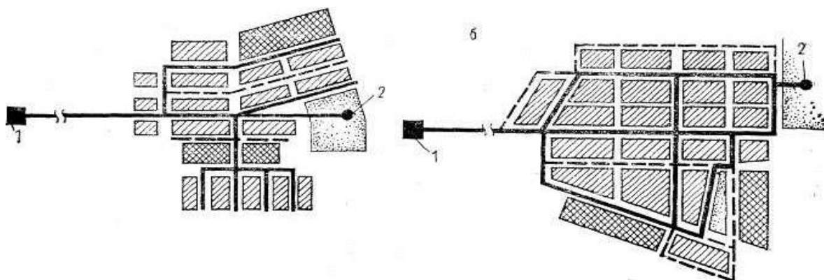
2.2 – расм. Сув қузури тармоғи
