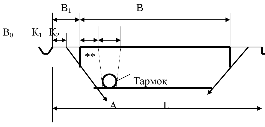
2.7–рasm. Ер ости муҳандислик тармоқларини махсус техник ораликда жойлаштиришнинг ҳисоблаш усули.
