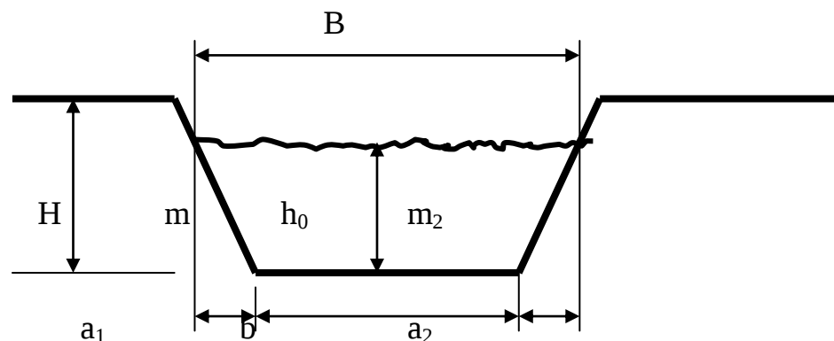
2.15- расм. Трапециякўринишидагиариккўндалангкесиминингюзаси.
