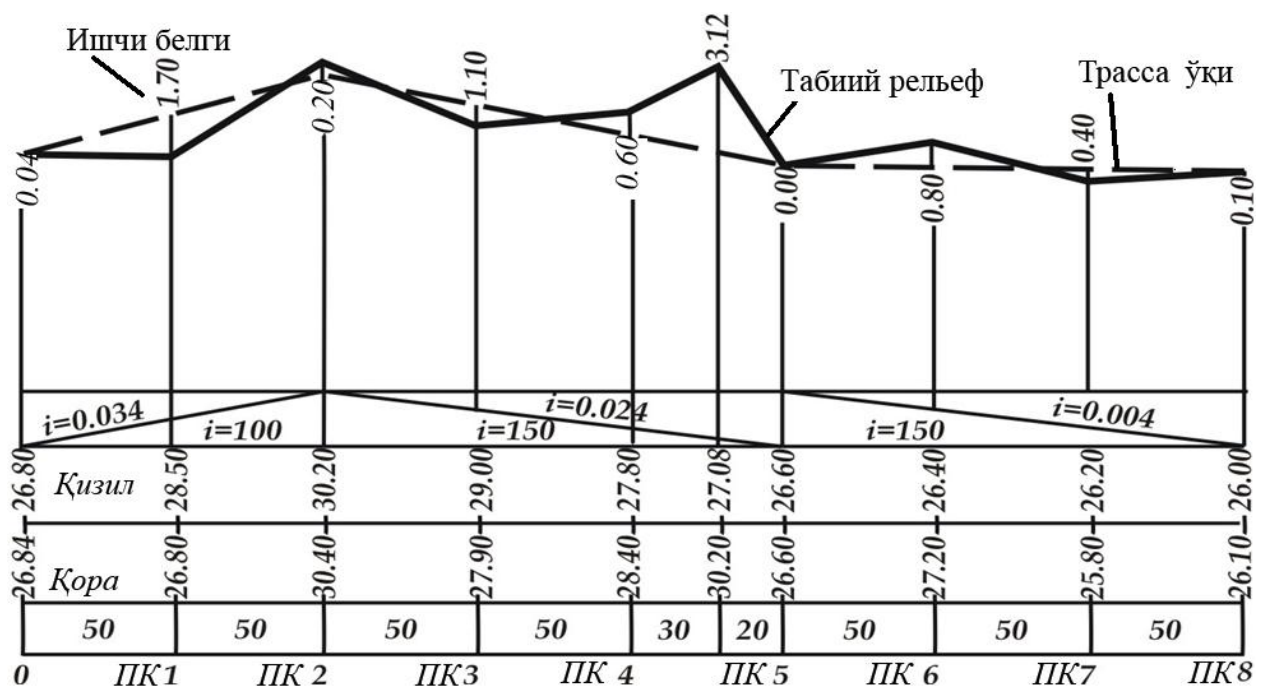
1.1-расм. Лойиҳавий ва ишчи белгилари кўрсатилган, лойиҳавий чизиқлар ўтказилган вертикал режа профили.
