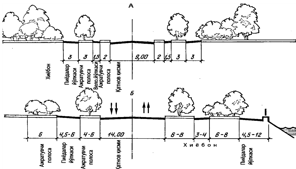
3.11- расм. Турар-жой кўчаларининг (А) ва қирғок бўйи кўчаларининг (Б) кўндаланг кесими.
