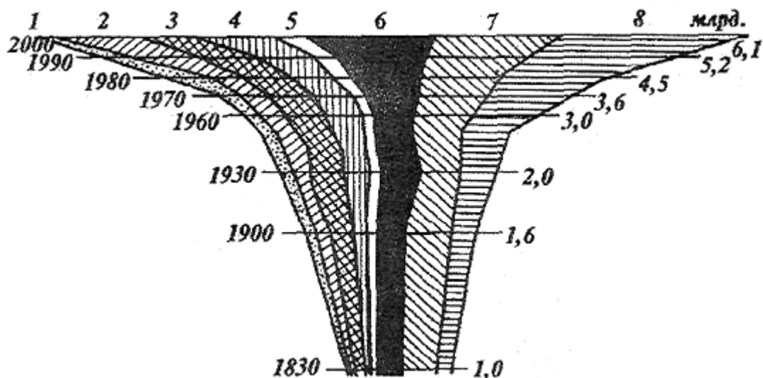
4-расм. Демографик портлаш Дунё регионлари хиссаси: 1-Шимолий Америка; 2- Лотин Америкаси; 3- Австралия ва Океания; 4-Африка; 5-Россия ва МДХ; 6-Ҳиндистон; 7-Хитой; 8- Осиёнинг қолган қисми (1)
