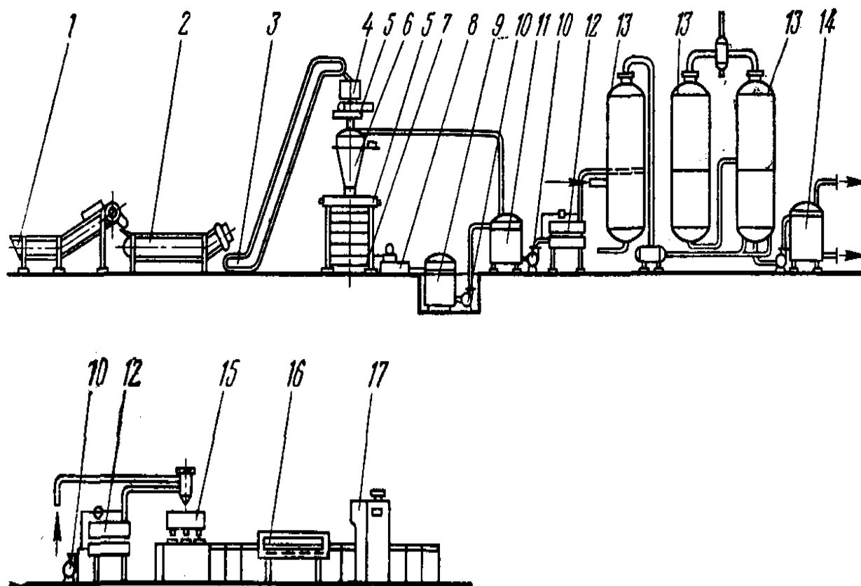
6- Расм. Қуюлтирилган тоmat шарбати ишлаб чиқариш схемаси
