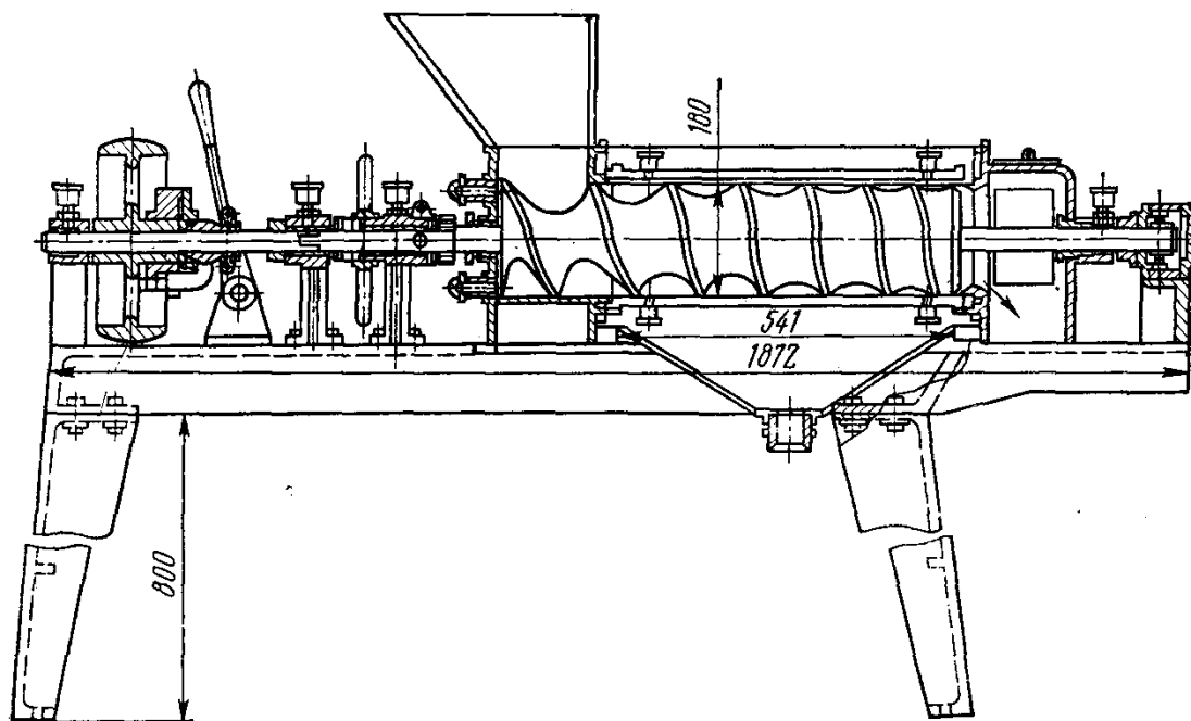
3-расм. Шарбат сиқиш. Экстрактор схемаси
