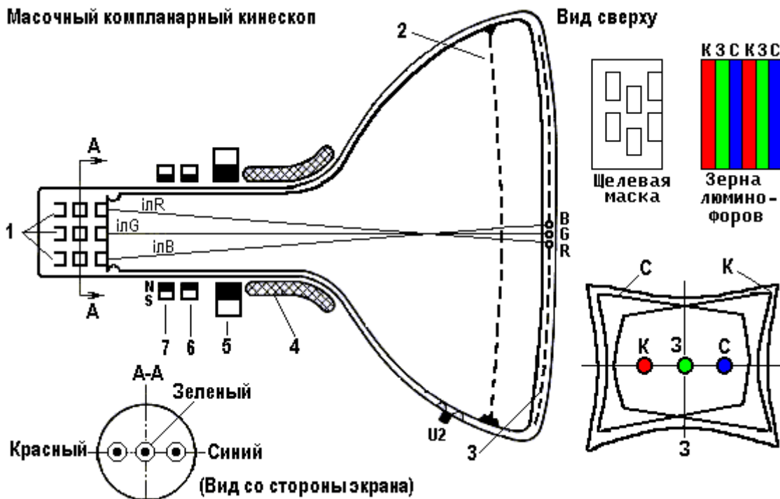
Рис.8.4. Конструкция компланарного кинескопа
