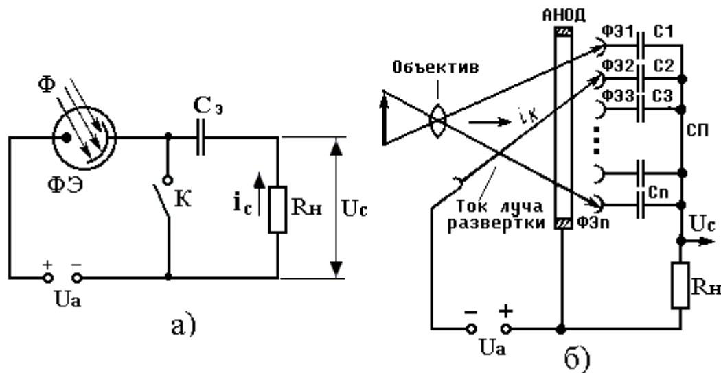
Рис. 7.3. Принцип накопления световой энергии: а - эквивалентная схема; б – модуль ТВ системы с накоплением
