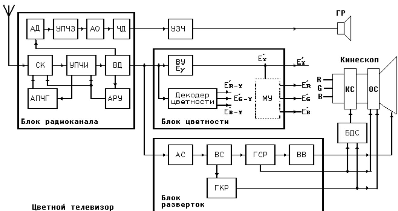
Рис.13.2. Обобщенная структурная схема цветного телевизора.
