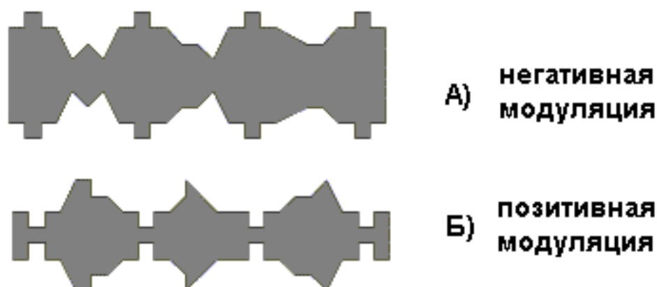
Рис.12.5. Вид амплитудно-модулированных сигналов изображения
