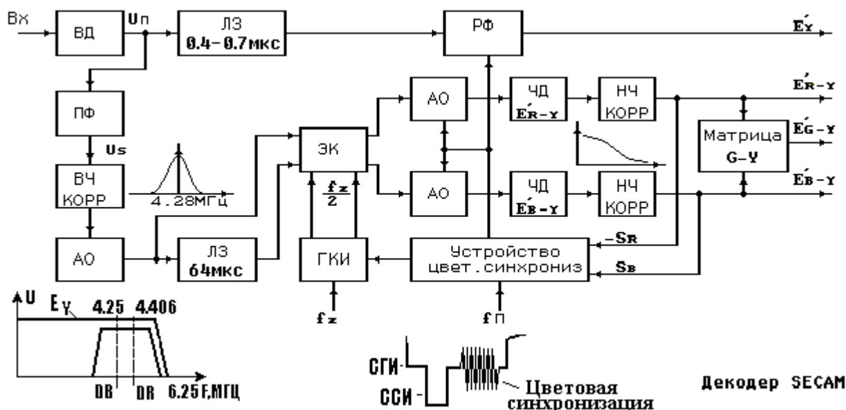
Рис.6.5. Обобщенная структурная схема декодера системы SECAM
