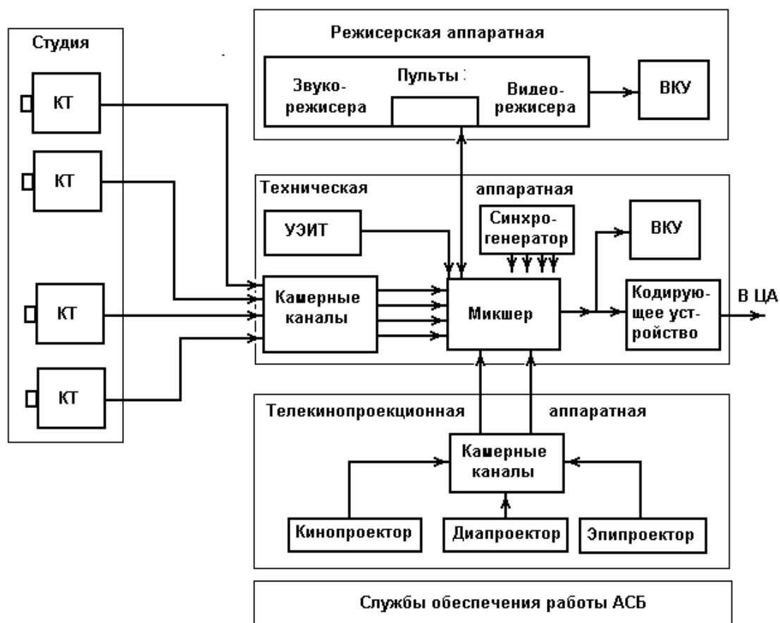
Рис.12. 2 Обобщенная структурная схема АСБ
