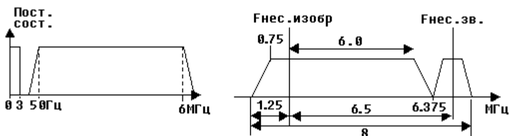
Рис.12.4. Номинальные АЧХ НЧ ТВ сигнала боковых полос радиопередатчика
