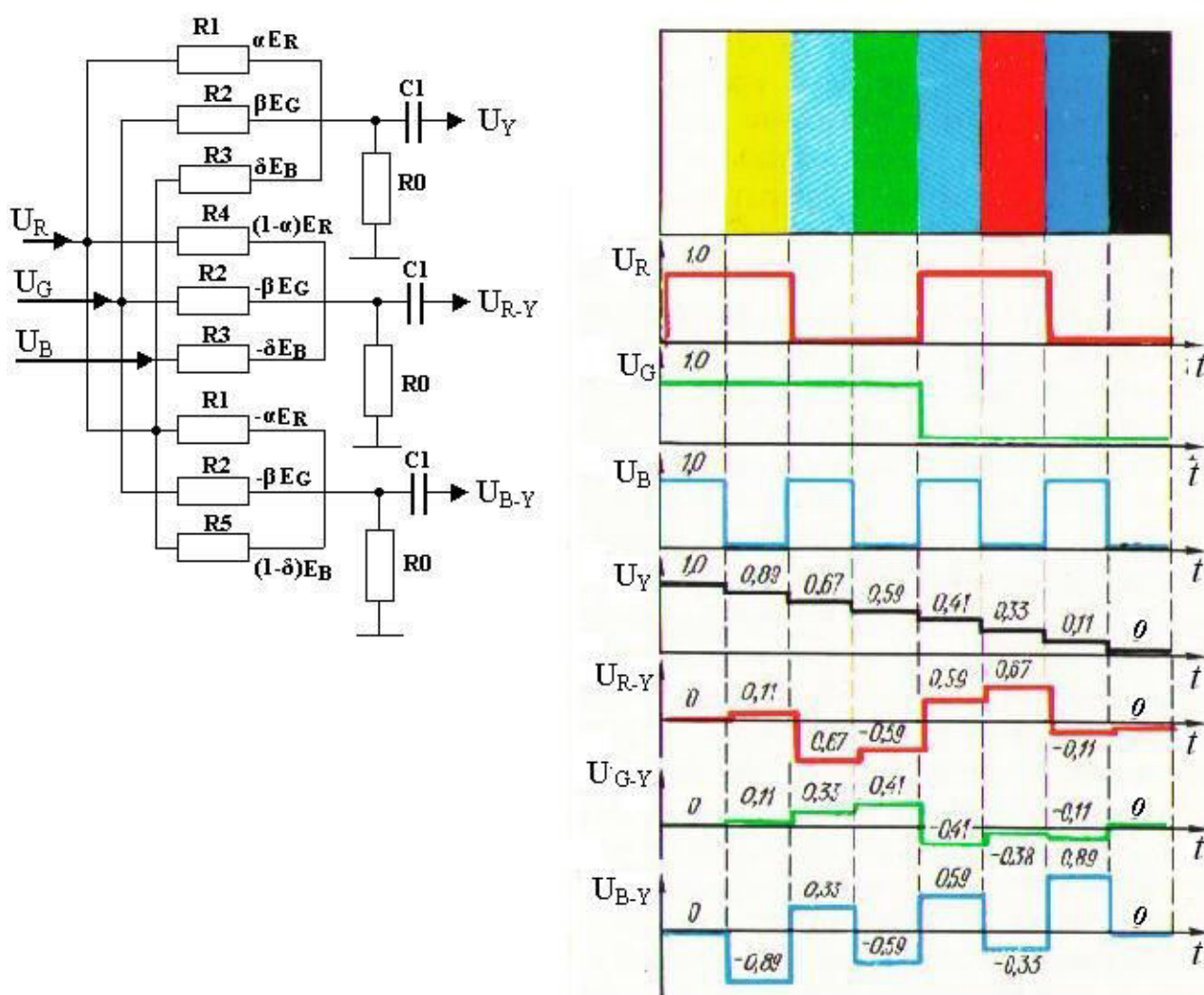
Рис. 5.6. Обобщенная структурная схема кодирующей матрицы
