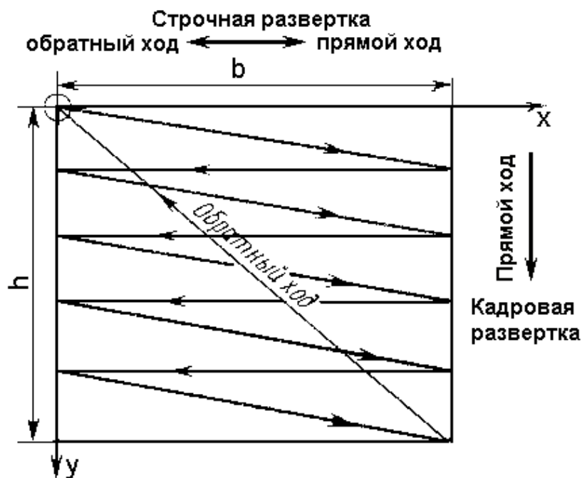
Рис.1.8. Линейно-строчная развертка
