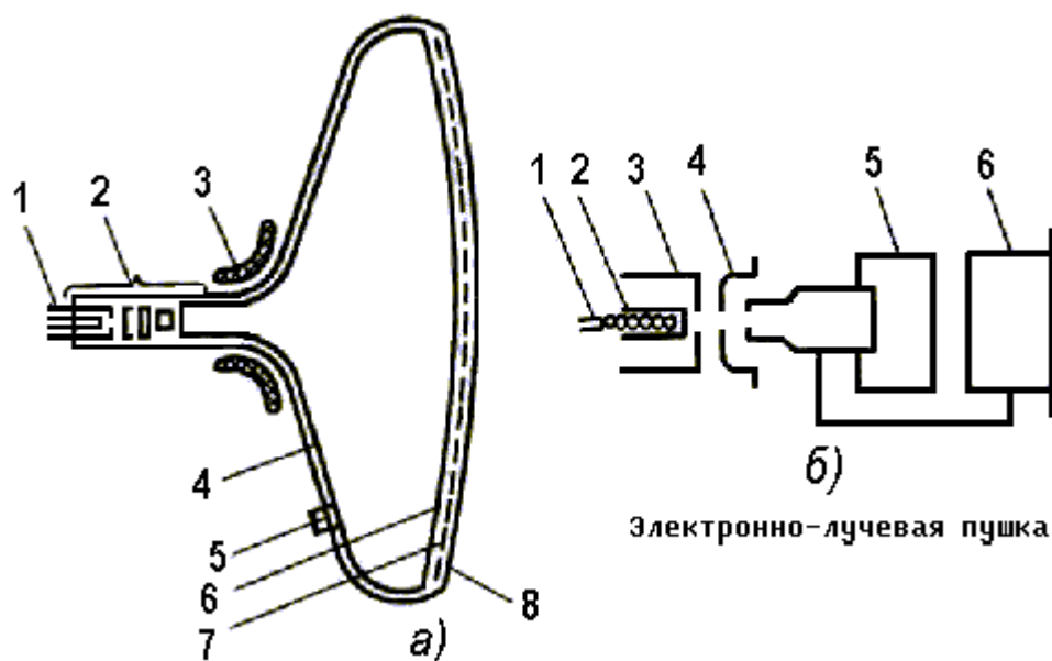
Рис.8.1. Устройство черно-белого кинескопа
