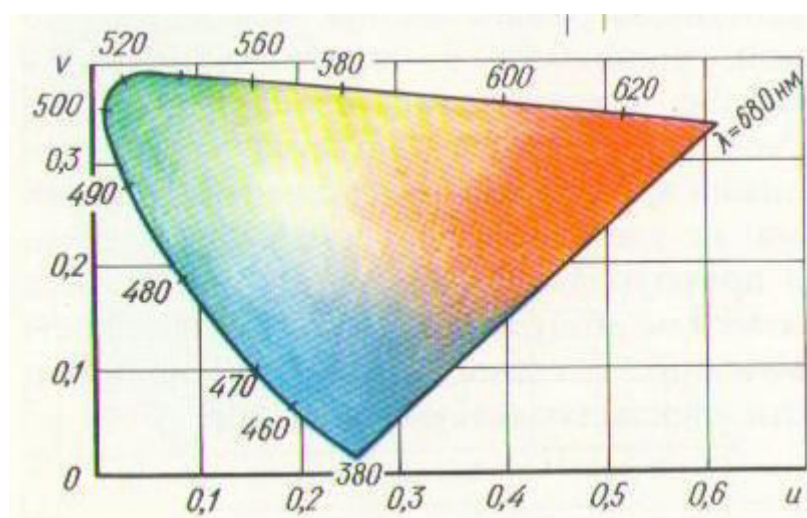
Рис.5.1. Система RGB
