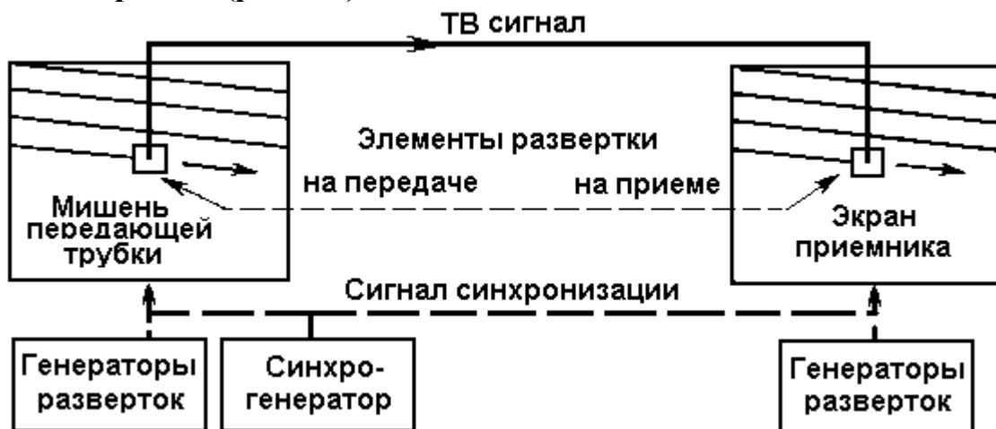
Рис.1.9. Синхронизация разверток передающей и приемной стороны
