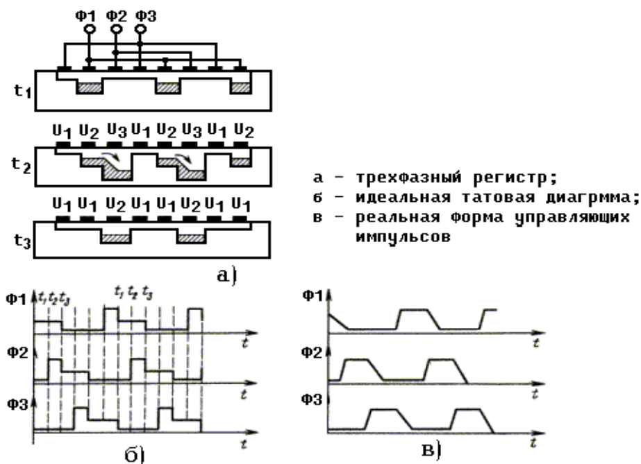
Рис. 7.8. Принцип перемещения зарядовых пакетов в сдвиговом регистре ПЗС
