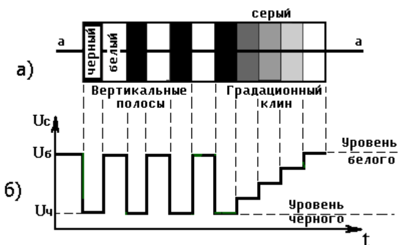
Рис.4.1. Формирование видеосигнала
