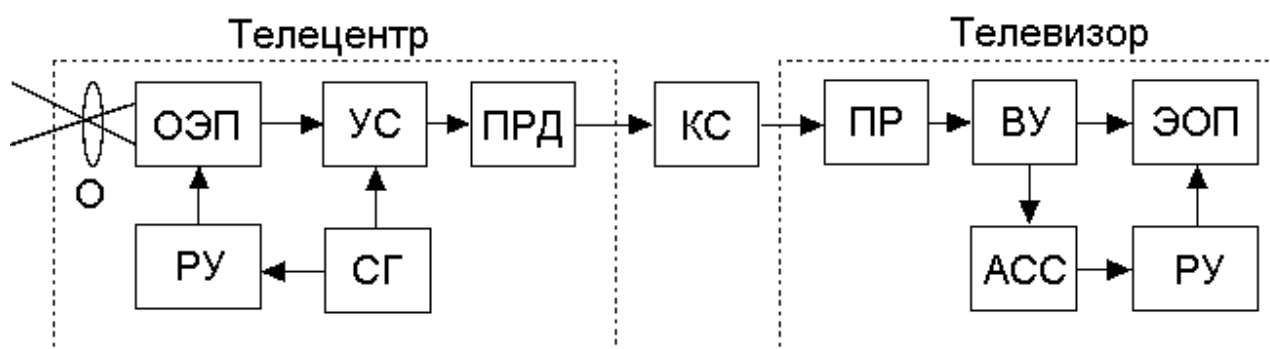
Рис.1.10. Обобщенная структурная схема ТВ системы
