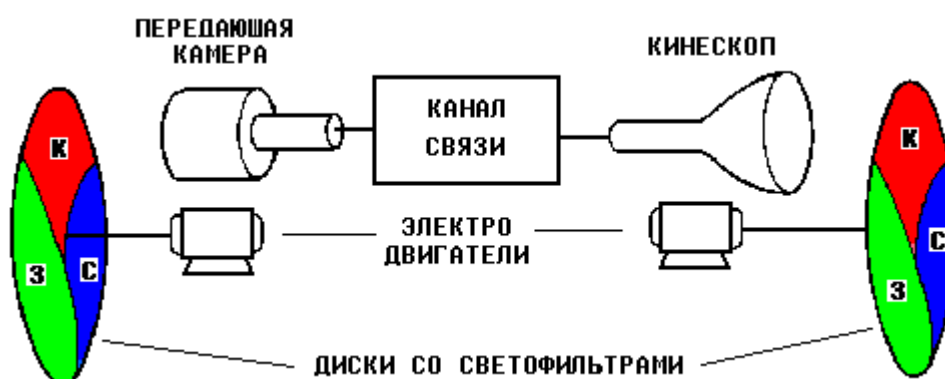
Рис. 5.3. Схема последовательной система ЦТВ
