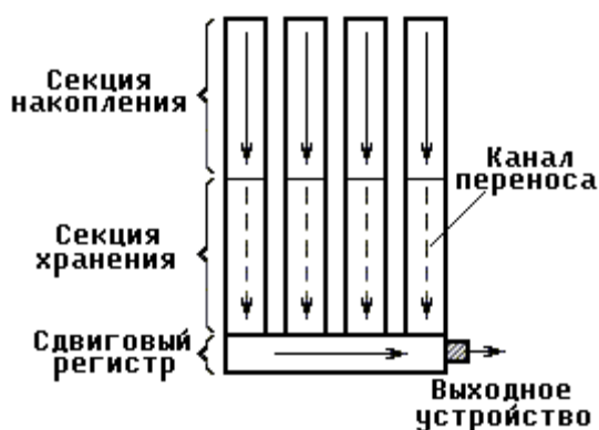
Рис.7.9. Способ организации покадрового считывания
