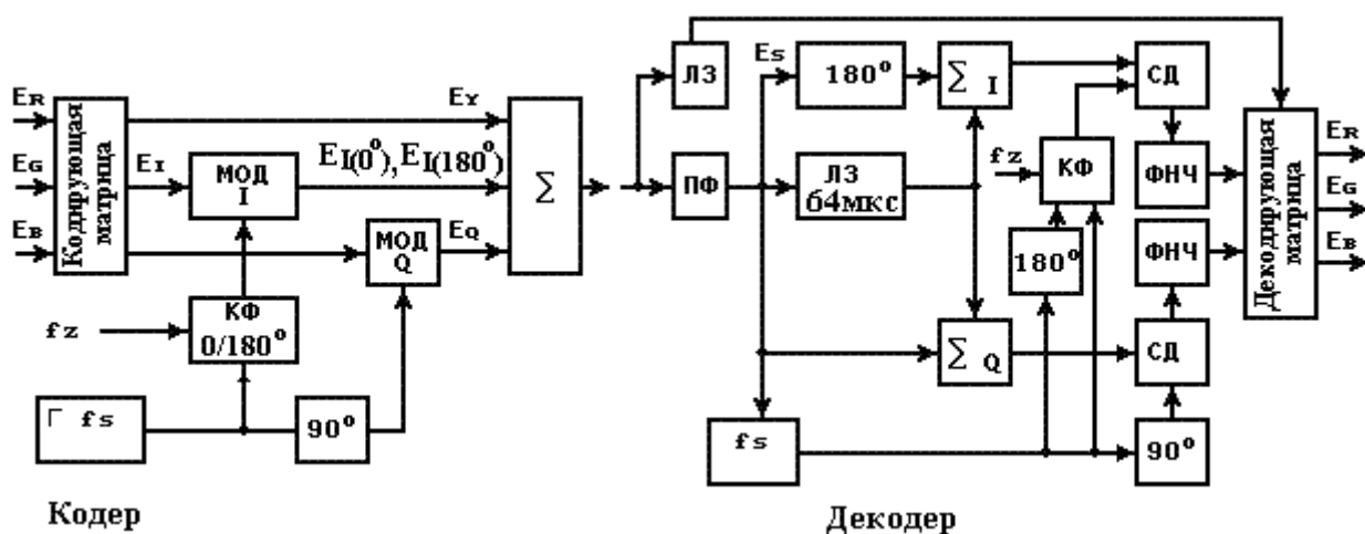
Рис.6.8. Обобщенная структурная схема системы PAL
