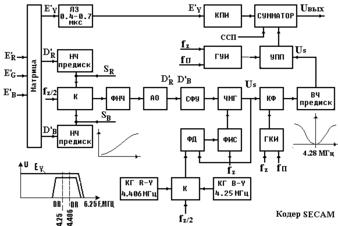
Рис.6.4. Обобщенная структурная схема кодера системы SECAM
