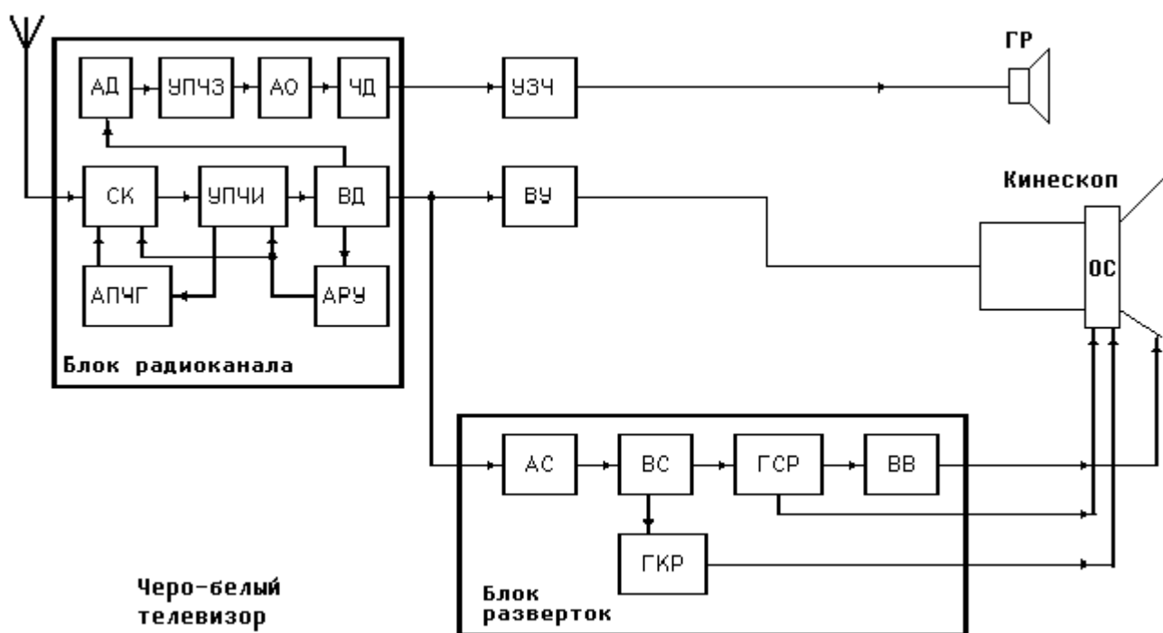
Рис.13.1 Структурная схема черно-белого телевизора
