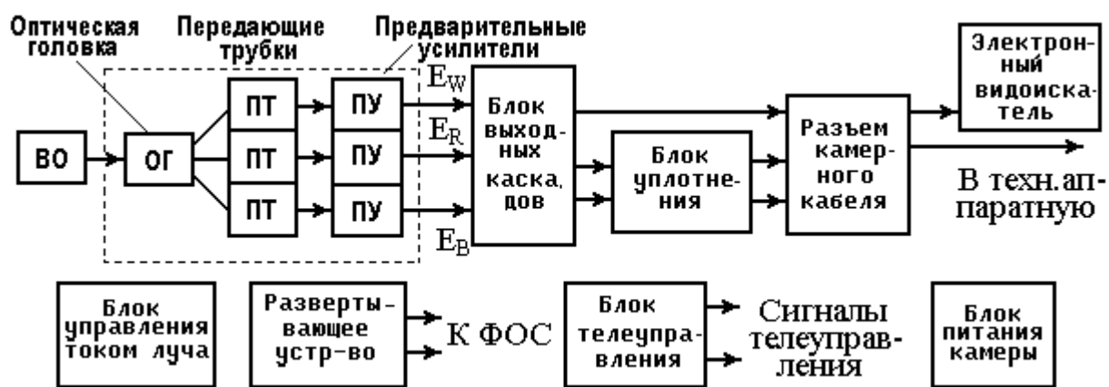
Рис.12.2. Обобщенная структурная схема 3-х трубчатой цветной передающей камеры
