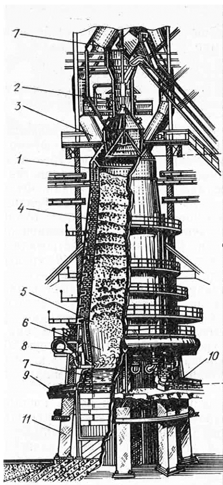
1- расм. Домна печининг тузилиш схемаси: 1-колошник; 2-юклаш аппарати; 3-трубалар; 4-шахта; 5-распар; 6-заплечик; 7-ўтхона; 8-фурма; 9-чўян чиқиш нови; 10-шлак чиқиш нови; 11-темир устун.
