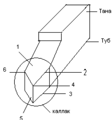
31-расм. Кескичнинг асосий қисми ва элементлари.
