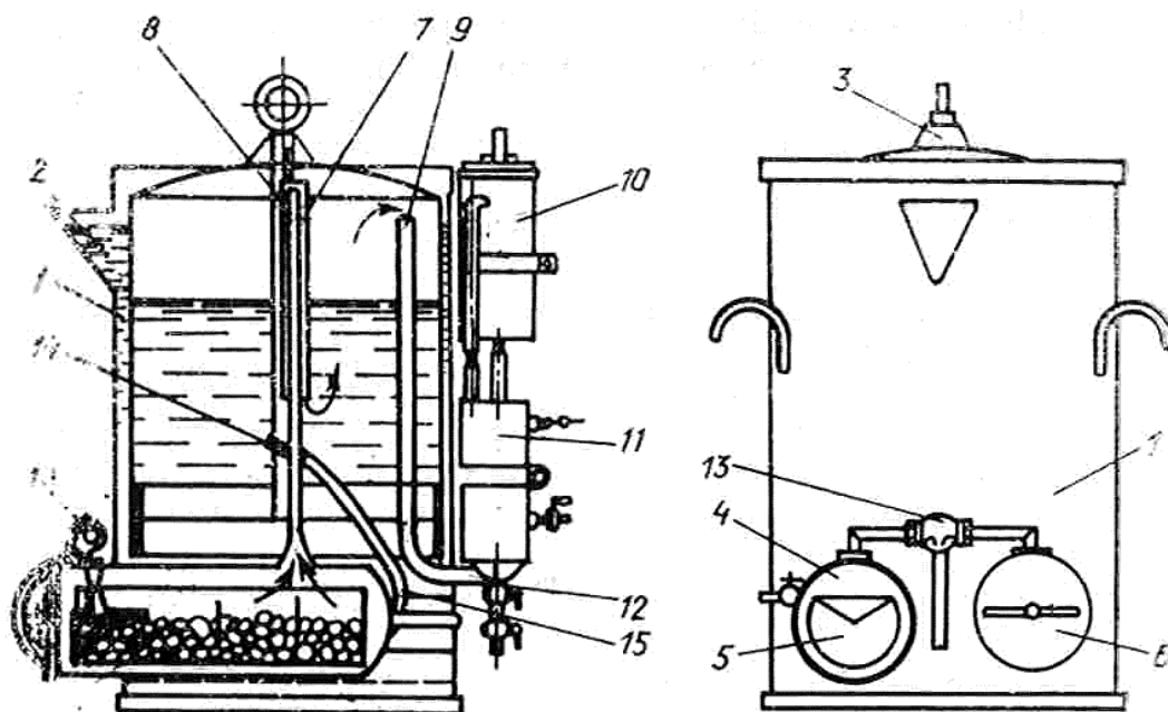
9-расм. Карбидга сув таъсир эттириш принципида ишловчи ацетилен генераторининг схемаси.
