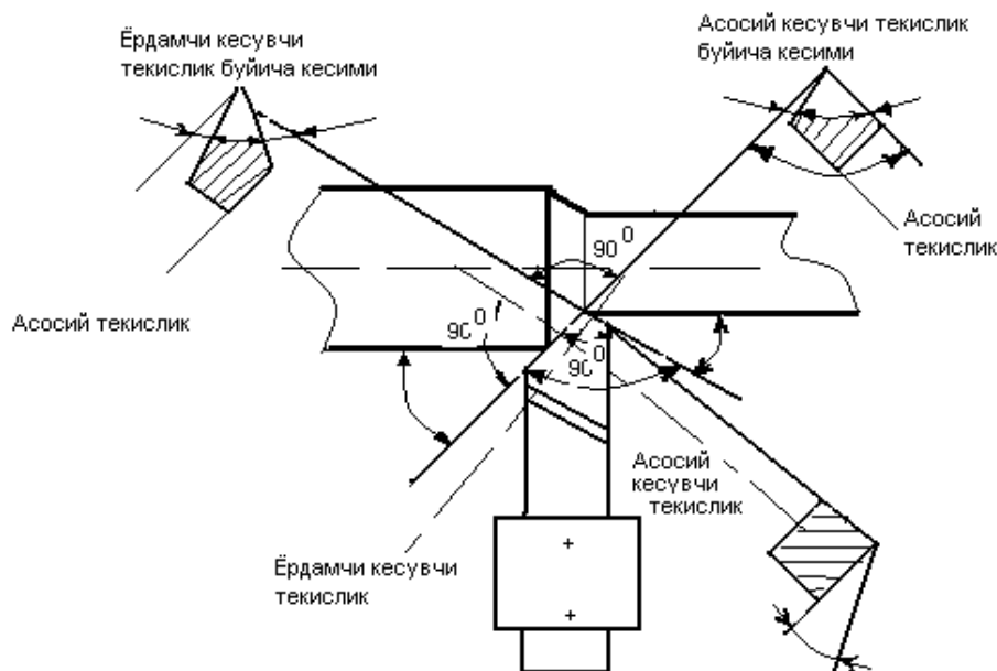
33-расм. Токарлик кескич кесувчи қисми геометриясининг асосий элементлари.
