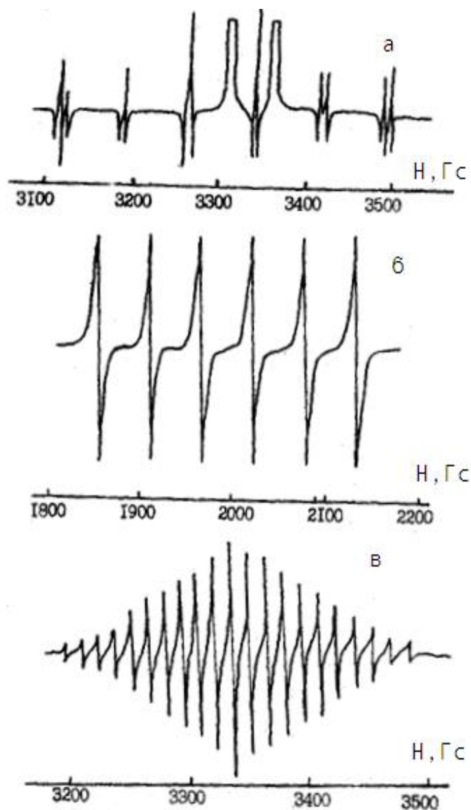
23-расм. n\text{-Si}\langle Mn \rangle даги Mn^+ (а), Mn^0 (б) ва (Mn^0)_4 (в) марказларининг ЭПР спектрлари. T = 4.2\text{ К}
