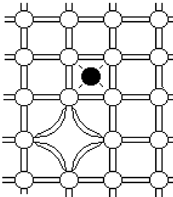
11, д-расм. Френкель нуқсони: вакансия ва тугундан чиққан хусусий атом жуфти
