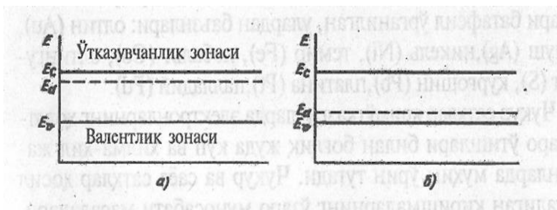
19-расм. Яримўтказгичнинг энергетик диаграммаси: а) донор киришмали яримўтказгич; б) акцептор киришмали яримўтказгич.
