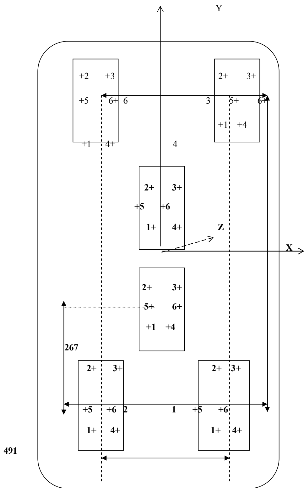
5-rasm. Fotoapparat maxkamlangan oynalarda va kamera kordinata sistemasida ob'yektivlarning hamda reper krestlarning joylashish sxemasi.
