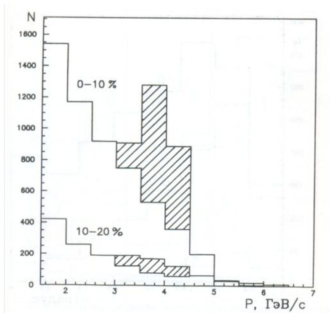
14-rasm. Proton-propan to'qnashuvlardagi protonlarning impuls taqsimoti (impul'sni 0-10% va 10-20% aniqlikda o'lchash uchun)
