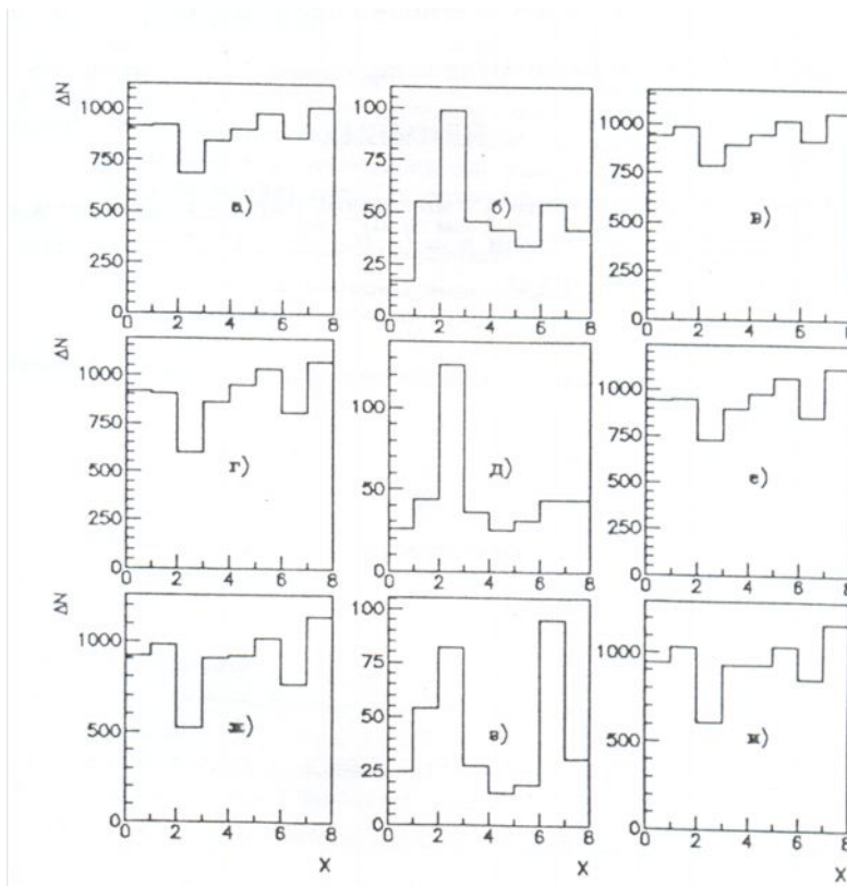
8-rasm. "7"-tipdagi zarrachalarning azimutal taqsimoti a,г,ж-impulslari o'lchangan protonlar); "47"-tipdagi (б,д,з-impulslari o'lchanmagan protonlar); va yig'indi (7+47,в,с,и) – qutb burchagining har xil 40^\circ < \theta < 50^\circ (a,б,в), 50^\circ < \theta < 65^\circ (г,д,е) va 65^\circ < \theta < 80^\circ (ж,з,и). Absissa o'qi bo'yicha X o'zgaruvchi
