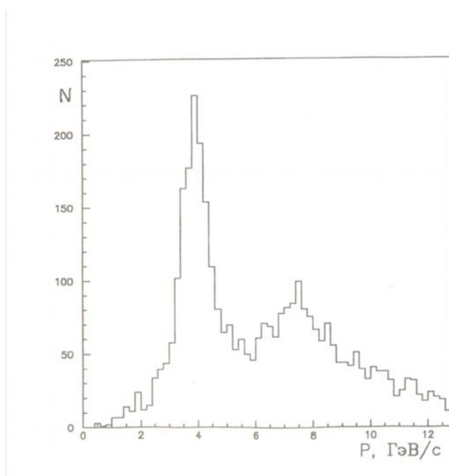
9-rasm. 4.2 A*GeV/c impulsli uglerod-propan o'zarota'sirlashuvlardagi protonlarning 0-1 gradus burchak ichida impuls bo'yicha taqsimoti (laboratoriya sistemi).
