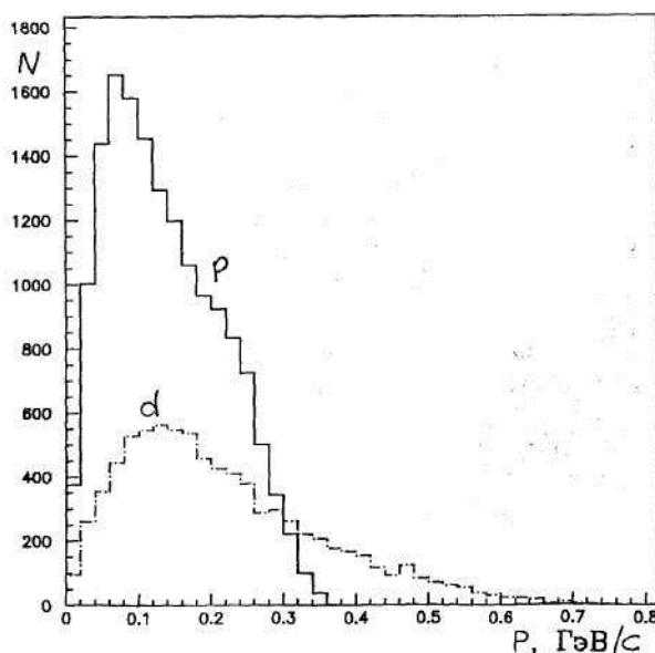
19-rasm. Uglarod-proopan o'zaro ta'sirlashuvlarda hosil bo'lgan rotonlar va deytronlarning ko'ndalang impuls bo'yicha taqsimoti.
