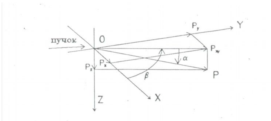
4-rasm. 500 litr hajmli propanli pufakchali kameraning koordinata sistemasi.
