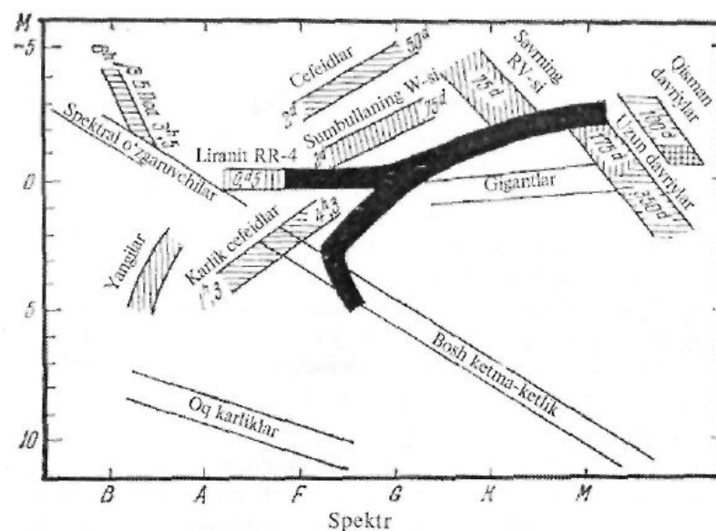
3.17-rasm. Har xil turdagi pulsatsiyalanuvchi yulduzlarni spektr — yorqinlik diagrammasida joylashishi.
