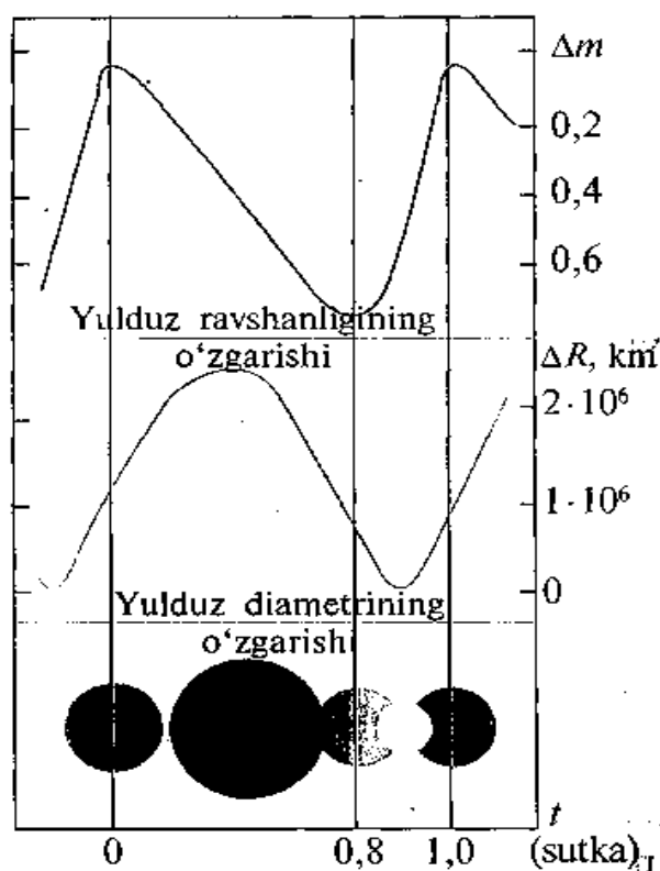
118- rasm. Sefeid (Sefeyning \delta tipidagi yulduz)larning ravshanligi ( \Delta m ) va radiusining o'zgarish ( \Delta R ) egriliklari.
