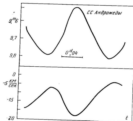
Кривые блеска (сверху) и изменения лучевой скорости звезды SS Андромеды. Кривые являются почти зеркальным отображением одна другой
