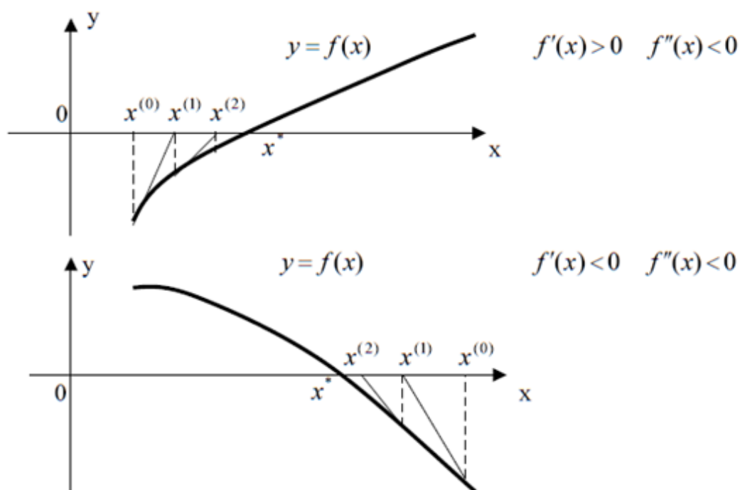
2.4-rasm. f(x) funksiyaning har xil holatlari uchun Nyuton usulining geometrik interpretatsiyasi.
