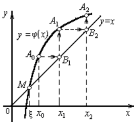
2.6-rasm. Uzoqlashuvchi iteratsion jarayon.
