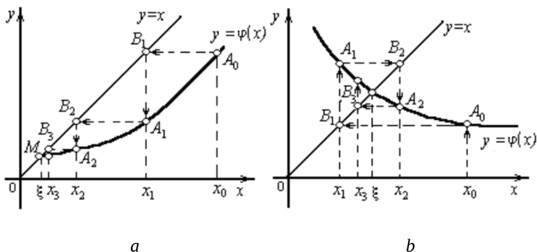
2.5-rasm. Yaqinlashuvchi iteratsion jarayonlar.
