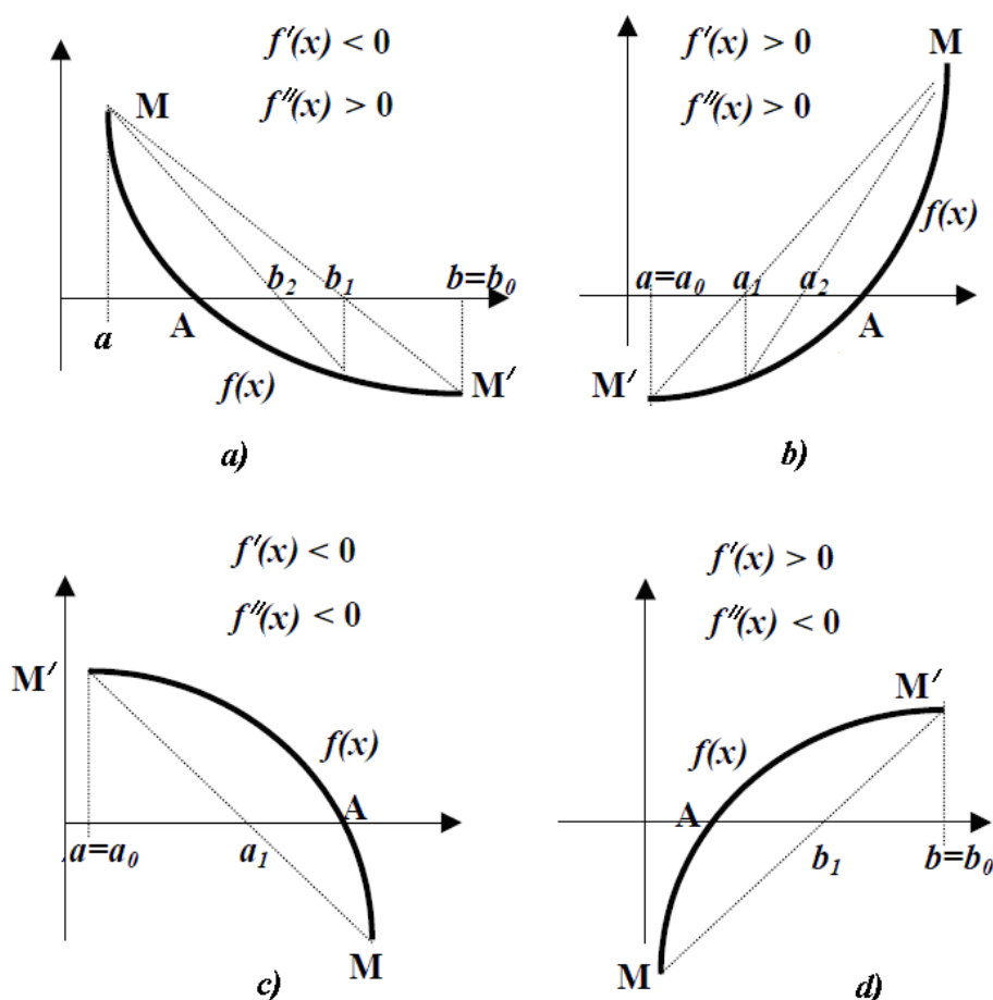
2.2-rasm. Proporsional bo'laklar usuli (vatarlar usuli)ning har xil hollari uchun sxemalar.
