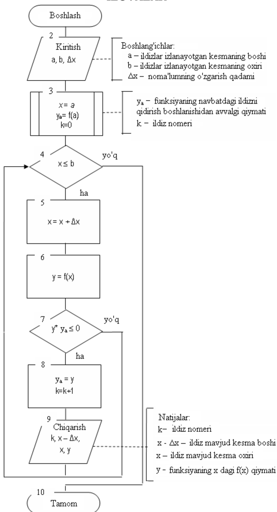
I.1-rasm. Tenglamaning haqiqiy ildizlarini ajratishning blok-sxemasi.
