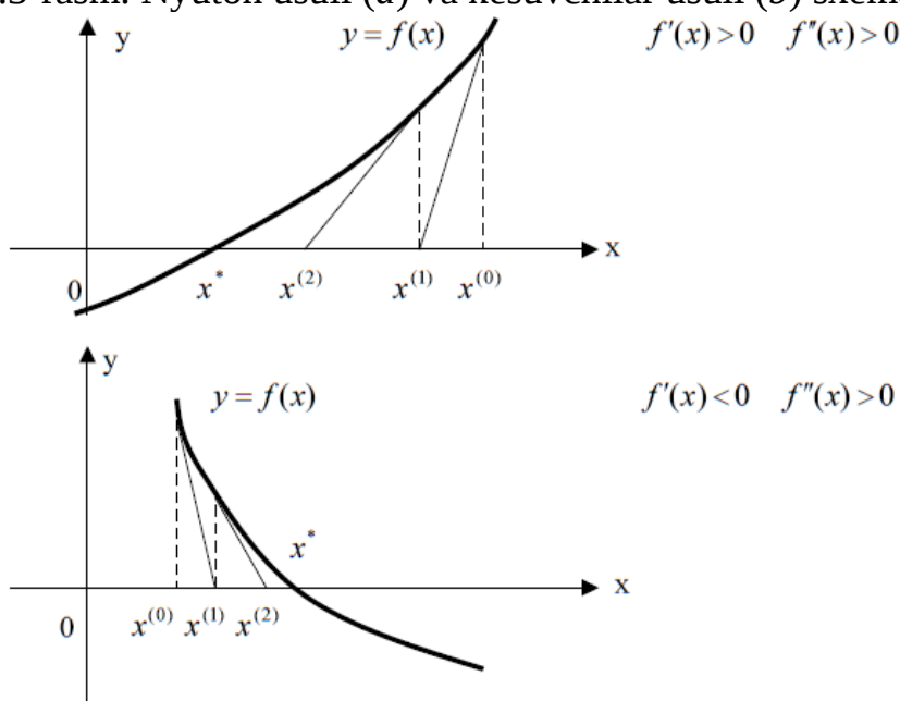
2.3-rasm. Nyuton usuli (a) va kesuvchilar usuli (b) sxemasi.
