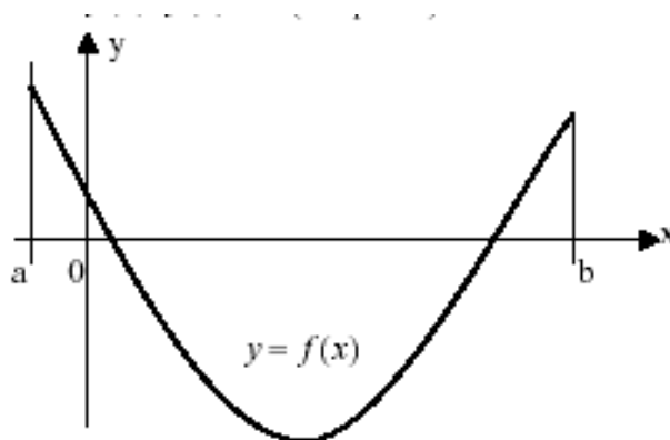
1.2-rasm. Tenglamaning kesmada bir nechta ildizlar yotishi mumkin bo'lgan hol.
