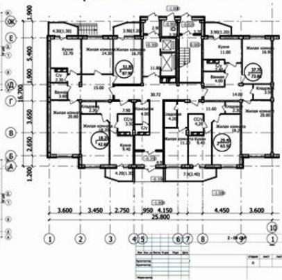
Фрагмент плана этажа М 1:100
