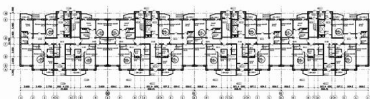
План первого этажа М 1:200
