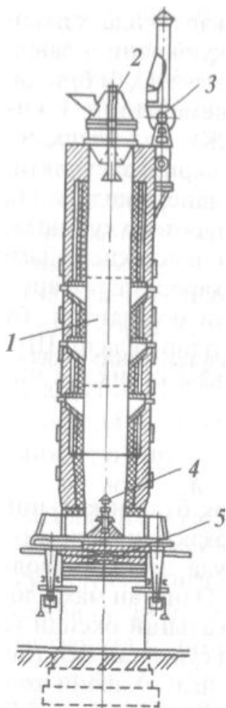
1-расм. Шахтали ўчоқ: 1— шахта; 2— хом ашё солади-ган қурилма; 3— ҳаво сўргич; 4— гребень; 5— пишиган оҳакни олиш.
