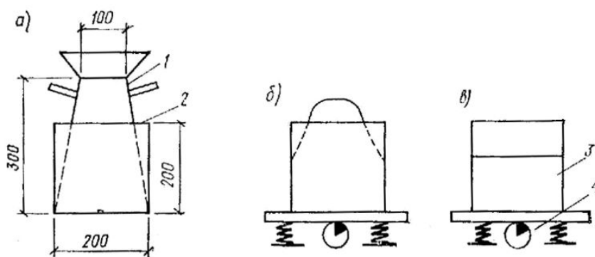
4-расм. Қоришма қаттиқлигини аниқлашнинг оддий усули. а) ускунанинг умумий кўриниши; б) – титратгунга қадар қоришма; в) титратгандан кейинги қоришма; 1-конус; 2-қолип; 3-бетон қоришмаси; 4-титратгич.
