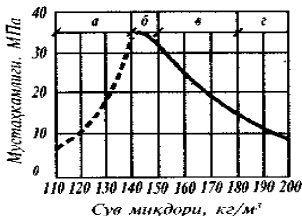
2-расм. Бетоннинг сиқилишдаги мустаҳкамлигининг сув миқдorigа боғлиқлиги: а–ўта қуюқ бетон қоришмаси (110 дан 140 л.гача); б–шунинг ўзи, энг юқори мустаҳкам ва зичланган (140–150 л.гача); в–шунинг ўзи, шгастик бетон қоришма (150 дан 180 гача); г–шунинг ўзи, қуйма суюқ бетон.
