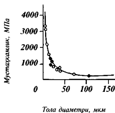
3-расм. Минерал толанинг йўғонлиги билан чўзилишдаги мустаҳкамлилиги орасидаги боғлиқлик.
