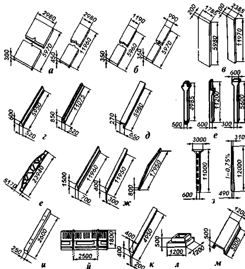
2-расм. Саноат биноларида йиғма темир-бетон конструкциялар турлари:
