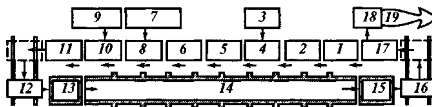
5-расм. Конвейер усулининг технологик схемаси: 1-қолипни тозалаш; 2- қолипни мойлаш; 3-арматура цеҳи; 4- арматура синчини ўрнатиш; 5-қолип деворларини маҳкамлаш; 6-арматурани таранглаш; 7-қўшимча арматура қисмлар; 8- қўшимча арматура қисмларни қолипга ўрнатиш; 9-бетон қоришма тайёрловчи цеҳ; 10- бетон қоришмани жойлаш; 11-бетон қоришмани зичлаш; 12- аравача; 13- кўтаргич; 14- қотириш хонаси; 15- совитиш; 16- аравача; 17- буюмларни жойлаш; 18-техник текшириш бўлими; 19-тайёр буюмлар омбори.
