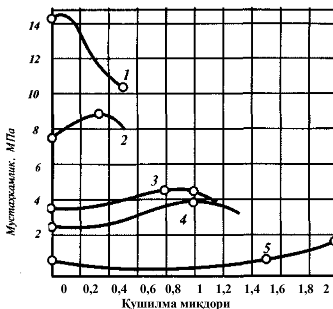
2-расм. Қўшиладиган оҳак ва тупроқнинг микдорига кўра қоришма мустаҳкамлигининг ўзгариши:
