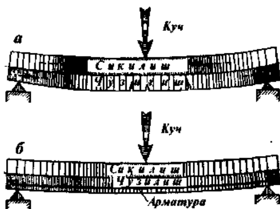
1- расм. Бетон ва темир-бетон тўсиннинг эгилиш схемаси: а- эгилиш кучи юқори, б- эгилиш кучи меъёрида
