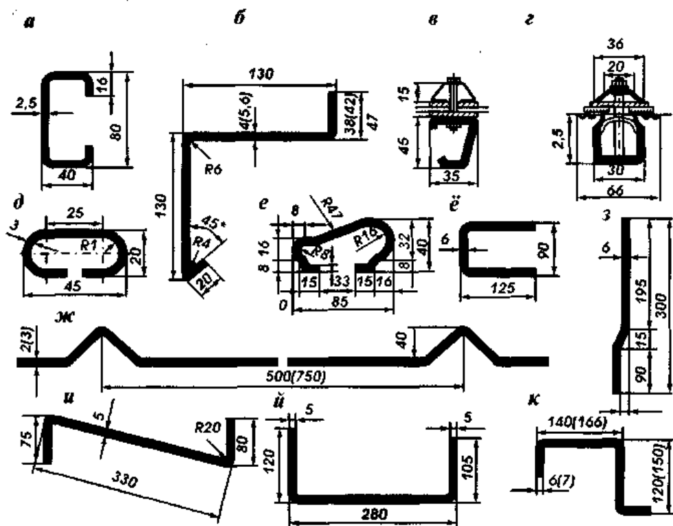
3-расм. Букилган узун пўлат буюмлар: а, б, д — юк кўтарувчи конструкциялар; в, г — деразобоп; е — зинапоя тутқичи; ё — резервуарбоп; з, ж, и, й, к — яроқли темир буюмлар.
