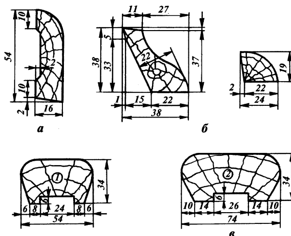
6-расм. Плинтус (а), галтель (б), зина тутқичлар (в).
