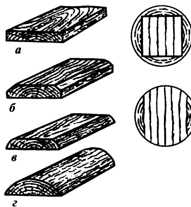
3-расм. Ёғоч тахталар: а—ҳамма томони тилинган тоза тахта; б-ярим тилинган тахта; в-кирраси тилинмаган тахта; г-пуштахта.
