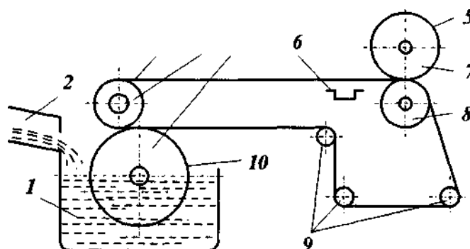
1-расм. Асбест-цемент буюмлари ишлаб чиқаришда ишлатиладиган қолипловчи машинанинг ишлаш схемаси: 1—чўян ванна; 2—асбест-цемент қуюқаси тушадиган тарнов; 3— конвейер тасмаси; 4— сиқувчи вал; 5—асбест-цемент бўтқа қатлами; 6— сўргич қутича; 7—бичувчи барабан; 8— бошқарувчи вал; 9—тортиб турувчи кичик вал; 10—пулат сим тўрли барабан.
