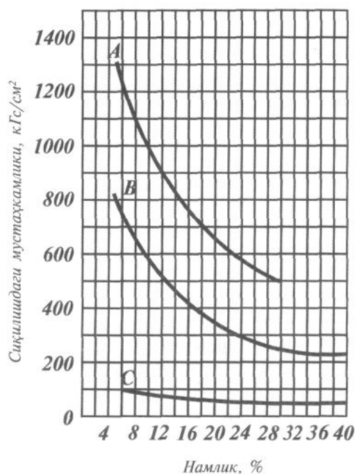
3-расм. Ёғоч мустаҳкамлигига намликнинг таъсири: а–кўндаланг эгилиши; б– толалар бўйлаб сиқилиши; с–толалари бўйлаб ёрилиши.
