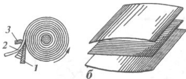
6-расм. Ёғочни қатламларга ажратиб тилиш (а) ва уларни ўзаро ёпиштириб (б) фанер тайёрлаш: 1–пичоқ; 2–шпон; 3– сиқиб турувчи мослама.
