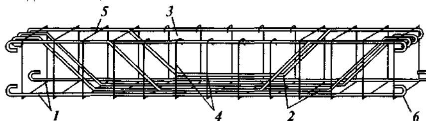
2-расм. Темир-бетон тўсинбоп арматура қовурға:
