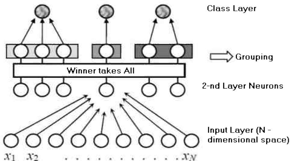
Рис.12. Структура нейронной сети Кохонена.
