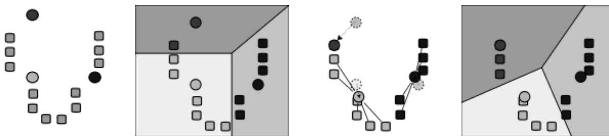
Рис 11. Обучение нейронной сети методом К-средних.
