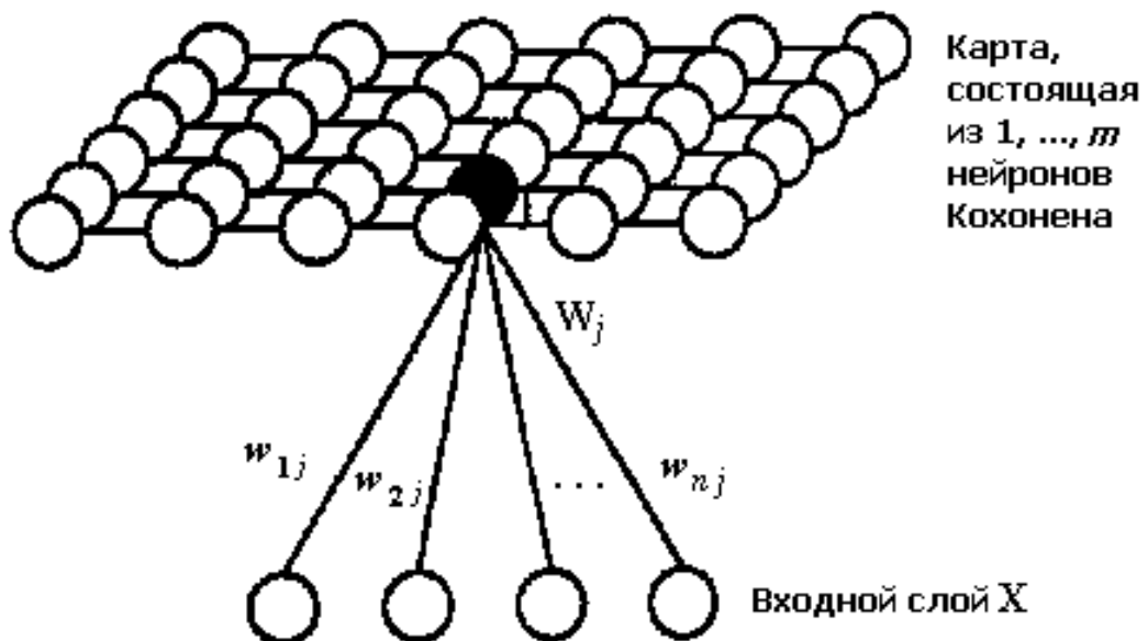
Рис. 7. Нейронная сеть Кохонена
