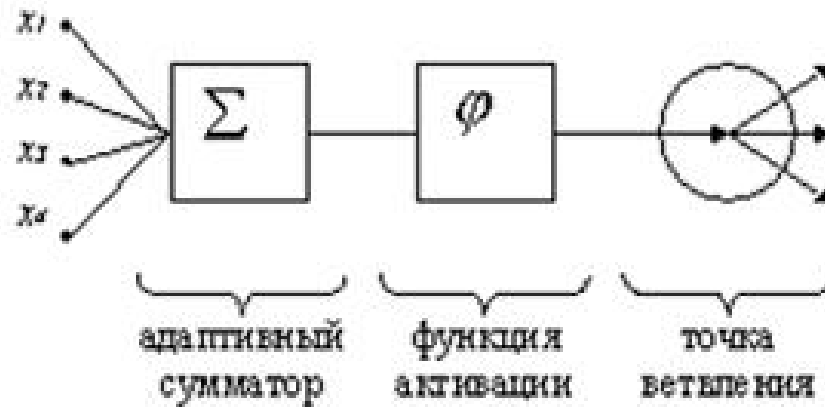
Рис. 9. Формальный нейрон
