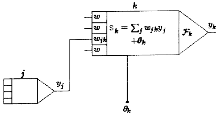
Рис. 6. Искусственный нейрон – простейший элемент искусственной нейронной сети
