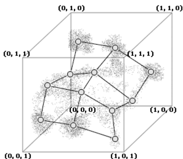
Рис 10. Обученные нейроны в 3х мерном пространстве признаков.
