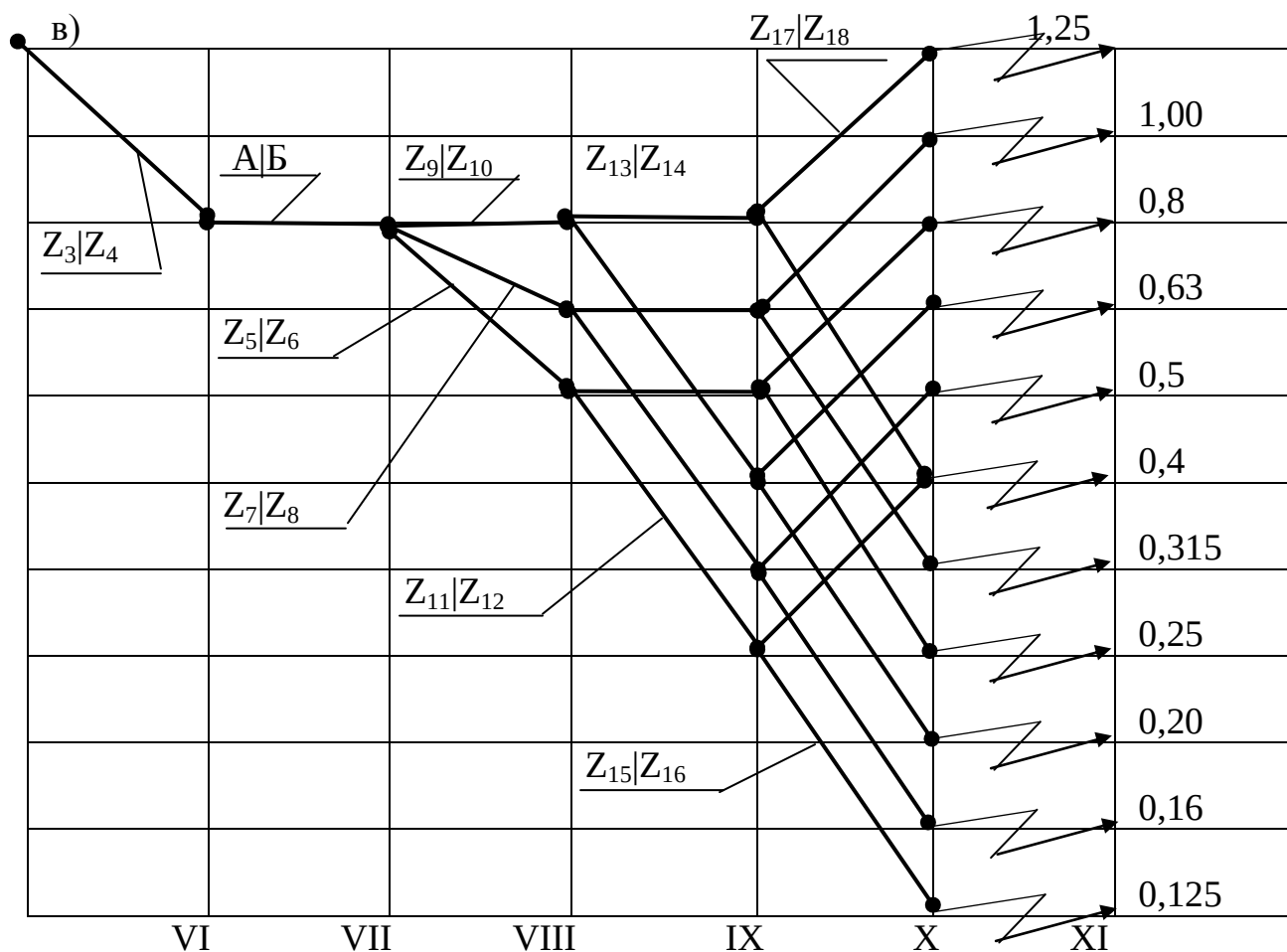
2.2-расм. Дастгоҳнинг суриш ҳаракати узатмаси:
