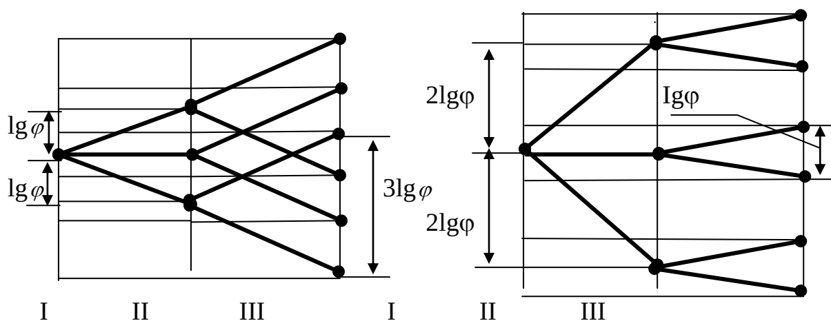
2. 3- расм. Олти поғонали узатманинг таркиб тўрлари.
