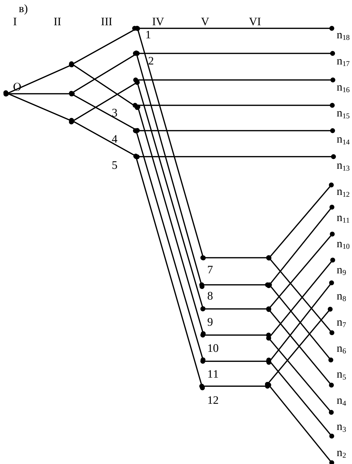
2.11 – расм. Z=18 , \phi = 1,416 ўлган узатманинг таркиб тўри(в).
