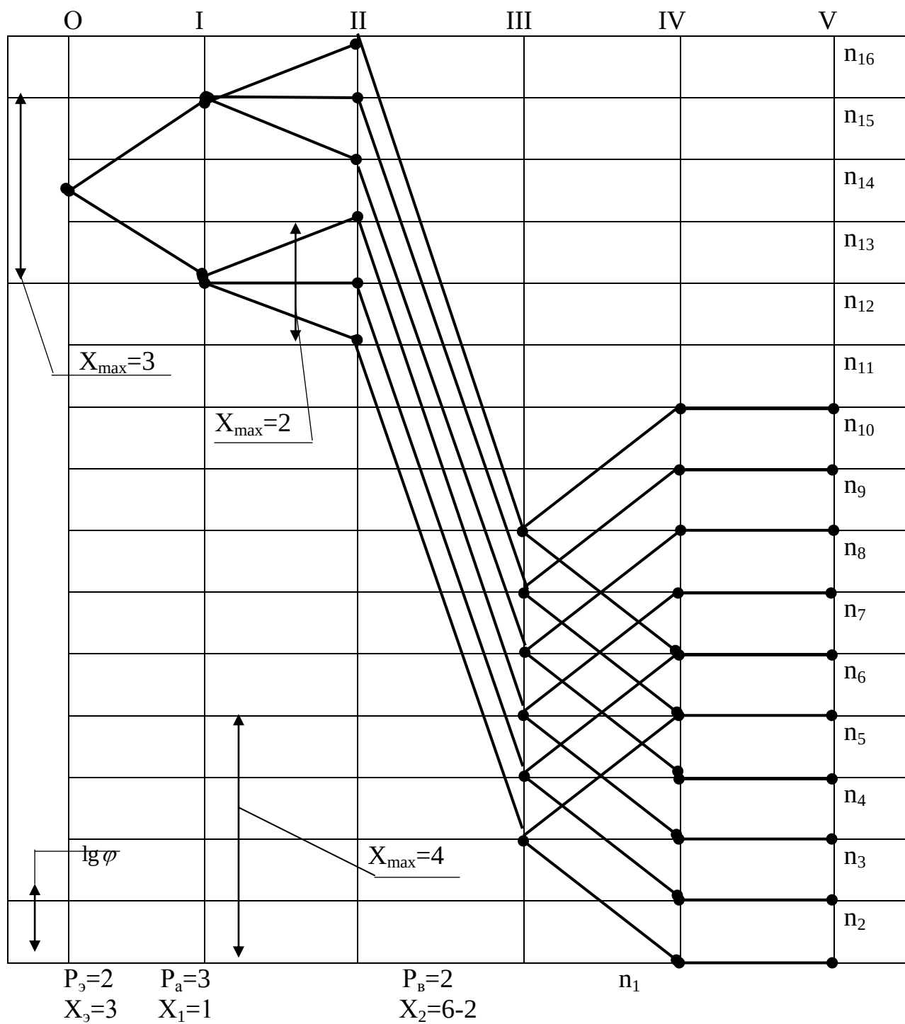
2.1а-расм. Дастгоҳнинг бош ҳаракат узатмаси таркиб тўри.
