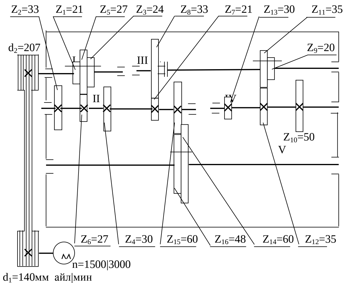
2.16-расм. Дастгоҳнинг бош ҳаракат узатмаси кинематик схемаси.
