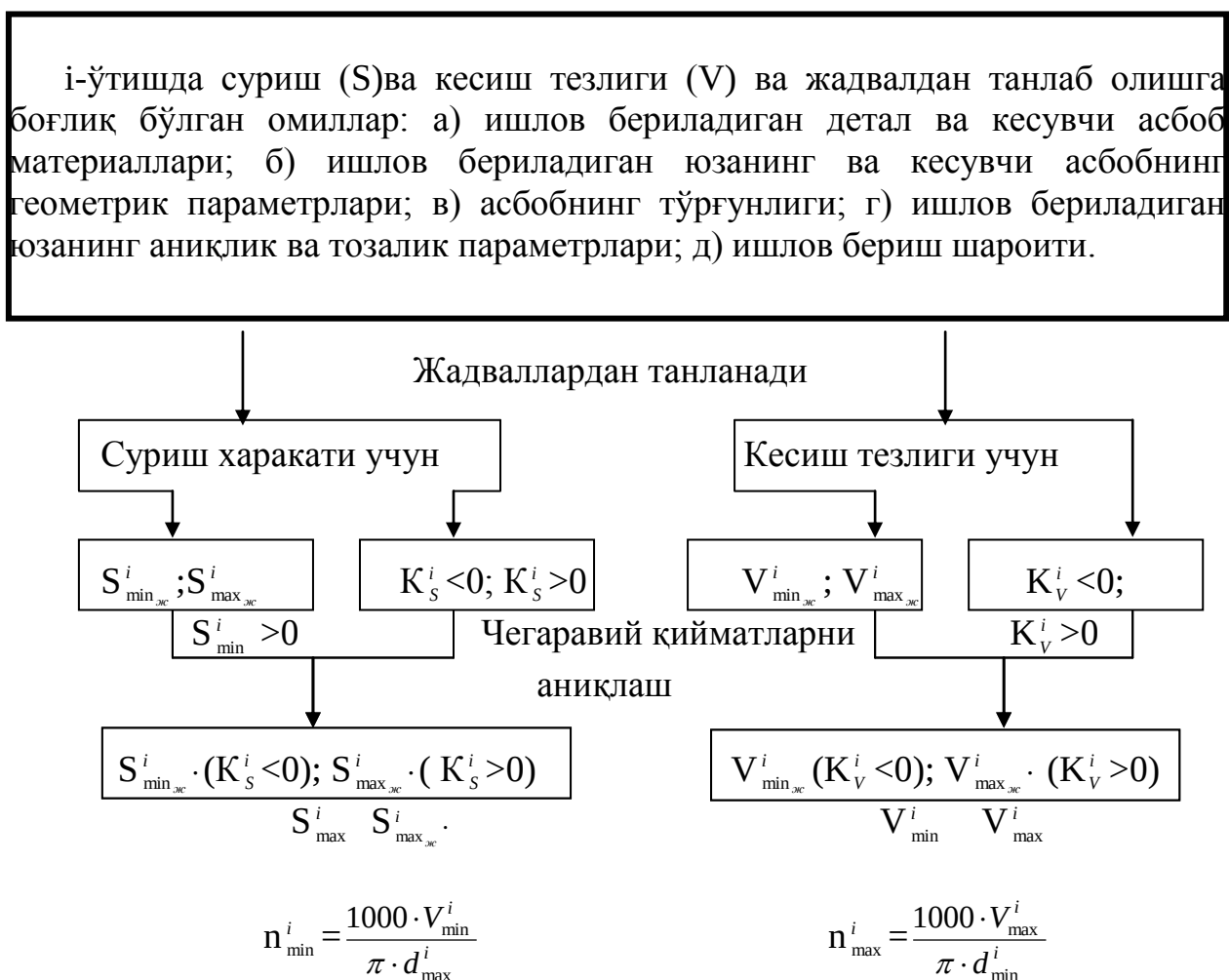
I.1–расм. Жадвал усули билан суриш ва кесиш тезлигининг чегаравий қийматларини танлаш схемаси.
