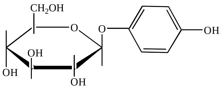
Арбутин
