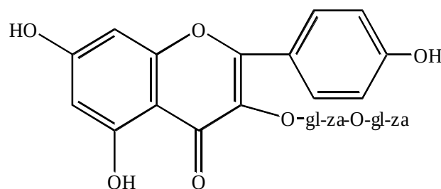
Кемефол 3-софороид
