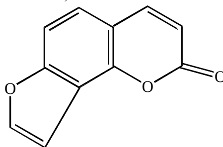
Изопсорален (ангелицин)
