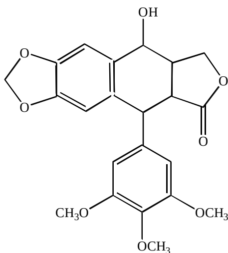
Подофиллотоксин
