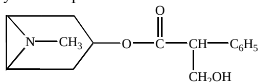
Гиосциамин
