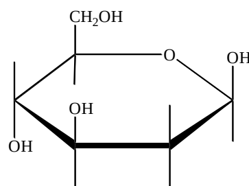
D - дигитоксоза
