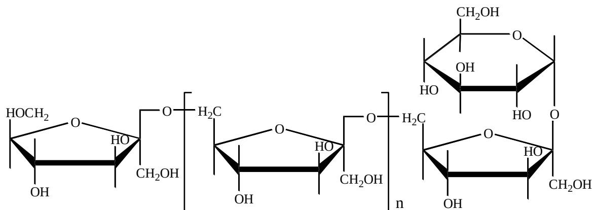
Инулин
