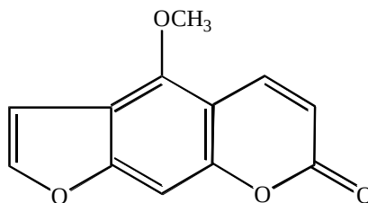
Бергаптен
