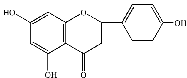
Апигенин
