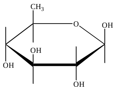
L - рамзона
