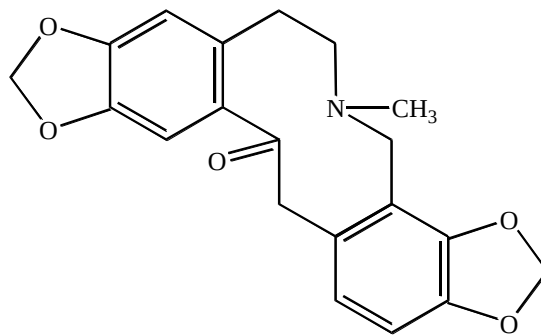
Протопин
