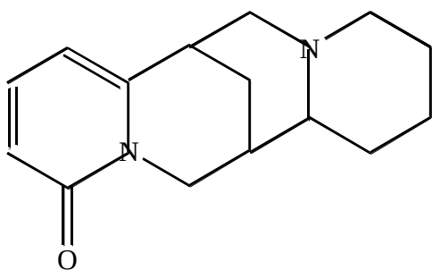
Термопсин
