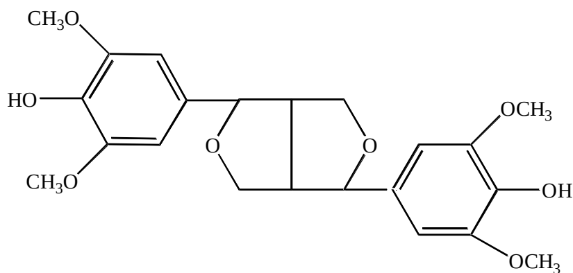
Сирингорезинол
