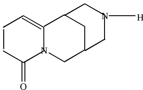
Цитизин
