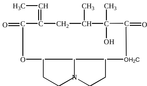
Платифиллин
