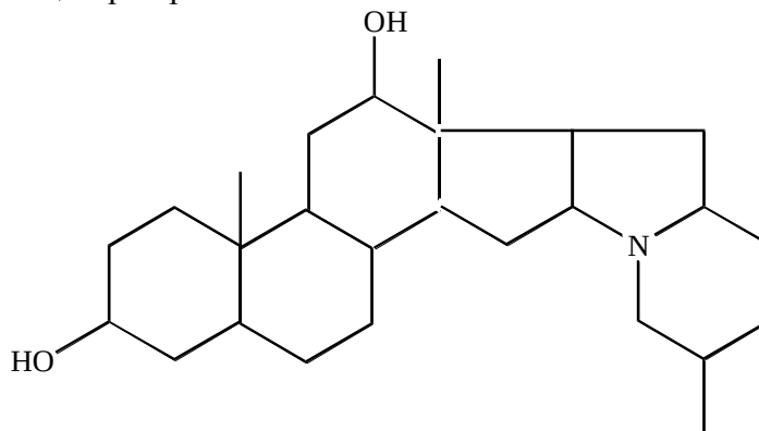
Рубимервин
