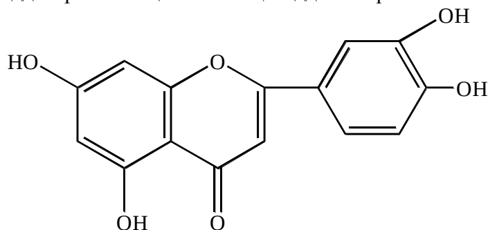
Лютеолин
