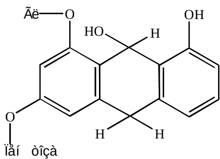
Жестерин
