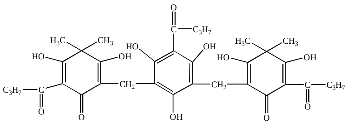
Филикс кислотаси
