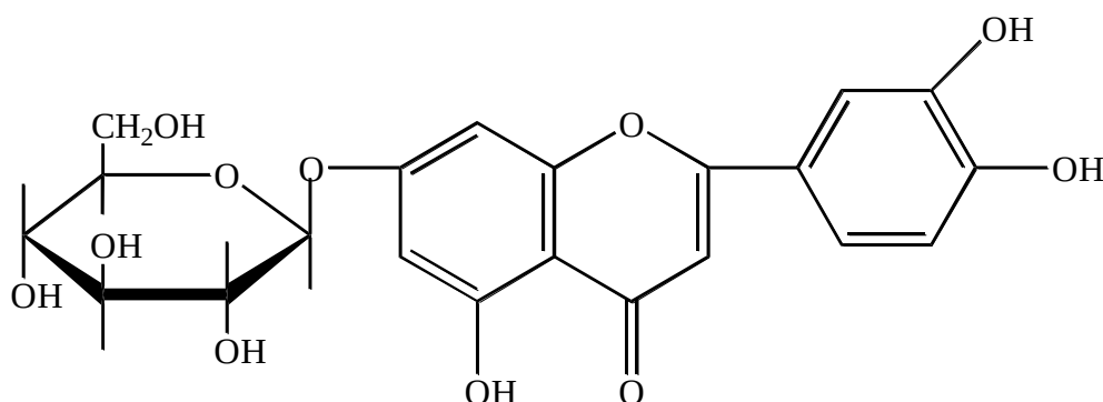
Цинарозид
