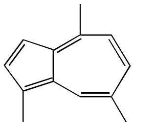
Хамазулен
