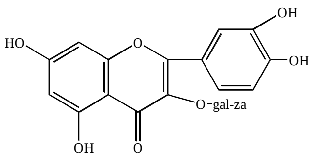
Гиперозид
