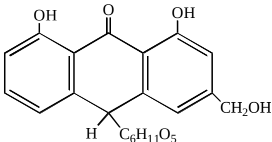
Алоин
