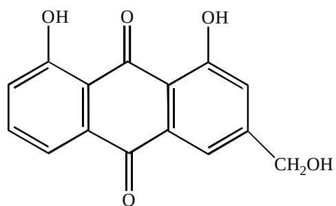
Алоэ эмодин
