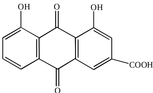
Реин
