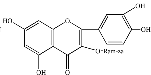
Кверцетрин
