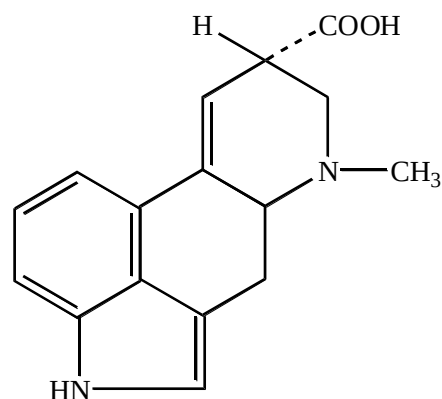
Изолизергин кислотаси
