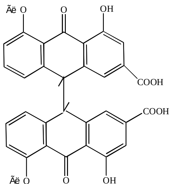
Сеннозид А,В
