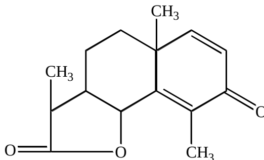
Сантонин
