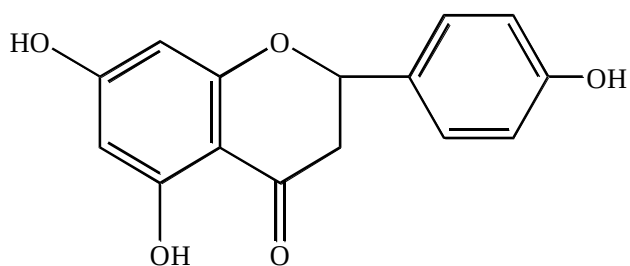
Нарингенин
