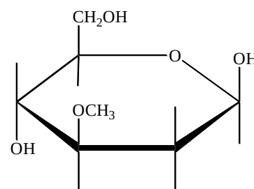
D - цимароза
