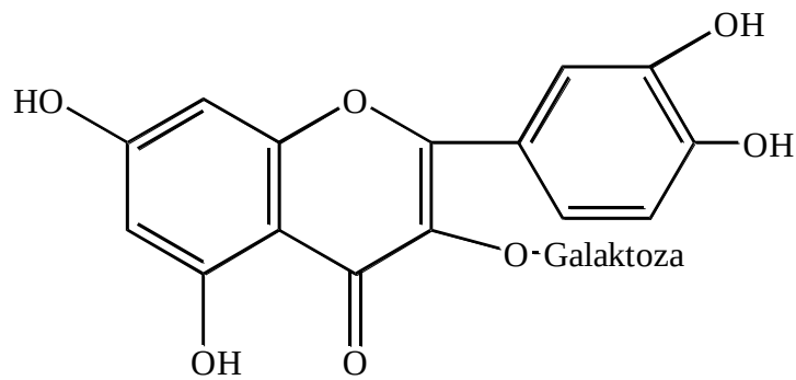
Гиперозид
