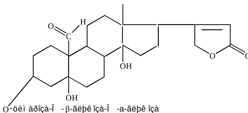
К- строфантозид
