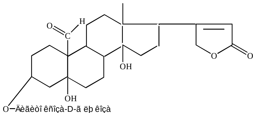
Эризимозид
