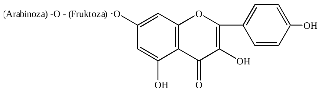
Эквизетерин
