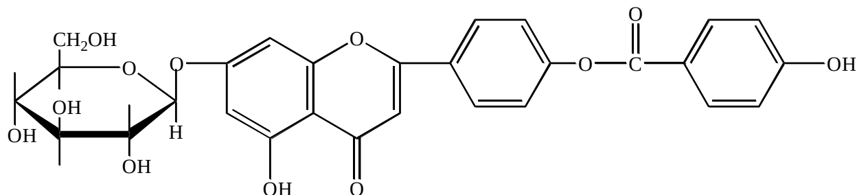
Квинквелозид
