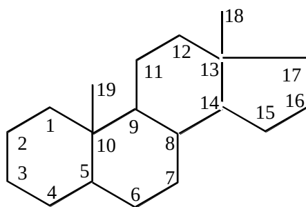
Циклопентан пергидрофенантрен
