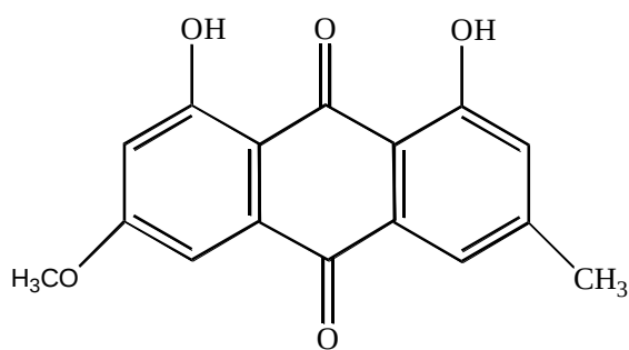
Фиоцион (реохриаин)
