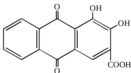
Псеудопурпурин
