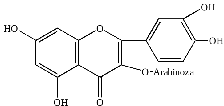
Авикулярин
