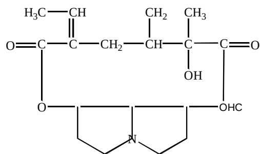
Сенецифиллин
