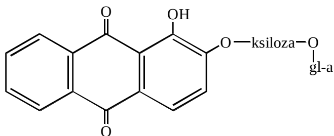
Руберитрин кислота
