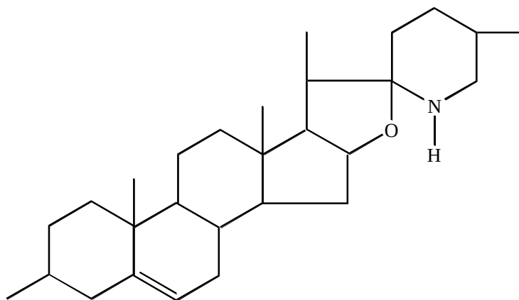
Соласодин
