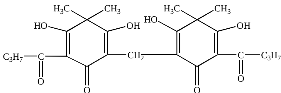
Альбаспидин
