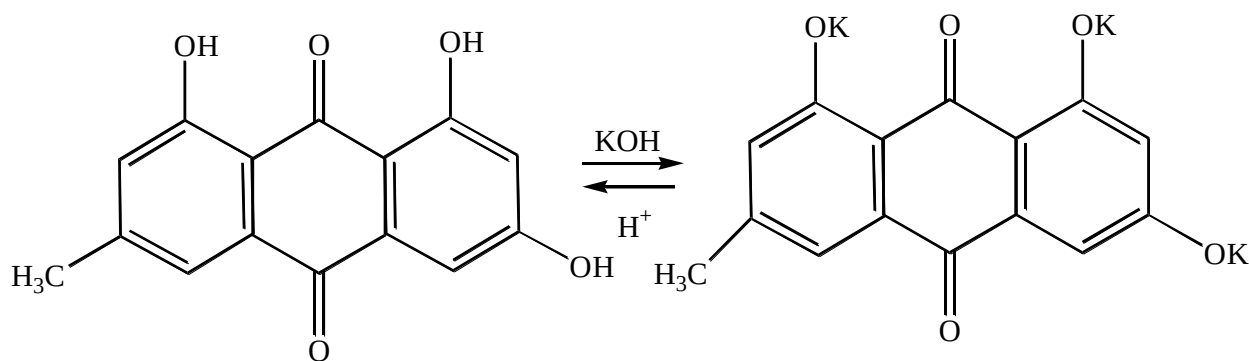
Реум эмодин
