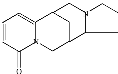
Пахикарпин
