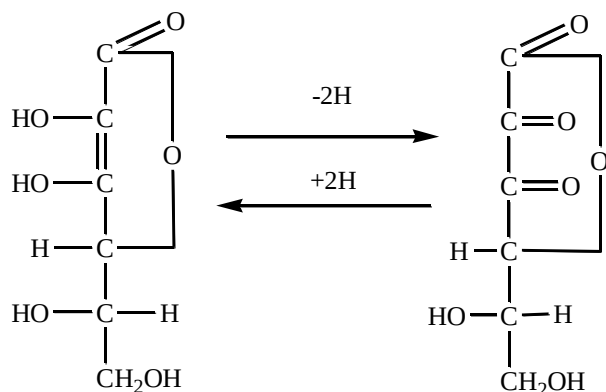
α-Аскорбин кислота
