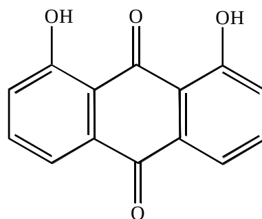
Хриаофанол
