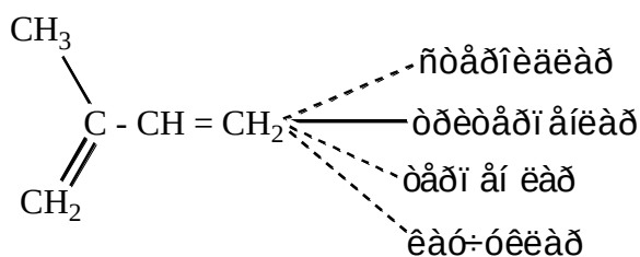
Изопрен
