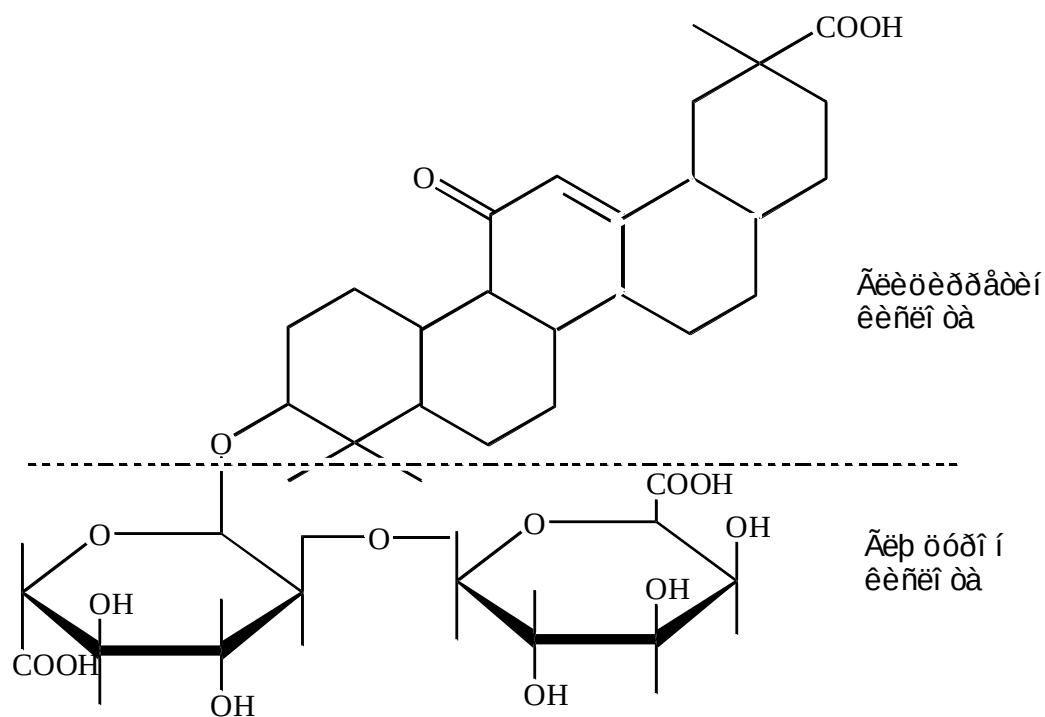
Глицирризин кислота
