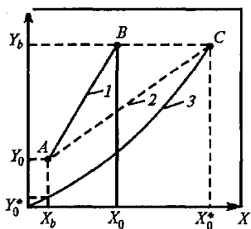
25.2-rasm. Absorbsiya jarayonining ish va muvozanat chiziqlari:
