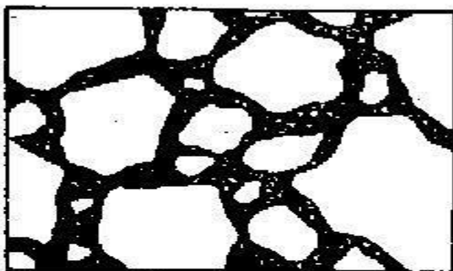
-расм. Бетон тузилиши (оч рангда йирик тулдиргич заррачалари, қора рангда-цемент тош)
