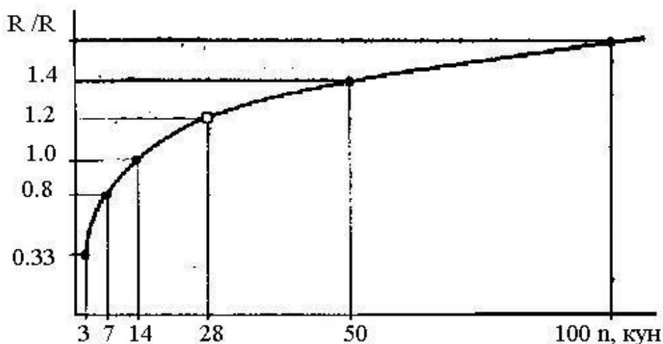
-расм. Бетон мустаҳкамлигининг вақт бўйича ўзгариши (R -бетоннинг маркадаги мустаҳкамлиги, n-кунлар давомида қотиш вақти)
