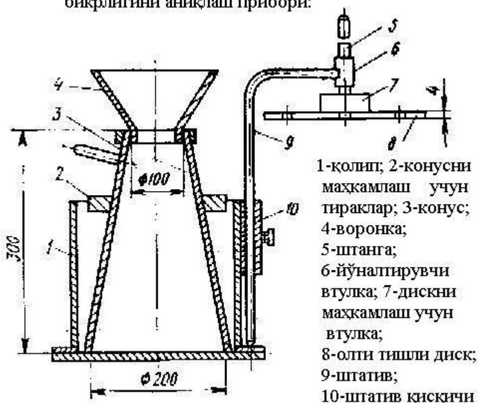
-расм. Бетон аралашмасининг бикрлигини аниқлаш прибори:
