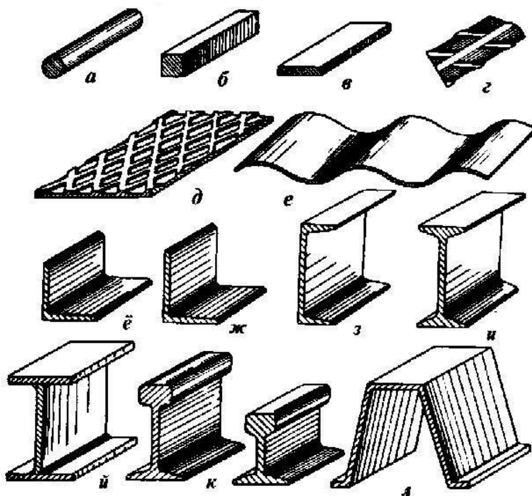
-расм. Пўлат навлари: а-думалок; б-квадрат; в-тасмасимон; г-такрорий узун; д-тарам-тарам; е-тўлкинли; ё-тенг бурчакли; ж-тенг бўлмаган бурчакли; з-швеллер; и-қўштавр; й-пайвандланган қўштавр; к-темир йўл изи (рельси); л-деворбоп шпунг.
