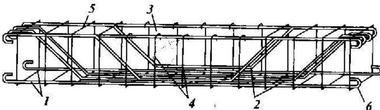
-расм. Темир-бетон тўсинбоп арматура қовурға: 1-тўғри арматуралар; 2-ўрдаксимон букылган арматуралар; 3-монтаж арматуралар; 4-очик хомуллар; 5-туташ хомуллар; 6-анкер илмоқлар.
