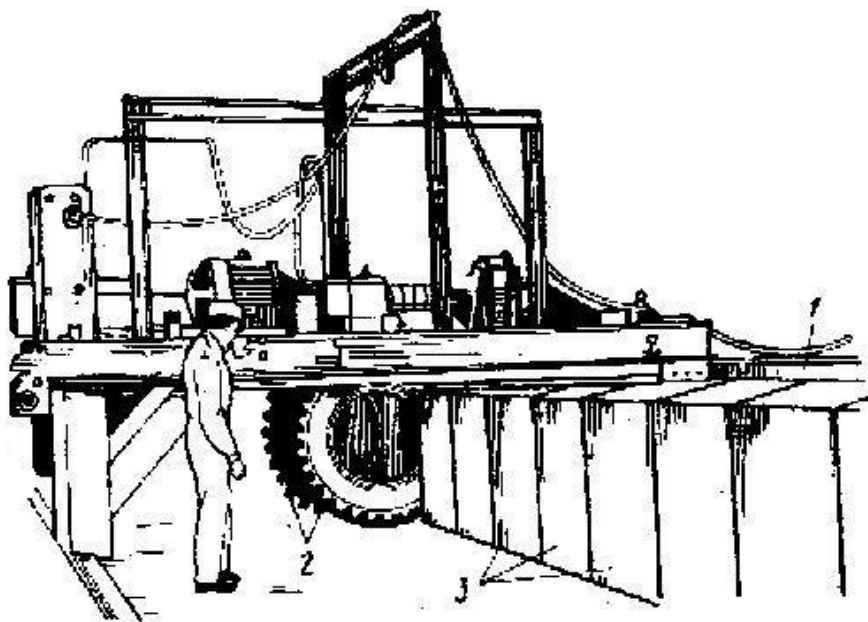
5-расм. Тош кесиш машинаси ёрдамида юмшоқ жинслардан олинган йирик блокларни арралаш: 1-рельслар; 2-кесувчи фреза; 3-блоклар.
