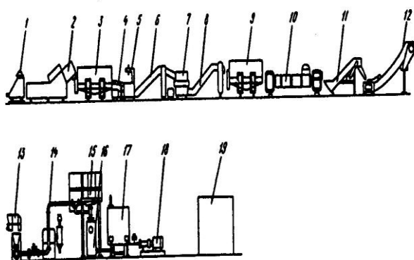
20-расм. Қад ва қабачқиларни тайерлаш комплекс жихози.
