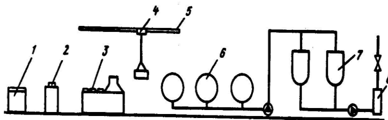
19-рasm Суякли шурва тайерлаш технологик схемаси
