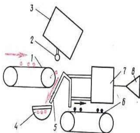
2-расм. Помидорларни фотоэлектрон ажратиш схемаси
