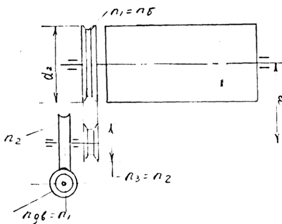
2.4- расм. Ҳаракат ўзатиш механизмларининг кинематик схемаси
