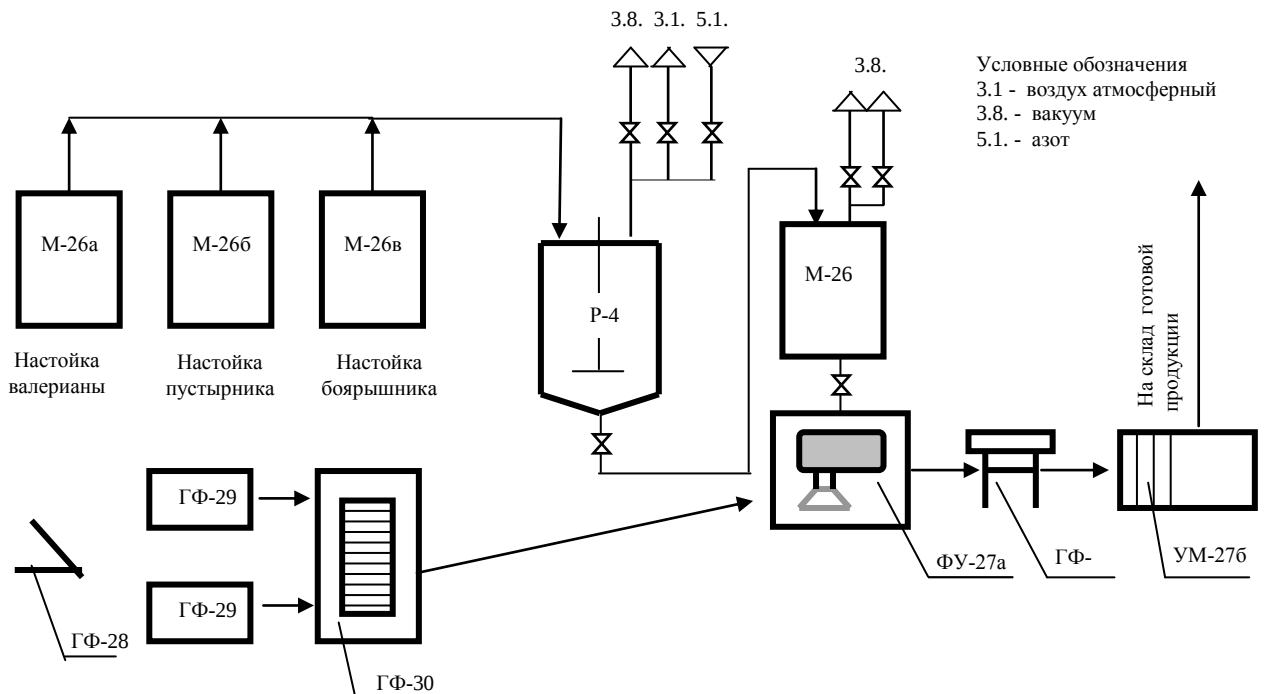
Рис. 5. Аппаратурная схема производства препарата «Триогален»
