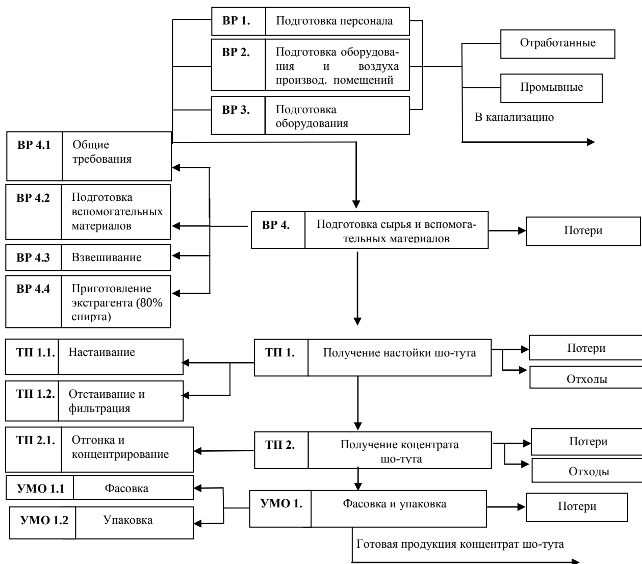
Рис. 1. Технологическая схема производства концентрата шо-тута
