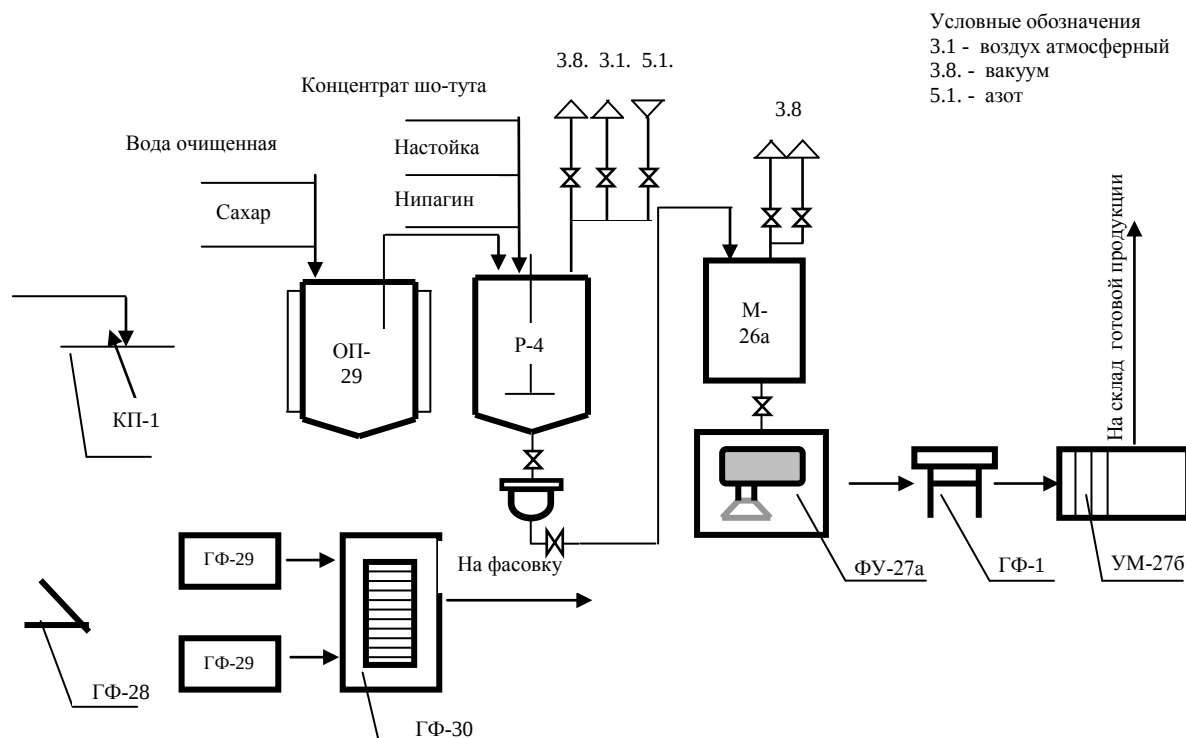
Рис. 3. Аппаратурная схема производства препарата «Сироп боярышника с шо-тутом»
