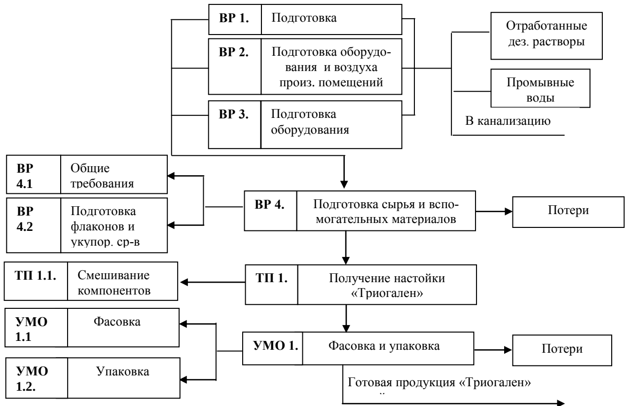
Рис. 4. Технологическая схема производства препарата «Триогален»
