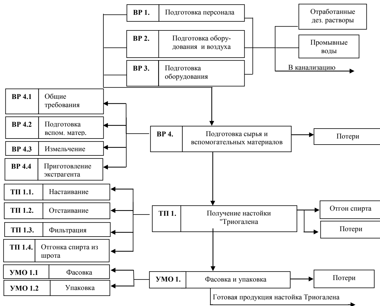
Рис. 6. Технологическая схема получения препарата «Триогален»
