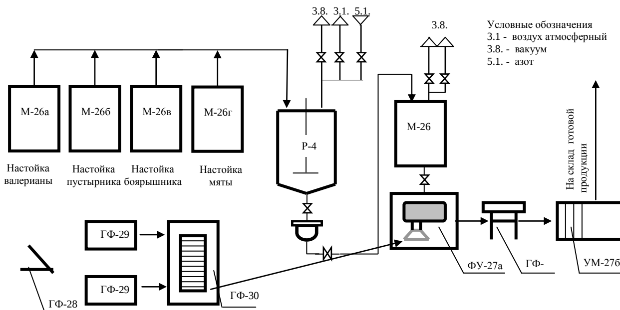
Рис. 8. Аппаратурная схема производства препарата «Фитогален»
