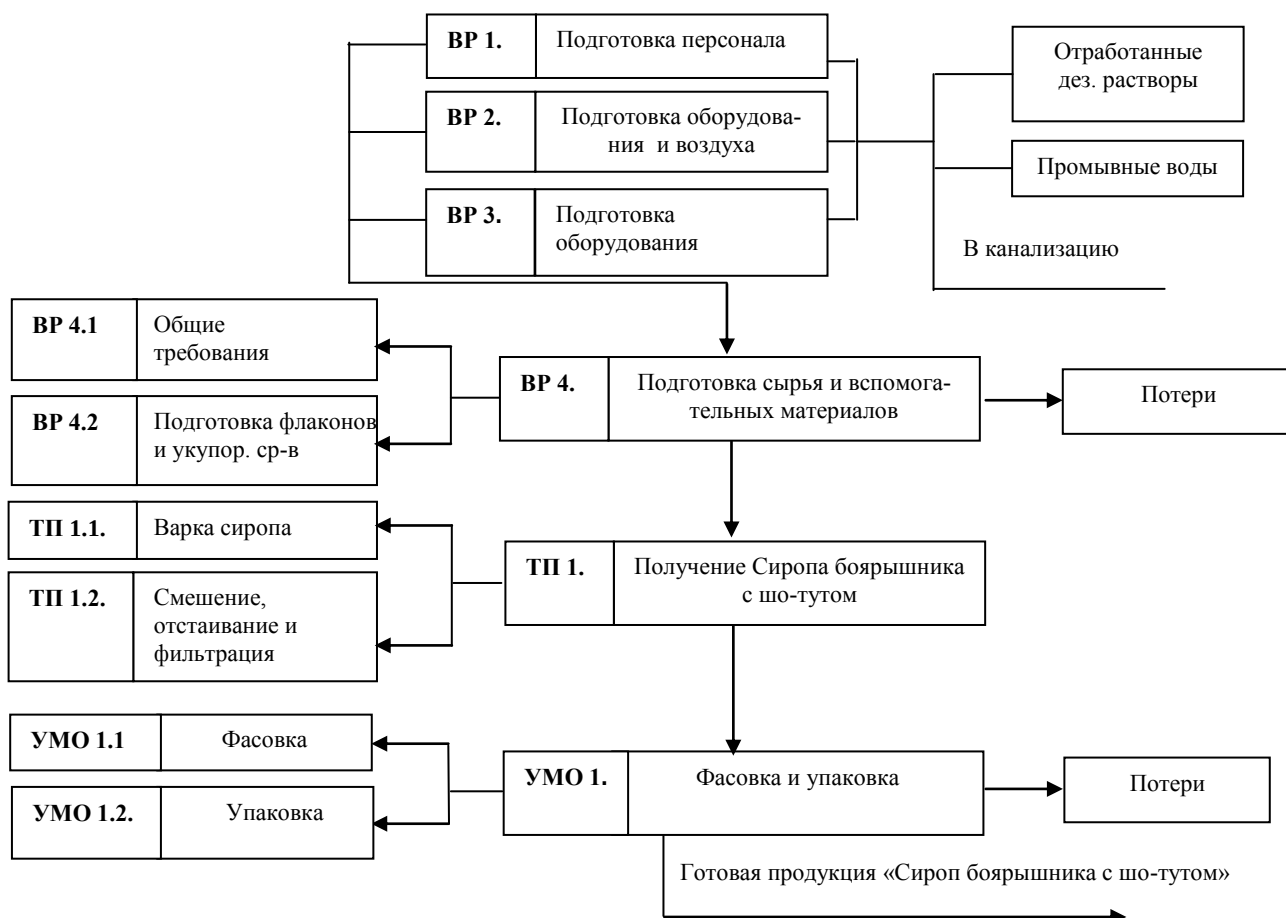
Рис. 2. Технологическая схема производства препарата «Сироп боярышника с шо-тутом»
