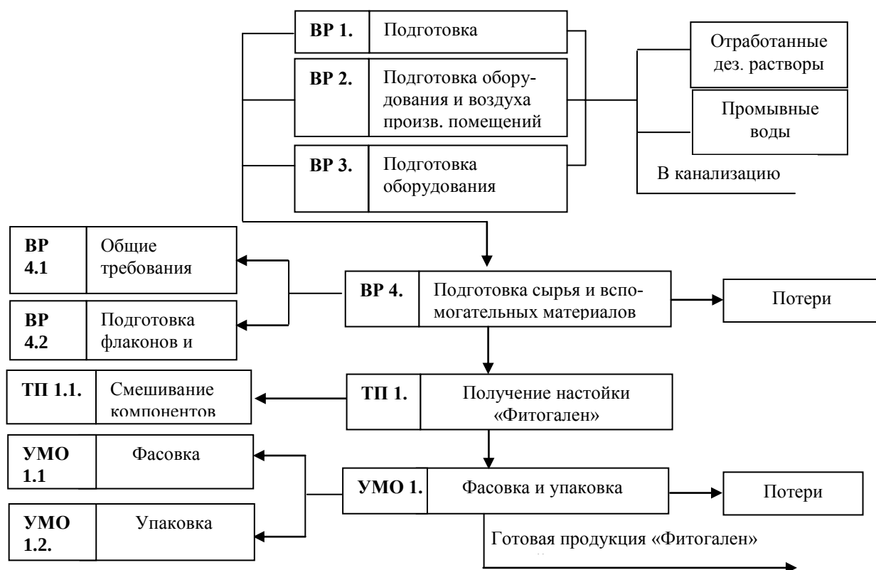
Рис. 7. Технологическая схема производства препарата «Фитогален»
