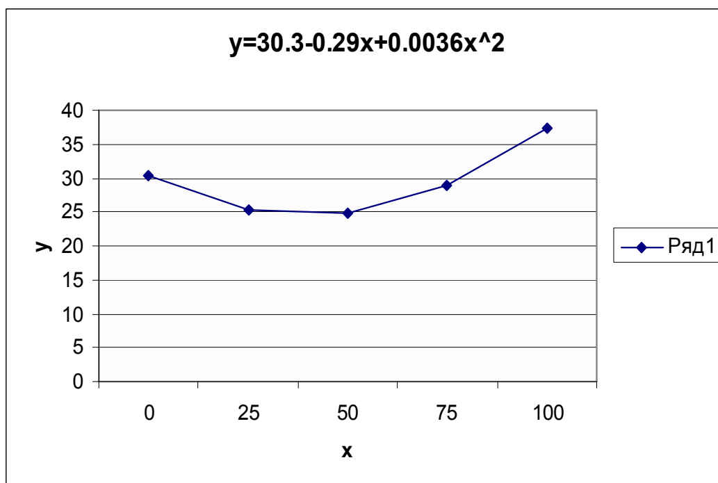
Рис.3.2 Закономерность изменения натяжения нитей основы по ширине заправки челночных станков типа АТ после модернизации.
