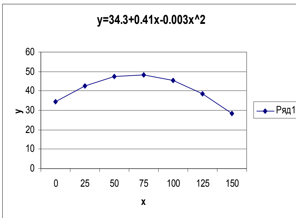
Рис. 3 Закономерность изменения натяжения нитей основы по ширине заправки микрошелочных станков.
