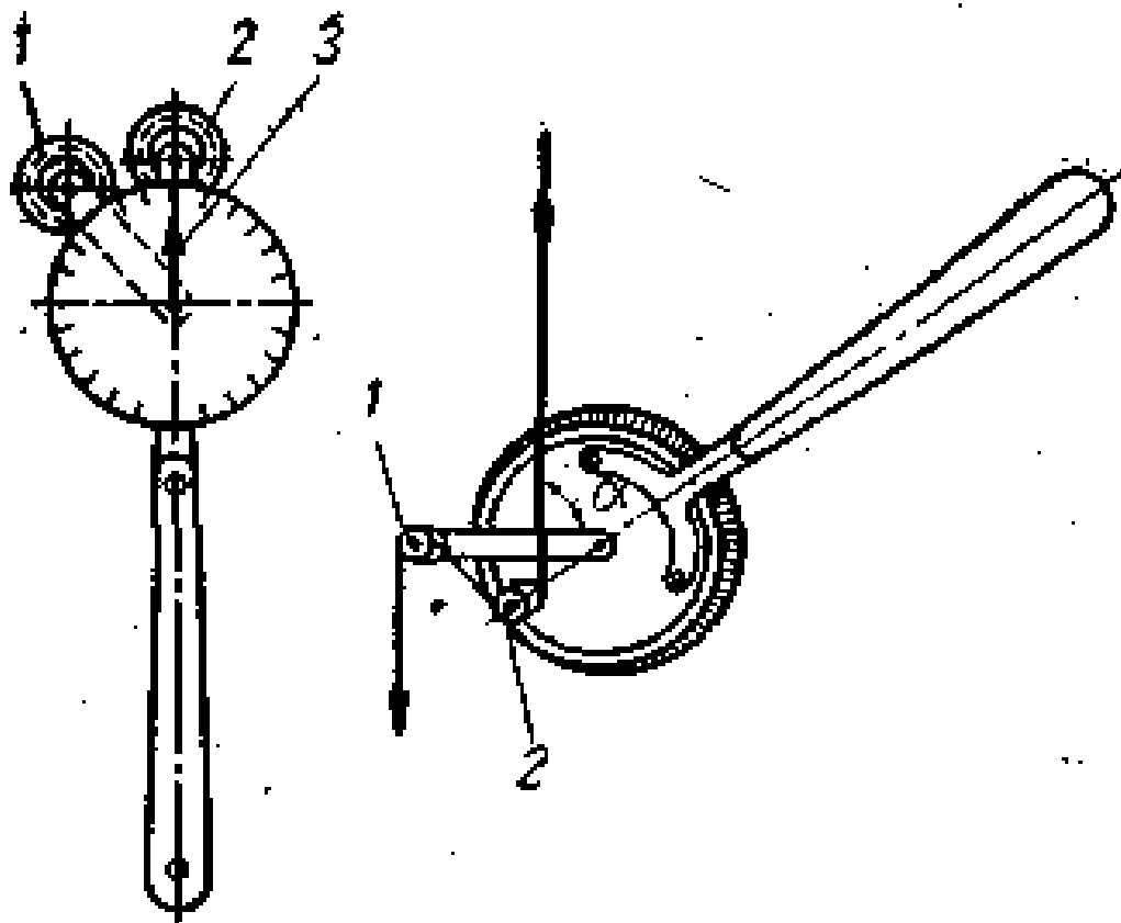
Рис. 1.7. Прибор HH-2 для измерения натяжения одиночных нитей
