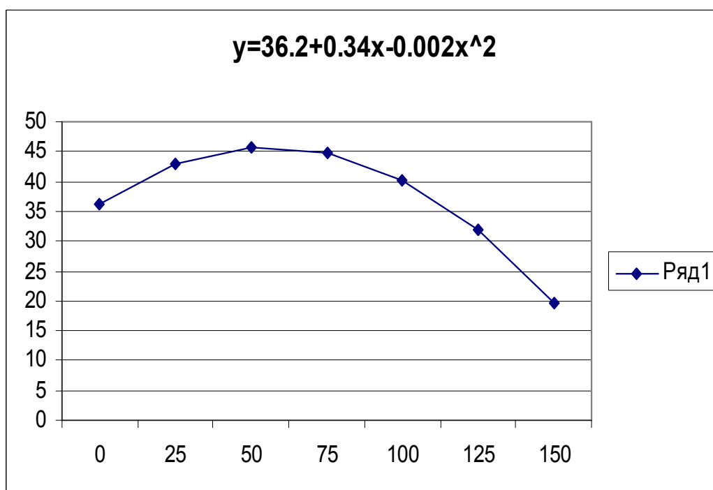
Рис. 4 Закономерность изменения натяжения нитей основы по ширине заправки рапирных станков.
