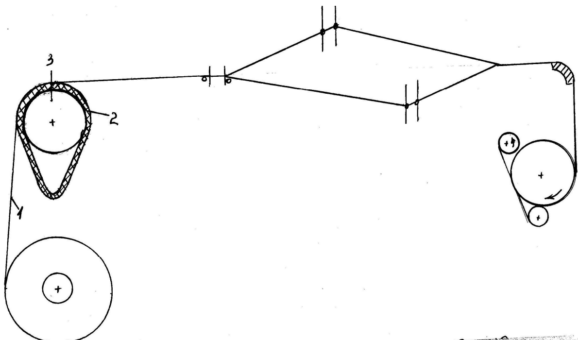
Рис.3.1.Стабилизатор натяжения нитей основы по ширине заправки ткацких станков
