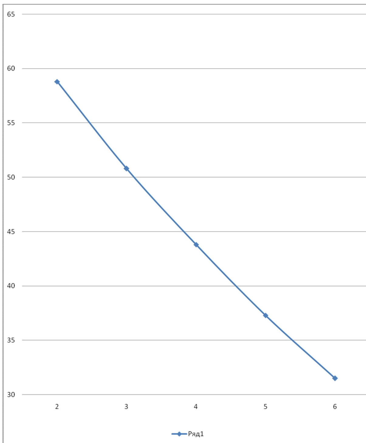
Рис.2.9. Зависимость количества слабо натянутых нитей от заправочного натяжения.
