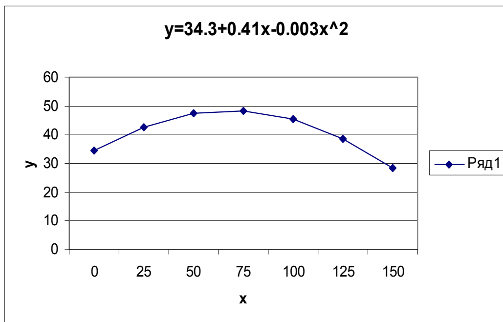
Рис.3.4. Закономерность изменения натяжения нитей основы по ширине заправки микрошелочных станков типа СТБ после модернизации.
