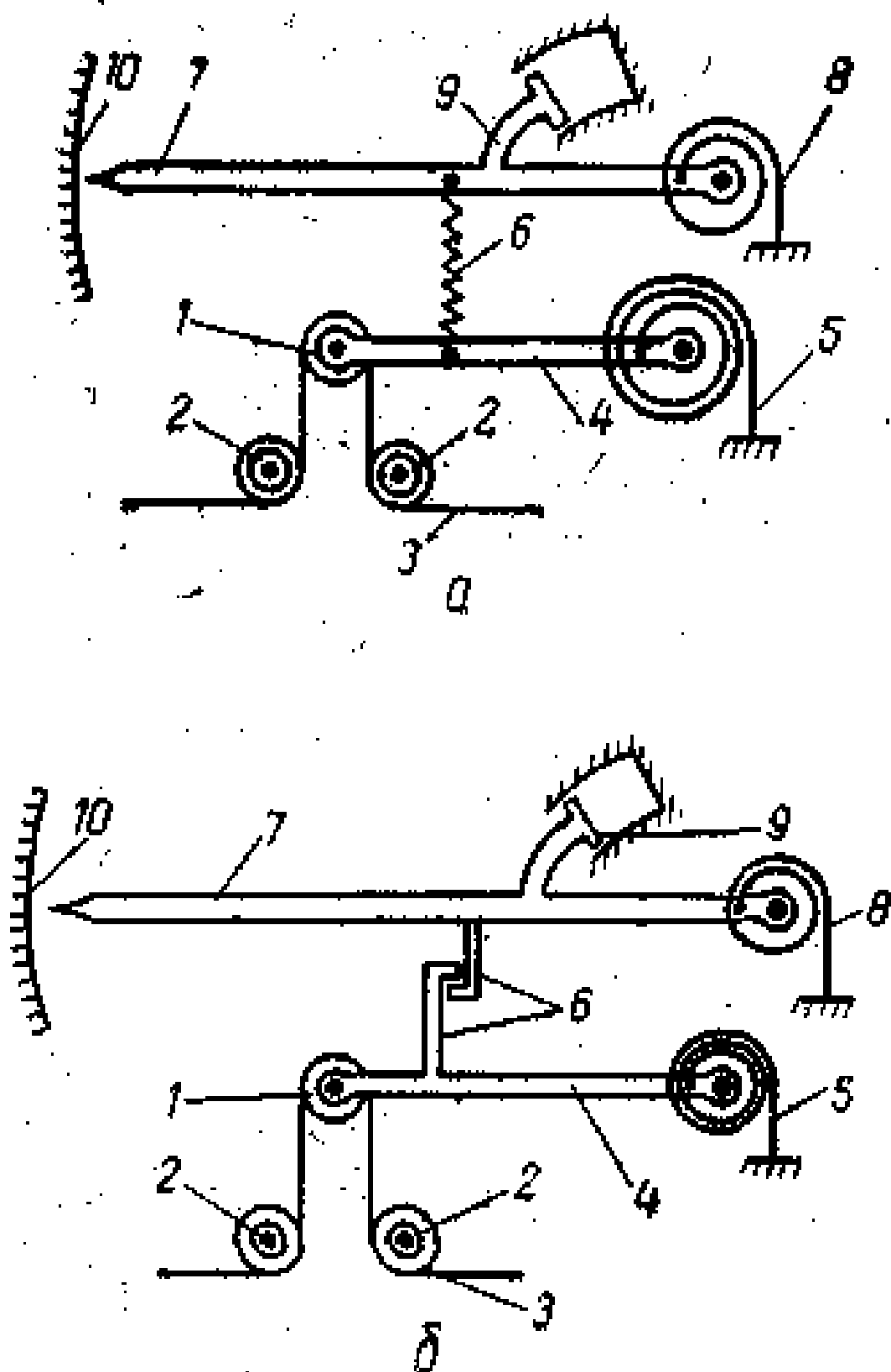
а - схема прибора для измерения средней величины натяжения; б - схема прибора для измерения наибольшей величины натяжения.
