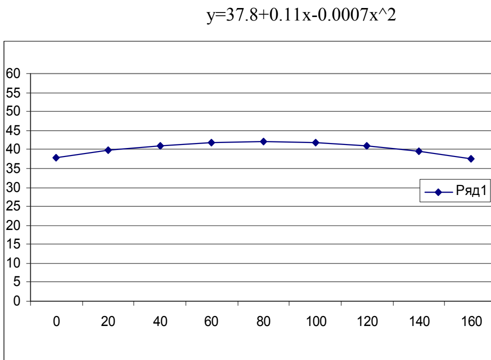
Рис.3.5. Закономерность изменения натяжения нитей основы по ширине заправки рапирных станков типа Р после модернизации.
