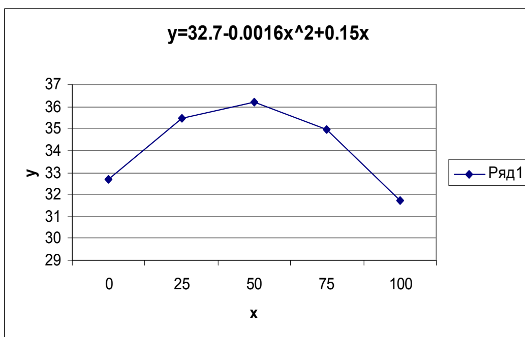
Рис.3.3 Закономерность изменения натяжения нитей основы по ширине заправки пневморайрных станков типа АТПР после модернизации.
