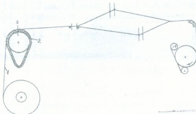
Рис.1.Стабилизатор натяжения нитей основы по ширине заправки ткацких станков
