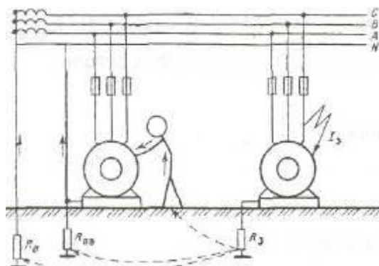
17.7.-rasm. Nollashtirilmagan elektr uskunasi setidagi tutashish.
