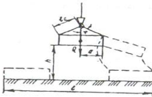
16.2.-Rasm. Yuk arqoni uzilganda xavfli zona chegarasini aniqlash sxemasi.
