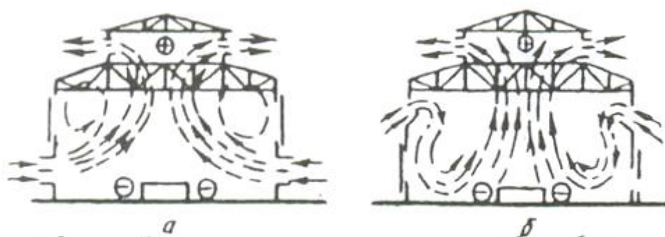
9.3.-rasm. Havo zichligi har xilligi hisobiga amalga oshadigan havo almashish sxemasi.
