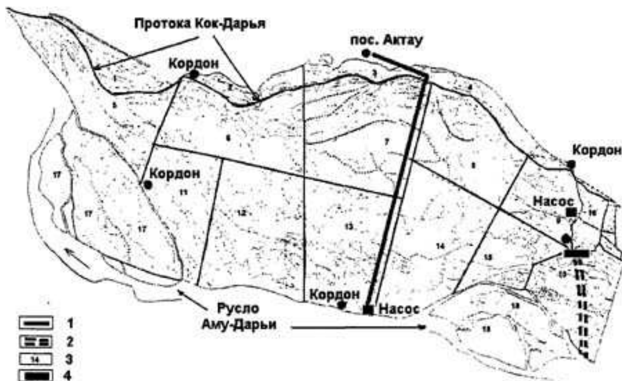
4-su`wret. Baday tog`ay qorıqhanası suwg`arıw sxeması.
