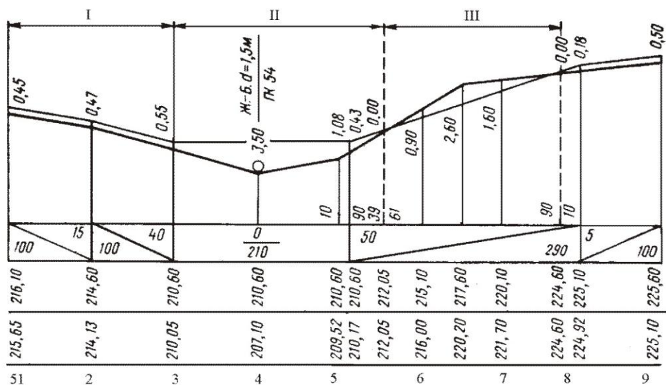
43-rasm. Bo'ylama profilda yo'lining joylashishi
