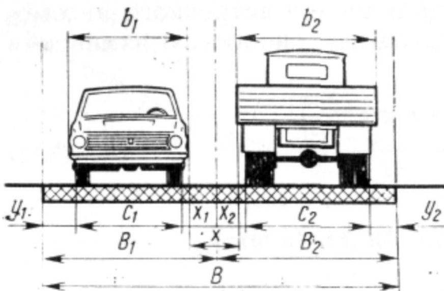
54-rasm. Yo'l qatnov qismini aniqlash chizmasi
