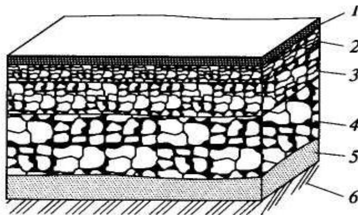
56-rasm. Yo'l to'shamasi:
