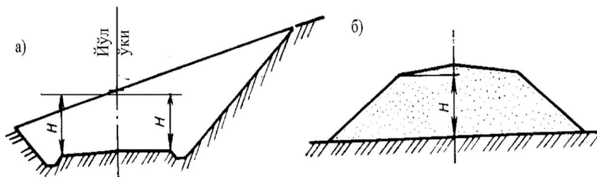
52-rasm. Yo'l poyining ishchi belgisi: a - o'ymada; b - ko'tarmada.
