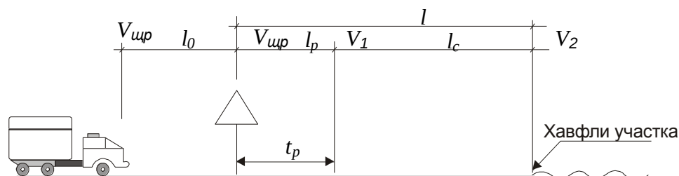
81-rasm. Xavfli uchastkadan oldin qo'yiladigan yo'l belgisi masofasini aniqlash sxemasi
