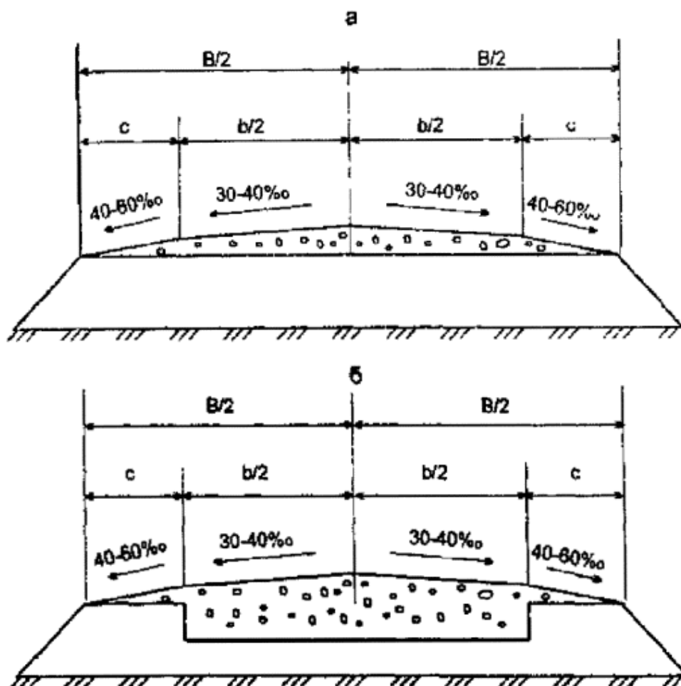
32-rasm. Xo'jalik yo'llari ko'ndalang kesimlari
