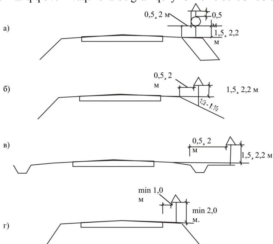
83-rasm. Aholi yashamaydigan joylarda yo'l belgilarini ko'ndalang kesimda joylashtirish
