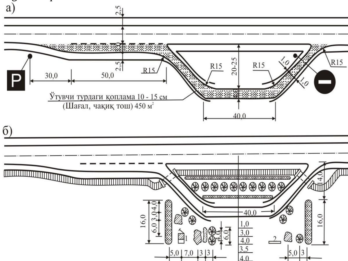
80–rasm. 5 ta yengil avtomobilga mo'ljallangan dam olish maydonchasini loyihalashga misol. a – dam olish maydonsaini andozaviy loyihasi; b – maydonchani ko'kalamzorlashtirish rejasi; 1 – hojatxona; 2 – o'rindiqlar.
