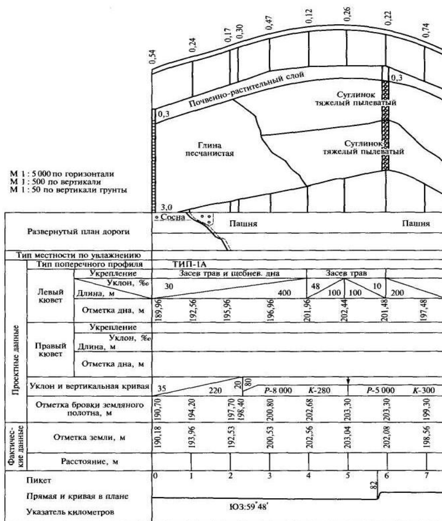
50-рasm. Yo'lning bo'ylama kesimi elementlari
