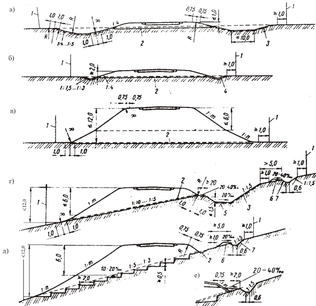
54-rasm. Ko'tarmada o'tgan yo'l poyining ko'ndalang kesimlari:
