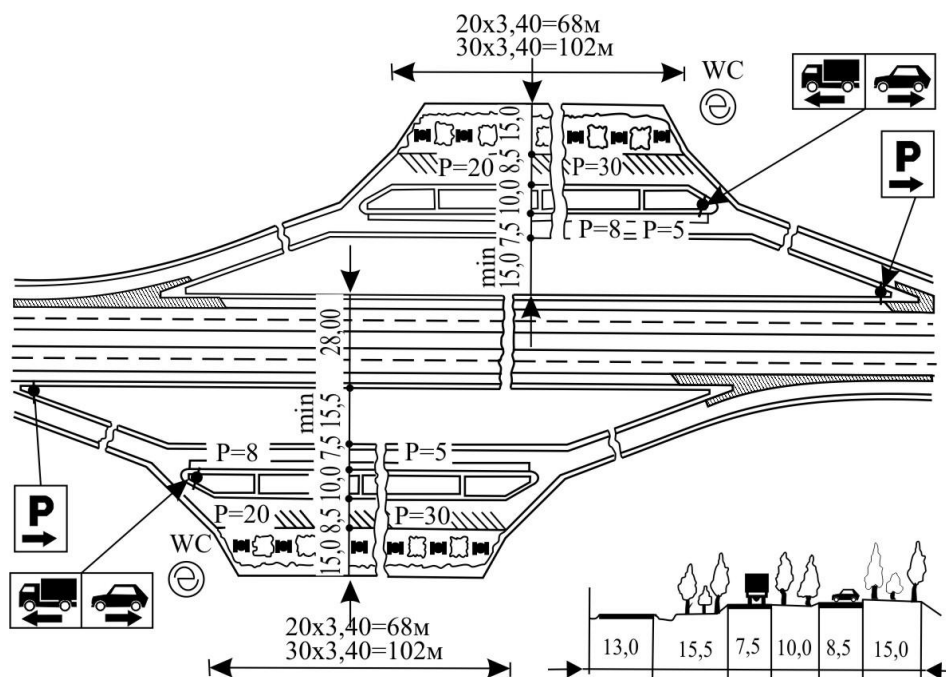
78–rasm. Avtomobil magistrallarida dam olish maydonlarini rejalashtirish andozalari.
