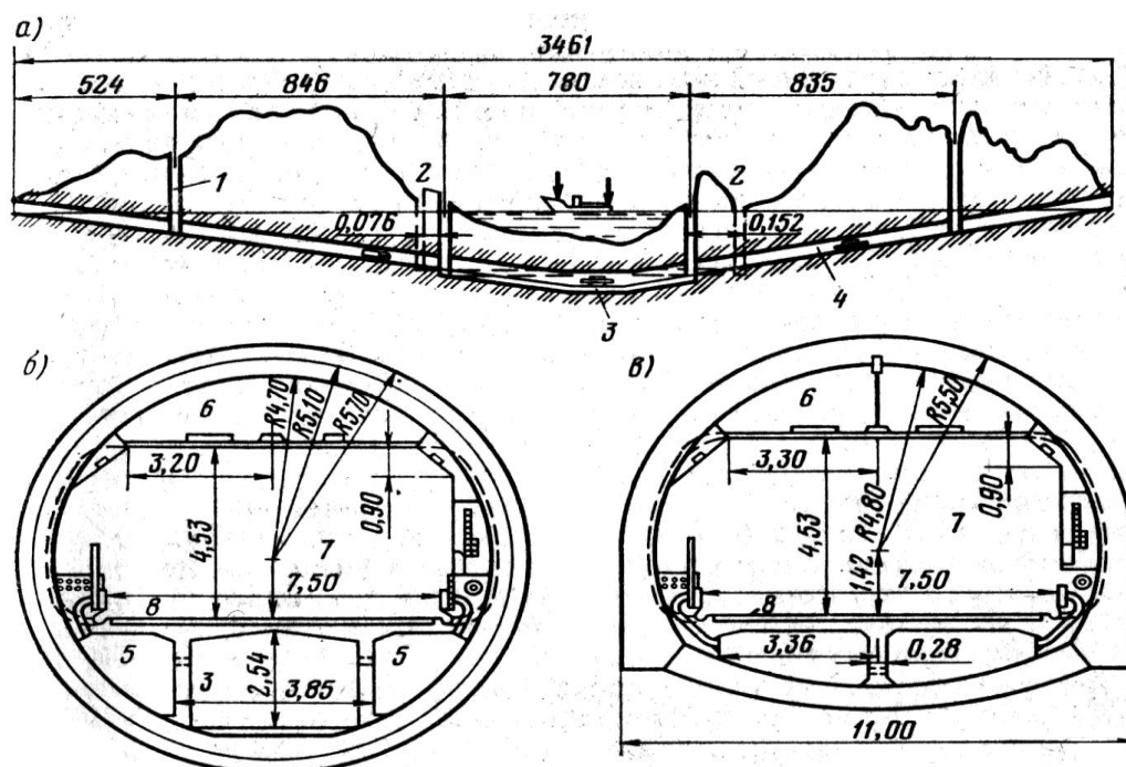
67-rasm. Suvosti tunelli:
