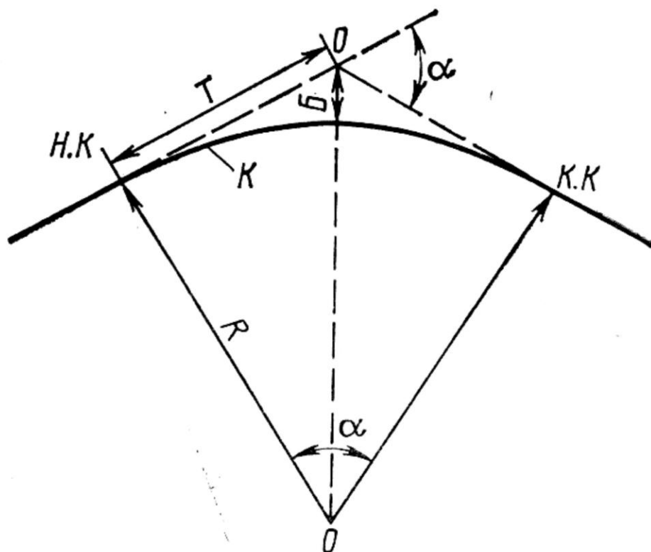
48-rasm. Aylanma egrilik elementlari
