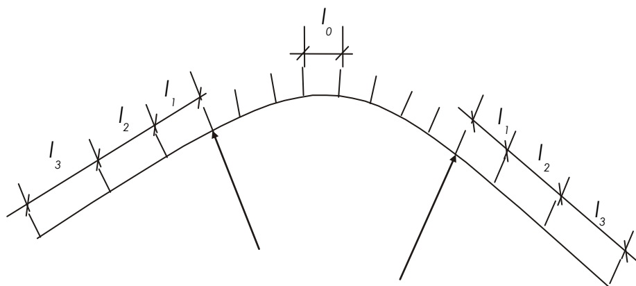
88-rasm Bo'ylama kesimdagi egrilikda va undan oldindagi yo'l uchastkalarida yo'naltiruvchi ustunchalarni joylashtirish.
