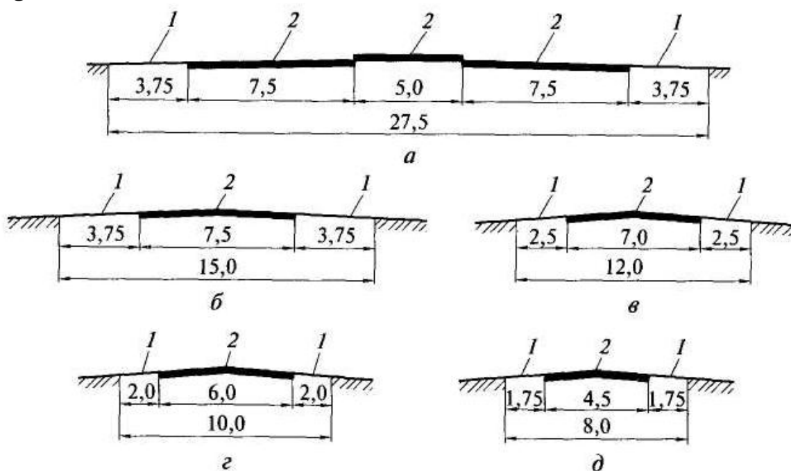
53-rasm. Avtomobil yo'llari andozaviy ko'ndalang kesimlari (o'lchamlar metrda berilgan):
