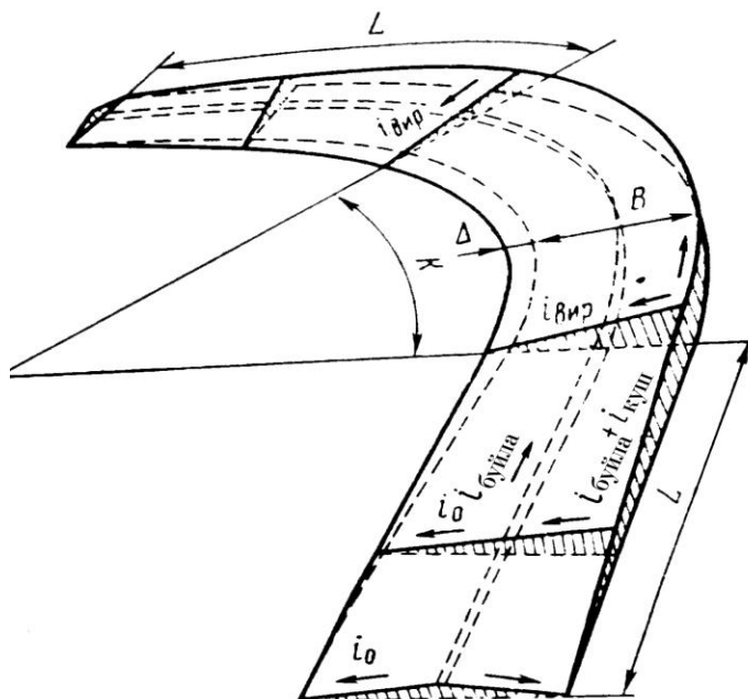
49-rasm. Yo'lining doiraviy egri qismida virajning chiqarish sxemasi.
