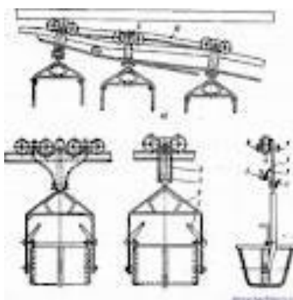
29-rasm. Arqon yo'llari konstruksiyalari
