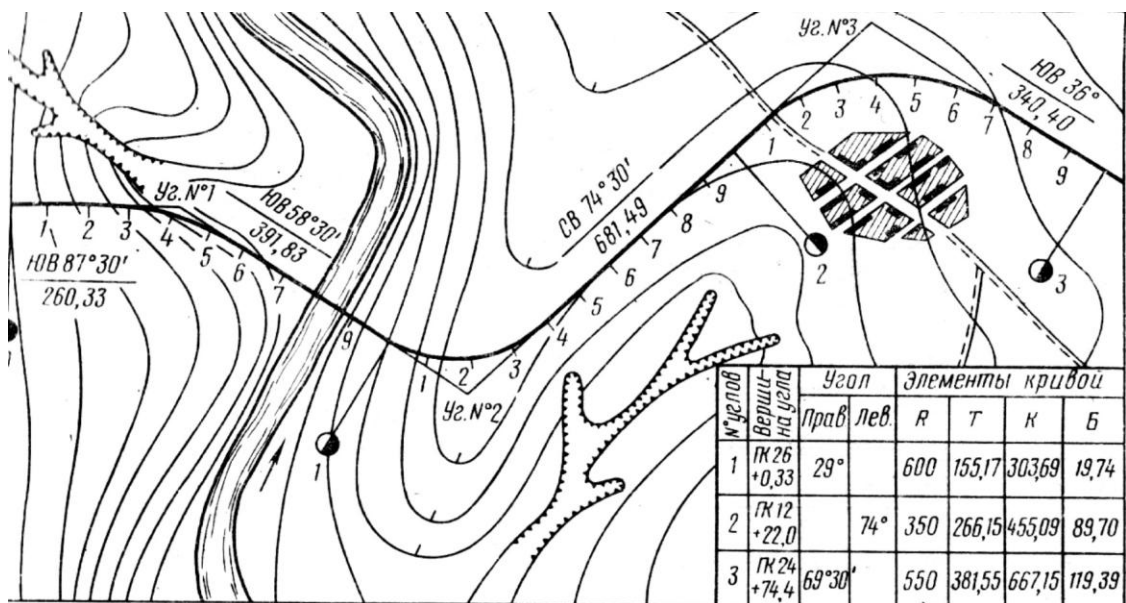
42-rasm. Yo'l o'qi rejasi ko'rinishi
