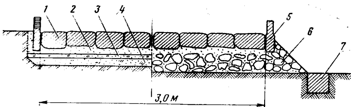
2-Rasm. Yo'l to'shamasi kundalang kesimi.
