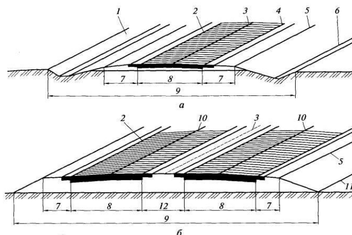
45-rasm. Avtomobil yo'li ko'ndalang kesimi
