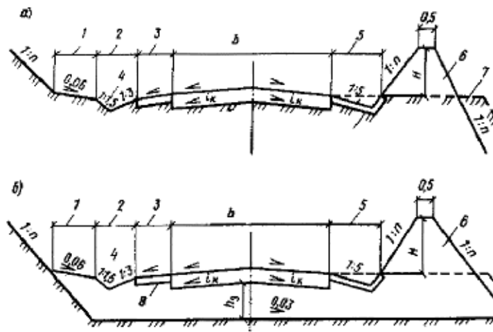
25-rasm. Kon yo'llari yo'l poyi tuzilmasi
