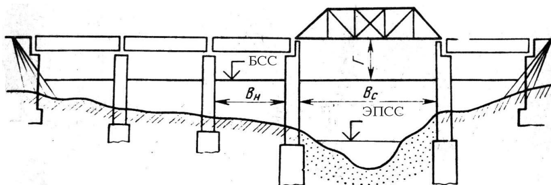
61-rasm. Ko'priknı prolyotlarga bo'lish va kema qatnashi uchun prolyotlar ajratish
