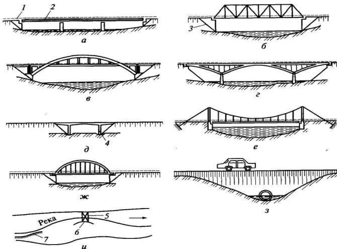
57-rasm. Avtomobil yo'llaridagi sun'iy inshootlar:
