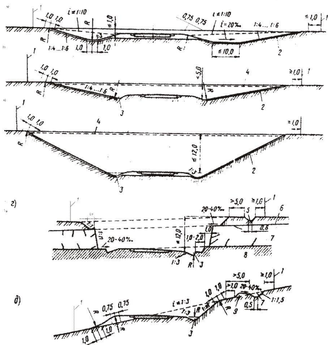
55-rasm. O'ymalardagi yo'l poyining ko'ndalang kesimi:
