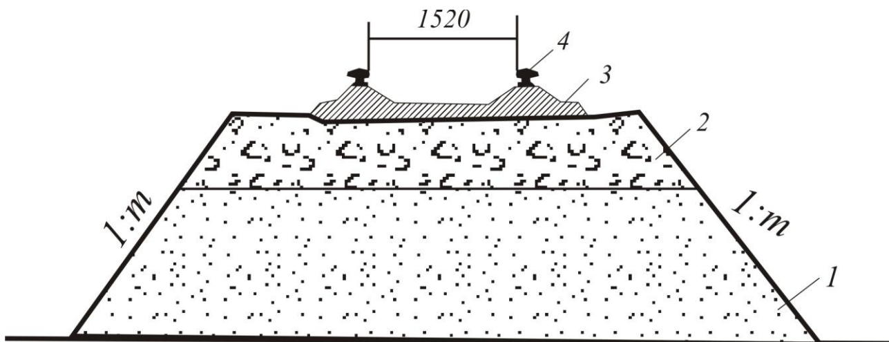
5-rasm. Temir yo'l poyining ko'ndalang kesimi. 1 - yo'l poyi (er tushamasi), 2 - balpasst prizma, 3 – shpal, 4 - pulat rels.
