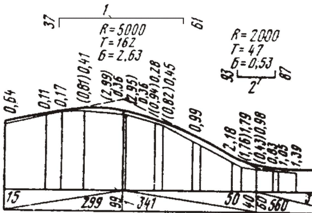
51-rasm. Yo'lining bo'ylama kesimi elementlari (qavariq va botiq egrilar)
