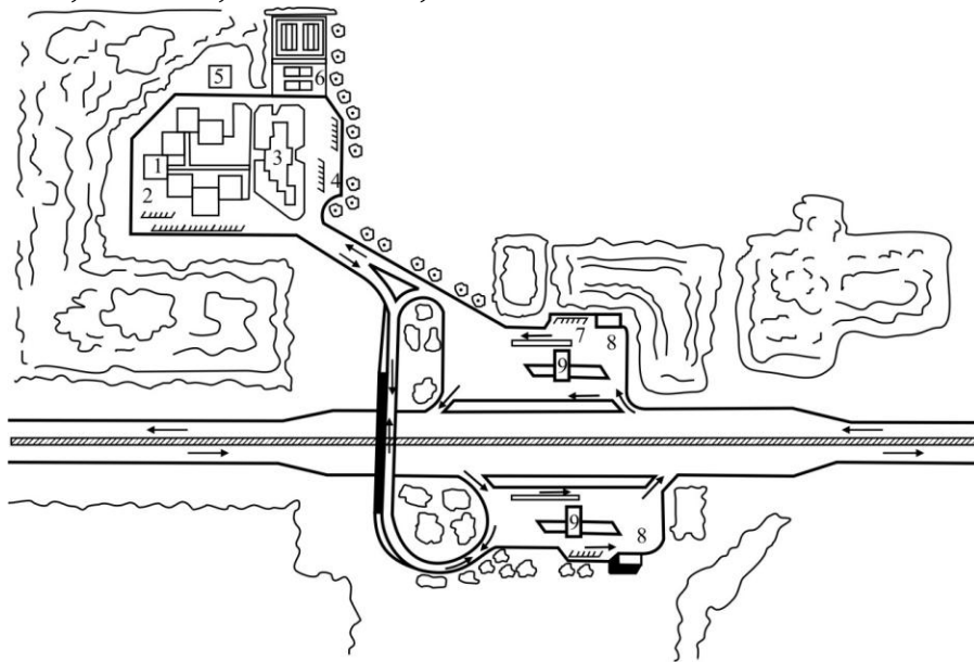
70– rasm. Avtomagistrallarda xizmat ko'rsatish majmualari namunalari:
