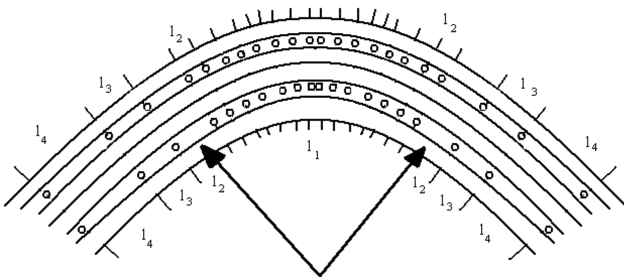
89-rasm. Rejadagi egrilikda yo'naltiruvchi ustunchalarni joylashtirish
