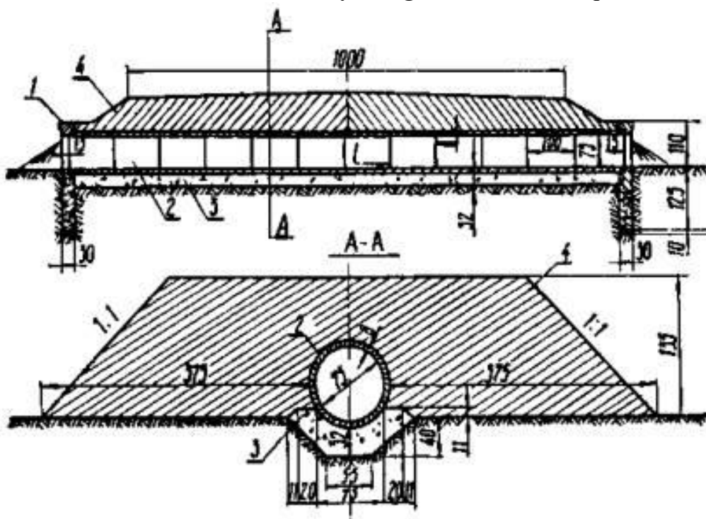
58-rasm. Quvur sxemasi:
