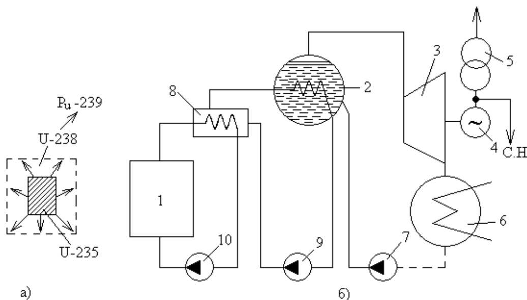
3-rasm. BN tipidagi reaktorlari AES ning printsipl sxemasi.
