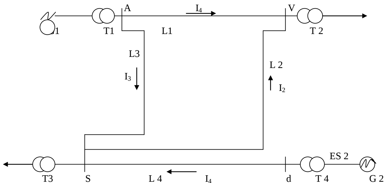
1 - rasm. Elektr energetika tizimining printsipial sxemasi.
