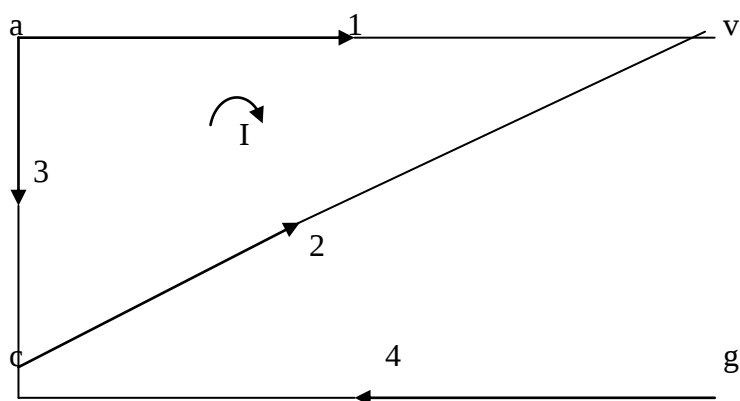
2 – rasm. Elektr energetika tizimining bog'langan yo'naltirilgan grafi.
