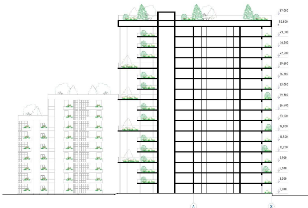
Рис. 3.12. Разрез 1-1. Жилой дом №2.
