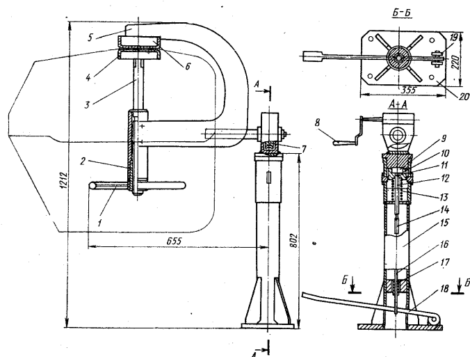
3.-rasm. Avtomobil qanotlarini ta'mirlash va to'g'rilash stendi
