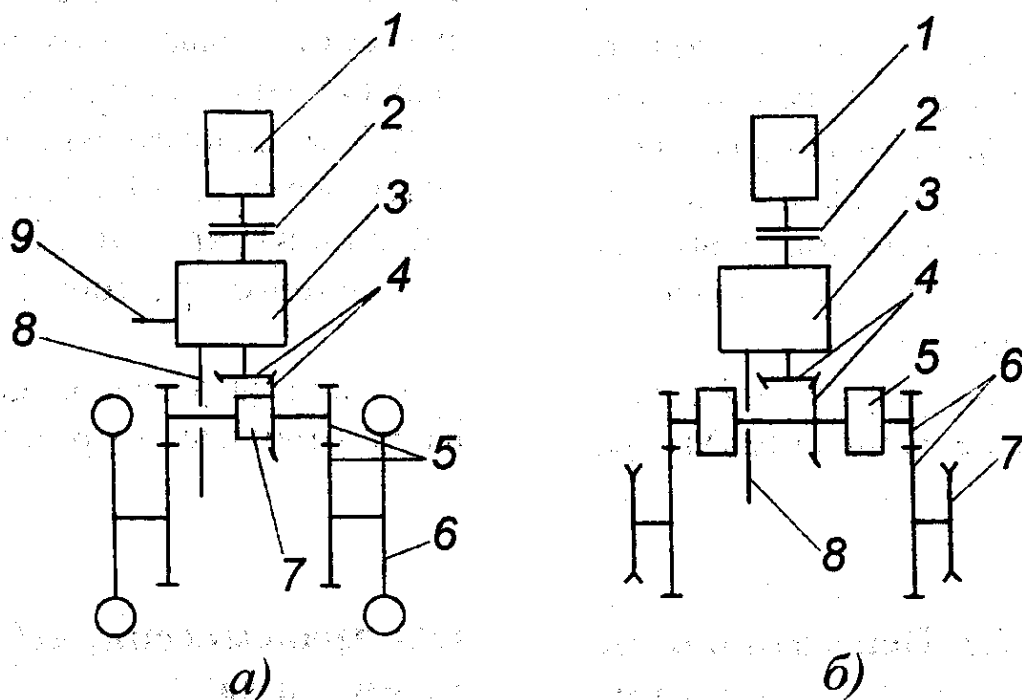
1.4-расм. Ғилдиракли (а) ва занжирли (б) тракторларнинг трансмиссияларини тузилиши: а) 1-двигател; 2-илашиш муфтаси; 3-узатмалар қутиси; 4-бош узатма; 5-охириги узатма; 6-етакловчи ғилдираклар;
