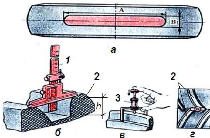
2-расм. Тупроқилгичнинг ейилиш даражасини аниқлаш: а ва г - ўлчаш жойлари; б-штанген-чуқурўлчагич билан ўлчаш; в – мослама ёрдамида ўлчаш: 1-штанген-чуқурўлчагич; 2-тупроқилгич; 3- мослама.
