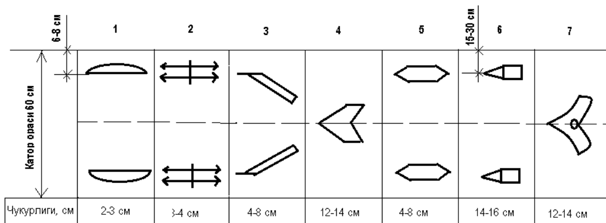
2.17-расм. Култиваторнинг ишчи қисмлари ва уларни ишлов бериш чуқурлиги : 1-лаппак (диск); 2-юлдузча; 3-пичок; 4-чукур юмшатгич; 5-панжа-юмшатгич; 6-ўғит солгич; 7-эгат олгич
