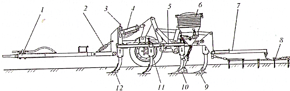
2.8-расм. ЧКУ-4А чизел-культиваторнинг тузилиши:
