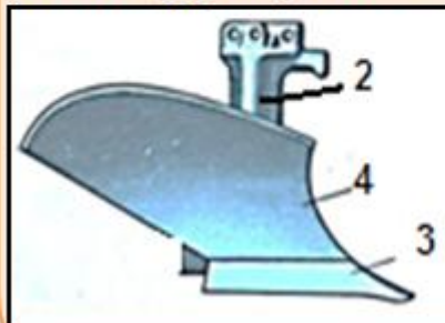
1-чимқарқар; 2-корпус; 3-лемех; 4-ағдаргич
