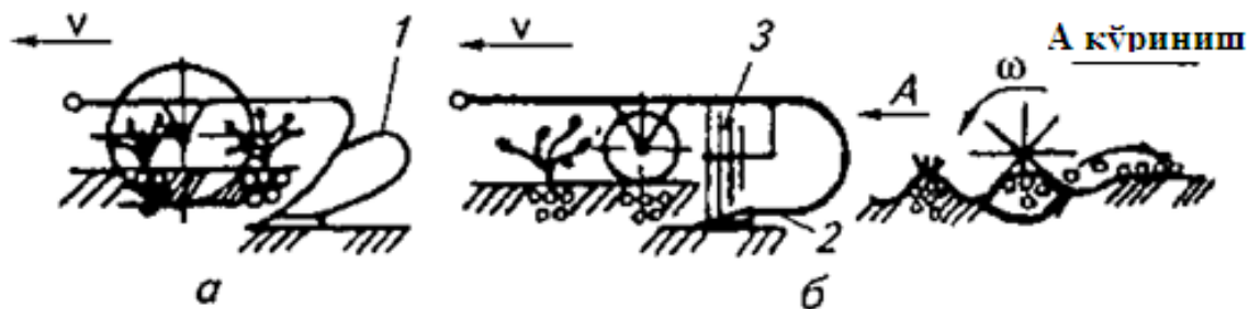
2.33- рasm. Картошка ковлагичлар турлари:
