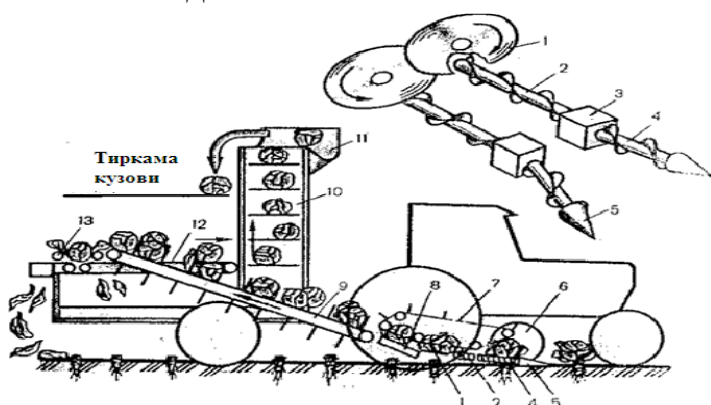
2.37-расм. МСК-1 карам йиғиш машинасининг тузилиши ва иш жараёни: 1-дискли пичоқ; 2,4-шнеклар; 3-редуктор; 5-конус; 6-ғилдирак; 7-транспортёр; 8,11-шнеклар; 9,10-транс- портёрлар; 12-саралаш столи; 13-барг ажратгич.
