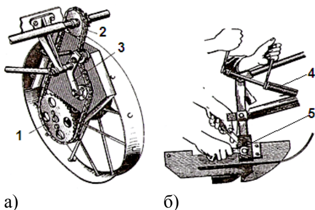
2.13-расм. Сеялкани созлаш: 1- катта юлдузча; 2-кичик юлдузча; 3-тарангловчи курилма; 4- тарангловчи пружина; 6-сирпангич.
