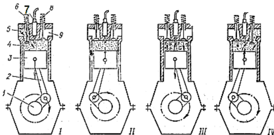
4-расм: Тўрт тактли дизел двигателининг ишлаш жараёни:
