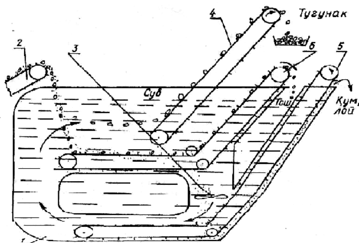
3.11-рasm: Картошка тугунакларини зичлиги бўйича суспензияда тош-кесаклардан ажратиш машинаси: 1-идиш; 2-транспортер; 3-винтсимон сув ҳайдагич; 4,5,6-транспортерлар
