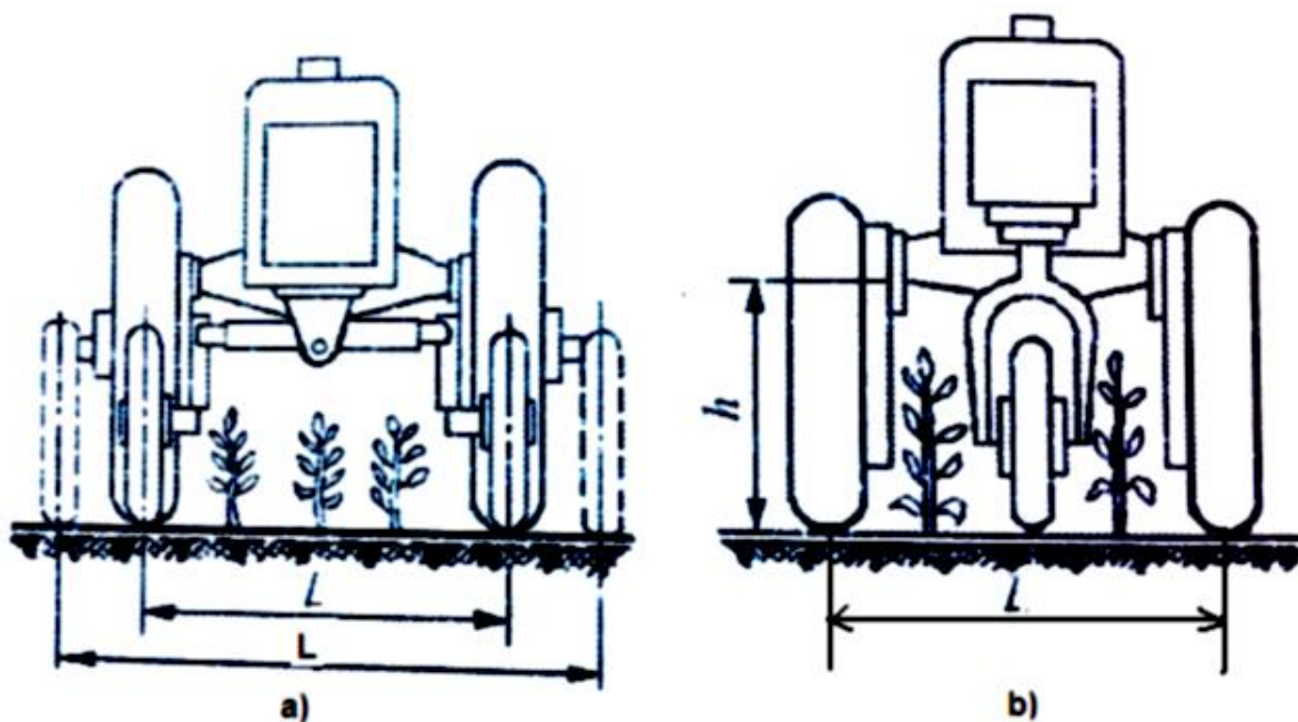
1.7-расм. Ғилдиракли тракторлар коляси ( L ) ва агротехника масофаси ( h )
