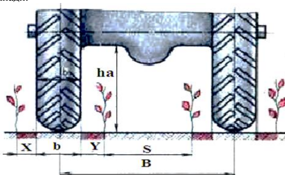
1-расм. Ғилдиракли тракторнинг ўтувчанлик кўрсаткичлари: X –ташқи ҳимоя йўлаги; Y -ички ҳимоя йўлаги; S - қатор ораси; b -трактор шинасининг кенглиги; B - трактор ғилдиракларининг оралиғи; h_a – агротехник масофа
