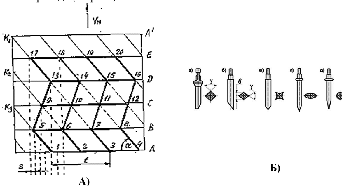
10-расм. Тирма тишларининг ўрнатиш схемаси (А) ва уларнинг кўндаланг кесимларига қараб турланиши (Б):
