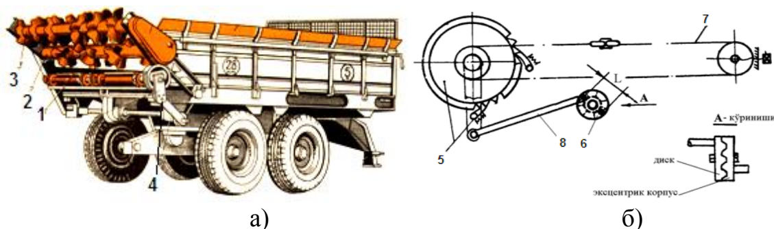
2.3-расм. РОУ-6 русумли маҳаллий ўғит сочиш машинасининг тузилиши (а) ва уни ўғит сочишга созлаш тартиби (б):
