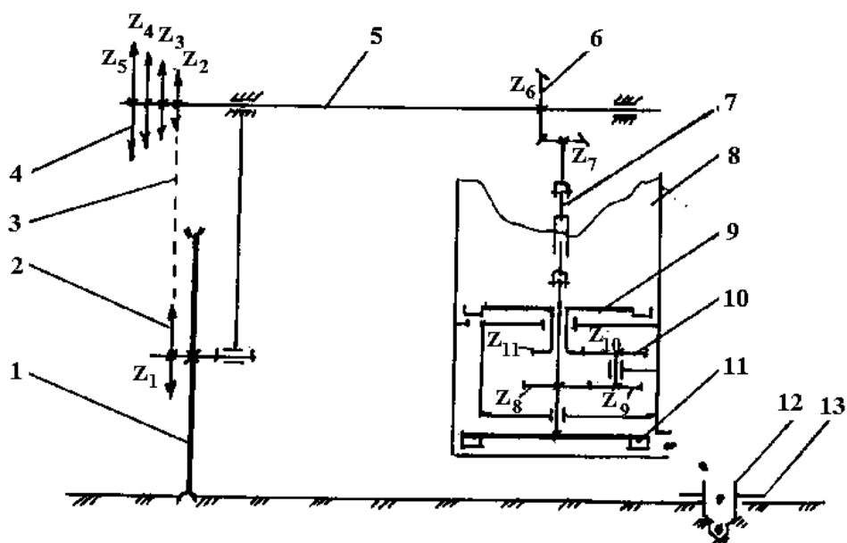
13 – расм. Чигит сеялкаси дисксимон микдорлагичига харакат узатиш схемаси.
