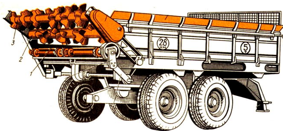
2.10-расм. РОУ-6маҳаллий ўғит сепишмашинаси:
