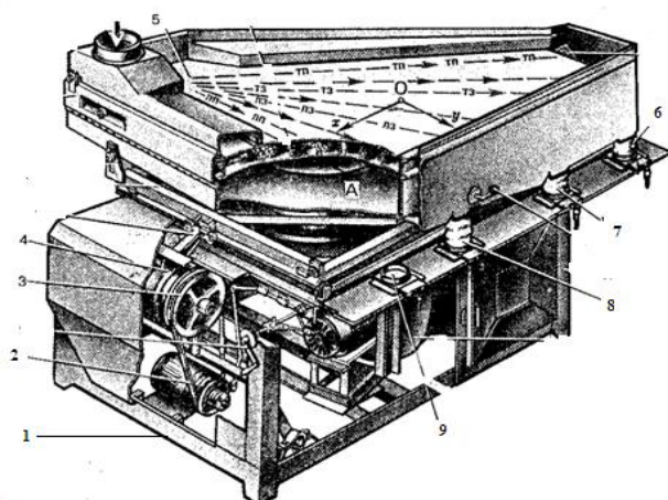
2.48-расм. ПСС-2,5В пневмосаралагичнинг тузилиши ва иш жараёни: 1-рама; 2-электродвигатель; 3-харакатузатиш механизми; 4-вентилятор; 5- тебранувчи дека; 6,7,8 ва 9- чиқариш тешиклари.
