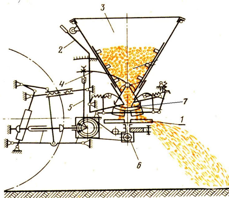
2.9-расм. НРУ-0,5 дисклиўғит сочгич схемаси:
