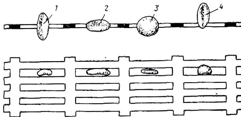
2.45-расм. Донларни чўзинчоқ тўртбурчак шаклдаги ғалвирларда ажратиш: 1,2 ва 3-қалинлиги ғалвир кўзи энидан кичик донлар;4- қалинлиги ғалвир кўзи энидан катта дон.
