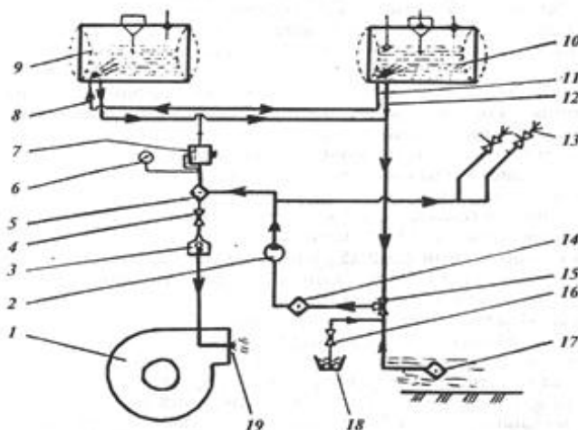
2.26-расм. Пуркагичнинг технологик иш жараёни (белгилар матнда кўрсатилган)
