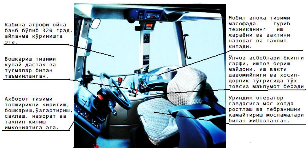
18-расм. Клаас фирмасининг ARES 816 трактори кабинасида бошқарув ва ёрдамчи қурилмаларни жойлаштириш.
