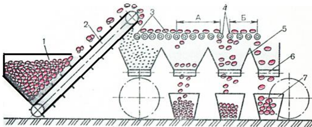
3.10-расм. Роликли тозалагичнинг тузилиши ва иш жараёни: 1-кабул бункери; 2- кия транспортер; 3-майда чиқиндиларни ажратувчи роликлар; 4-туганак ажратувчи роликлар; 5-туганак йиғгичлар; 6-лентали транспортерлар; 7-контейнерлар.
