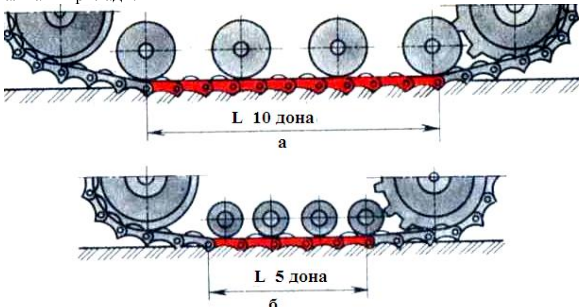
3-расм. Трактор занжирларининг ҳолатини аниқлаш: а- ДТ-75М трактори учун; б- Т-70С трактори учун; L -занжир звеноларининг узунлиги
