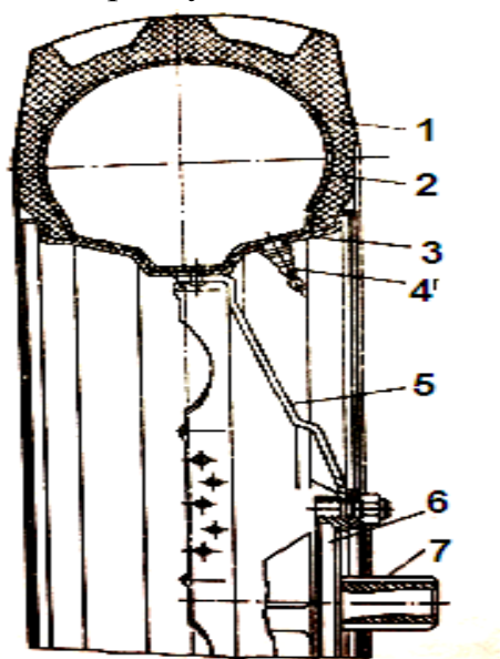
1.6-расм. Ғилдиракли тракторнинг етакчи ғилдираги: 1- покришка; 2- камера; 3- тўғин; 4-вентил; 5- диск; 6-губчак; 7- ярим ўқ
