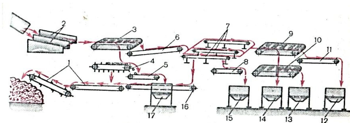
2.52-расм. Картошка саралагич пунктинингтехнологик жараёни ва машиналари: 1, 5, 6, 8, 11 ва 16- транспортерлар; 2- қабул қилиш бункери; 3- чиқинди тозалагич; 4-нинасимон саралагич; 7-қўлда тозалаш столлари; 9 ва 10- ғалвирли саралагич; 12,13, 14, 15 ва 17- йиғич-бункерлар.
