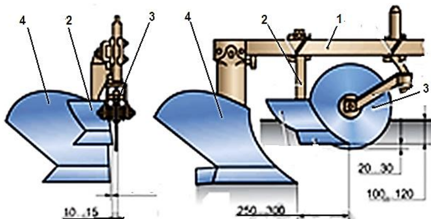
2.2-расм. Плугнинг асосий қисмлари ва уларни ростлаш ўлчамлари: 1-рама; 2- чимқирқар; 3- диски пичоқ; 4-асосий корпус
