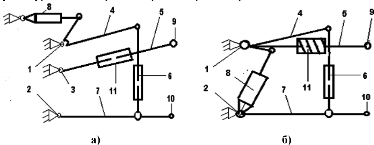
1.11-расм. Уч (а) ва икки (б) нуқтали осиш қурилмаларининг тузилиши:
