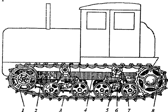
1.6-расм. Ўрмаловчи занжирли тракторнинг юриш қисми: 1- тарангловчи гилдирак; 2- таранглаш мосламаси; 3- ўрмаловчи занжир; 4- трактор рамаси; 5- тутқичролик; 6-каретка; 7- таянч гилдирак; 8-етакчи юлдузча.
