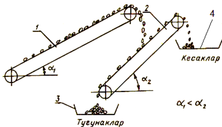
3.12-рasm, Ишқаланиш коэффициенти бўйича тугунакларни тош ва кесаклардан тозалаш мосмаси: 1-узатувчи транспортер; 2-сараловчи транспортер; 3- тугунаклар учун идиш; 4- қум, тош ва кесаклар учун идиш
