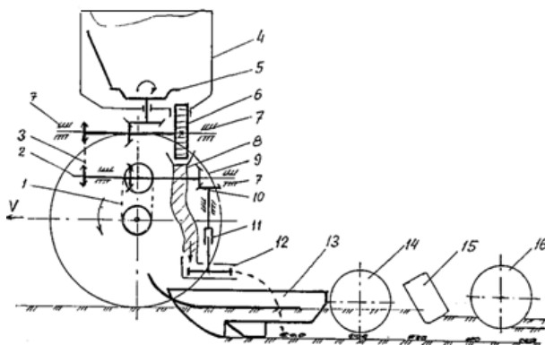
2.12-рaсм. Сеялканинг технологикиш жараёни: 1- занжирлиҳаракат узатмаси; 2-вал, 3- занжирли узатма, 4-бункер, 5-тўзиткич, 6-миқдорлагич, 8-уруғ ўтказгич, 9- юритувчи ғилдирак, 10 - конуссимон шестерня, 11-телес-копик вал, 12- тўдалагич, 13-сирпанғичли экич, 14- ботирувчи ғилдиракча, 15-кўмгич, 16- шаббалагич.
