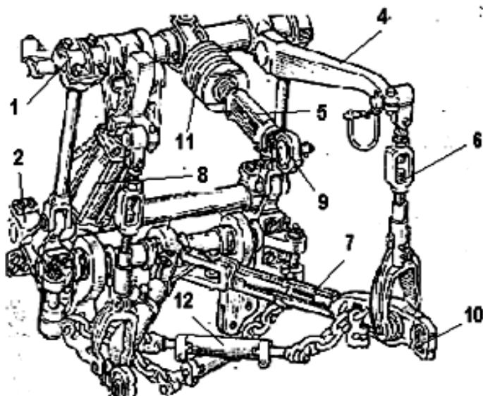
1.15-расм. Икки нуқтали осиш қурилмасини тузилиши:
