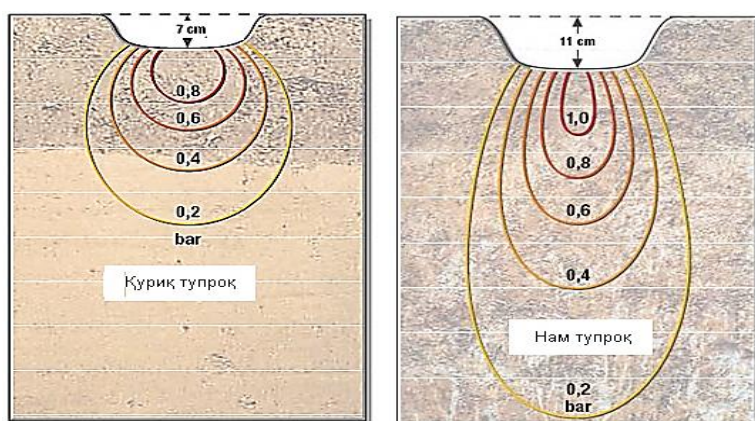
1.7-расм. Трактор ғилдирагининг курик (а) ванам (б) тупроқларни зичлаш диаграммаси
