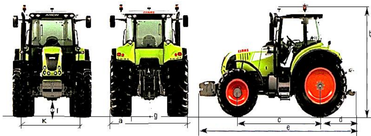
1-17-расм. Тракторнинг асосий ўлчамлари: e-узунлиги; b-баландлиги; g-эни; c- базаси; d-кинематик узунлиги; i-агротирқиш; k- колеяси; a- шина кенглиги.
