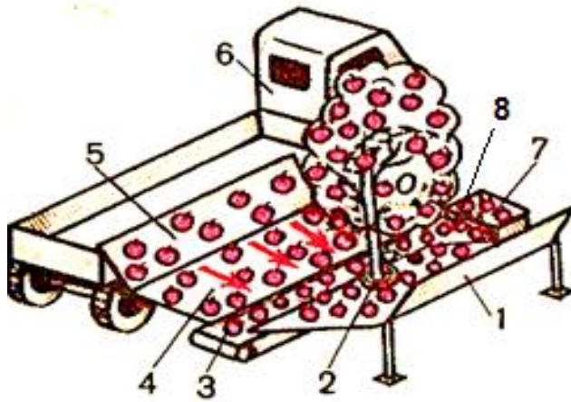
3.5-расм. Мева йиғиш машинасининг ( ВУМ-15А) тузилиши ва иш жараёни: 1,4- илгичлар; 2-тебратгич; 3-транспортёр; 5-экран; 6- шасси; 7-контейнер; 8- вентилятор.
