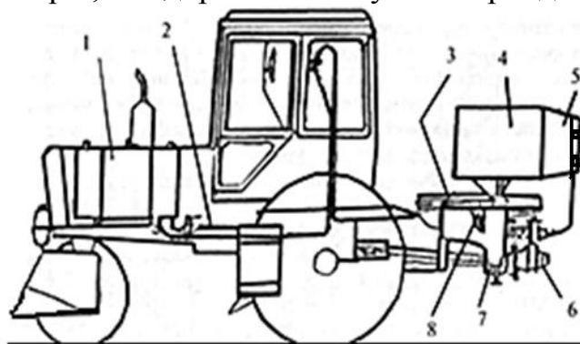
19-расм. ОВХ-600 пуркагичининг умумий тузилиши: 1-суюқлик идиши; 2-таъминлаш тизими; 3-ҳаракат узатиш механизми; 4-вентильатор; 5-сопло; 6-созлагич; 7- редуктор; 8-ростлагич; 9-учликлар.
