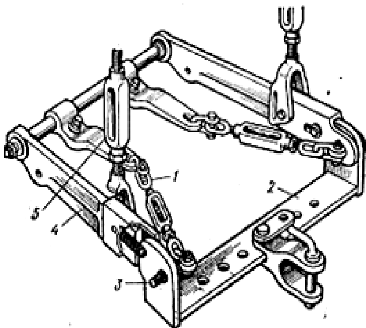
1.13-рasm. Ўрнатиш қурилмасига шатаклагич ўрнатиш: 1-қўзғатмаслик тортқилари; 2-шатаклагич; 3-маҳкамлагич; 4-пастки тортқилар, 5-тик кашаклар.
