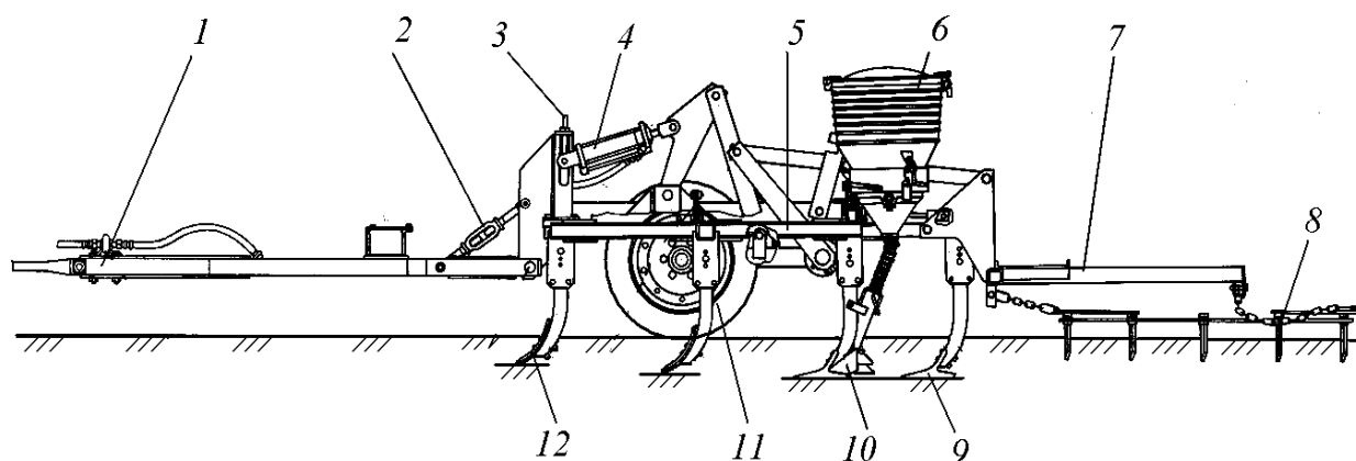
2.7-расм. ЧКУ-4А чизел-культиваторинг тузилиши:
