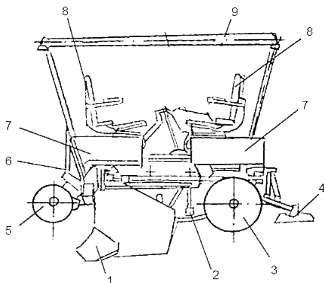
2.18-расм. ССН-1 кўчат ўтказиш машинасининг тузилиши: 1-эгат олгич; 2-экиш аппарати; 3-зичловчи ғалтак; 4-тупроқ кўмгич; 5-таянч ғилдирак; 6-рама; 7-кўчат яшиги; 8-ўриндик; 9-соёбон
