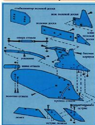
Ағдаргичнинг асосий қисмлари
