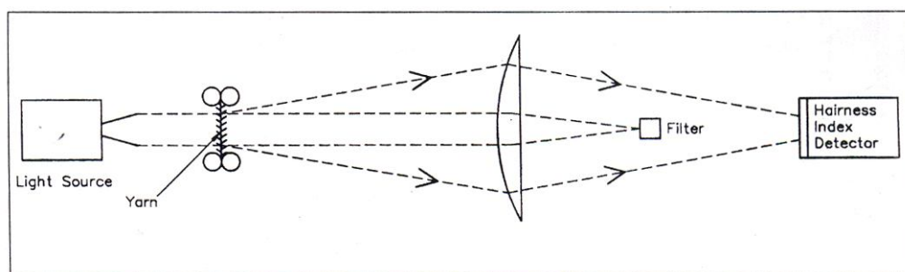
5-сүўрет. Түклилик индексин өлшеудің оптикалық принципінің схемасы.
