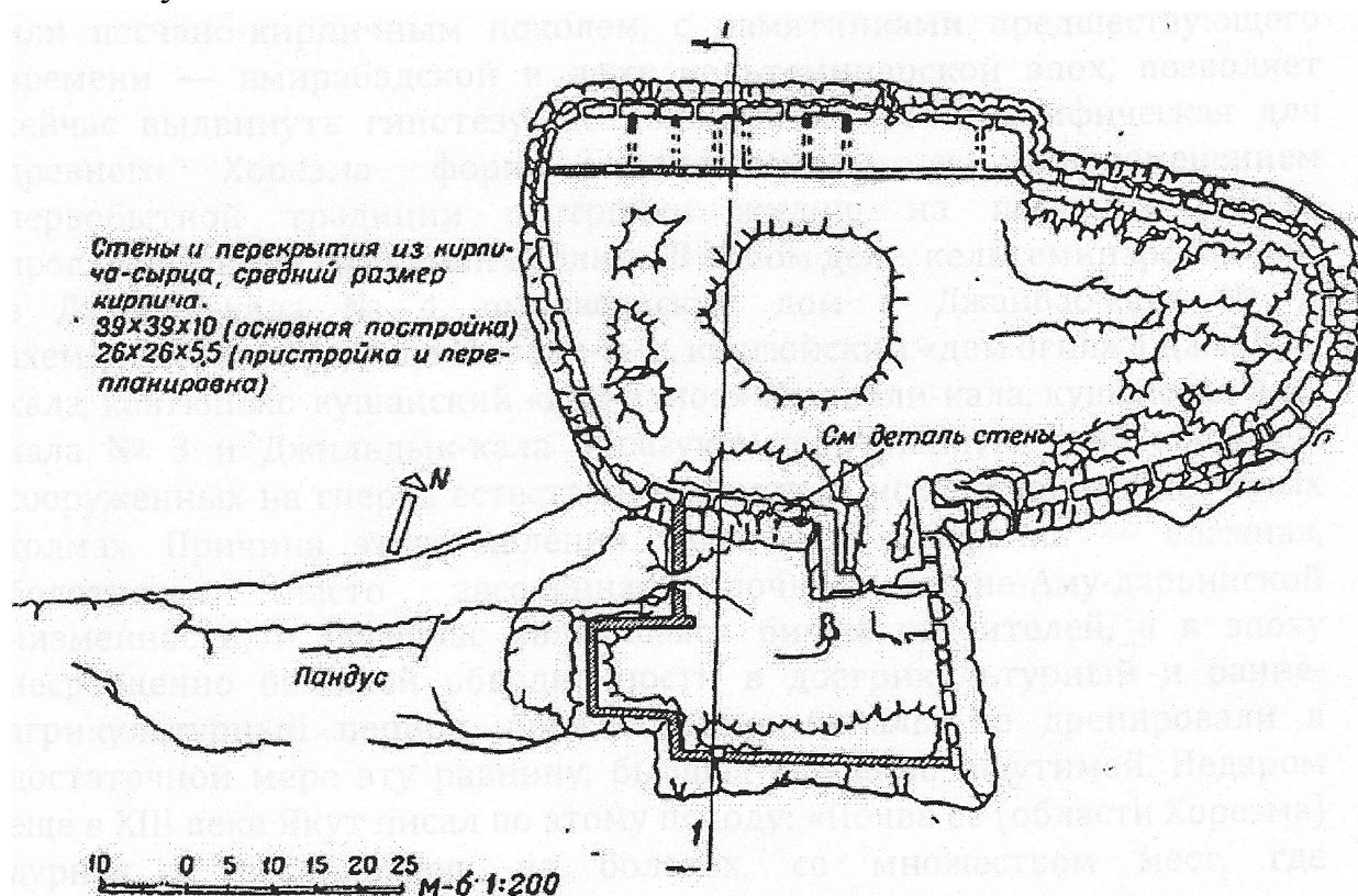
СҮЎрет 42. Аяз қала Қ2 План. В. Пилявскийдің обмери.
