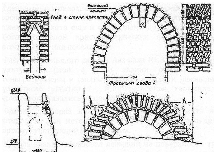
СҮҮрет 41. Аяз қала Қ1 Деталлар. Арх. В. Пилявский обмеры.
