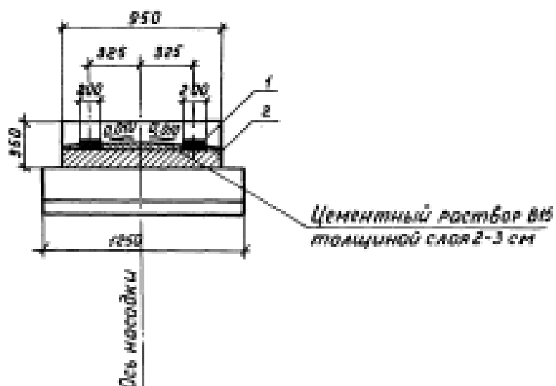
Разрез 1-1
