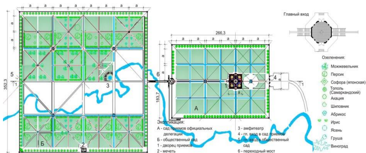
15-расм. Самарқанддаги Амир Темур бунёд этган - «Боғи Нақшижаҳон» ни Чорбоғ услубида қайта тиклаш лойиҳаси. Дипломант Садыкова С.Н, раҳбари А. С. Уралов (СамДАҚИ) 2005 й.
