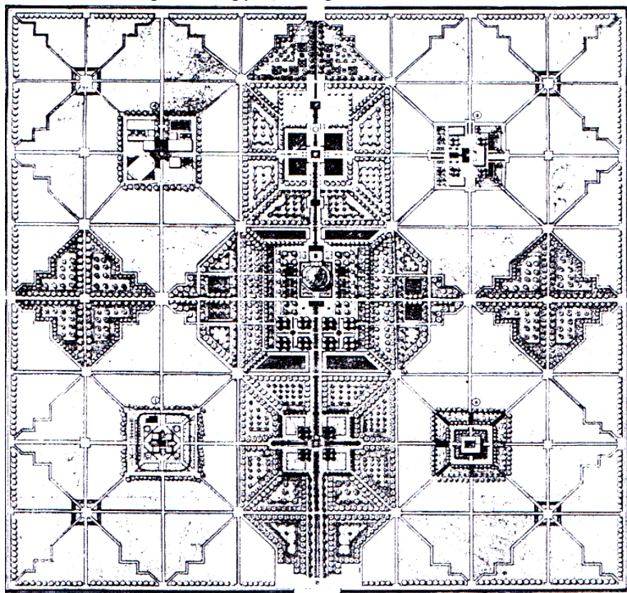
13-расм. Чорбоғнинг А.С.Уралов, К.Ж.Рахимов, Н.В.Дробченколар яратган реконструкцияси лойихаси. 2003 й.
