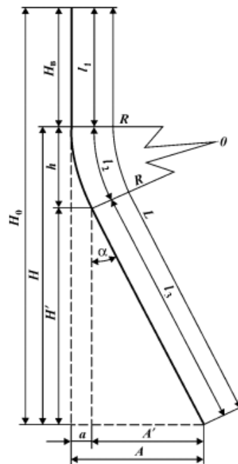
Рис. 9.6. Вертикальная проекция направленной скважины тангенциального (1-го) типа
