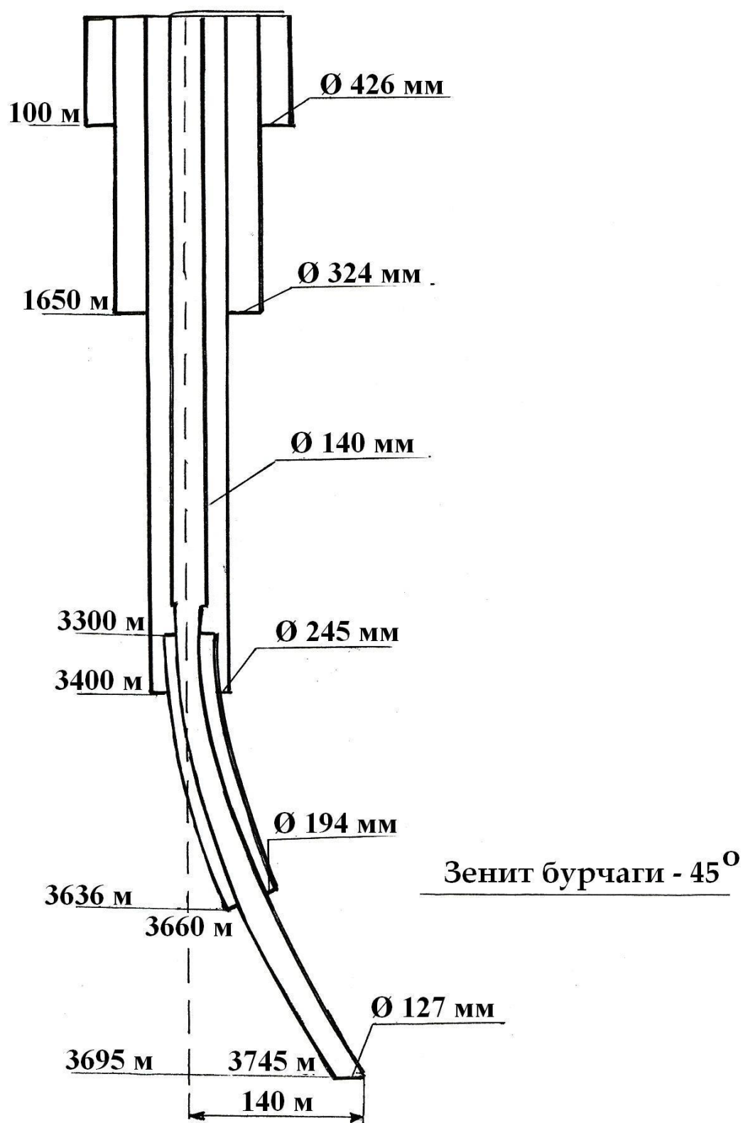
-расм. Шимолий Шўртан конида қудуқнинг қия профили
