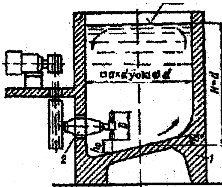
2-расм. 1 - ҳавза; 2 - парракли аралаштирувчи қурилма.
