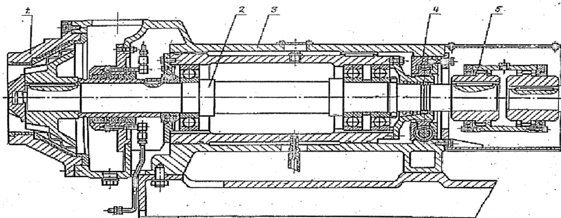
8-расм. МП-00 маркали пульсацияловчи тегирмон
