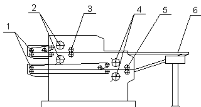
20-расм. Кўндаланг қирқиш дастгоҳи:
