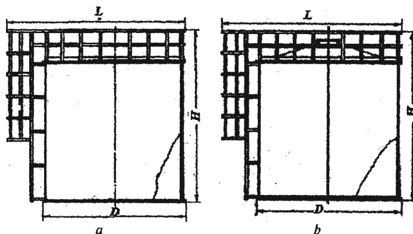
4-расм. Текис (а) ва конус шаклидаги (б) қопқоқли баклар
