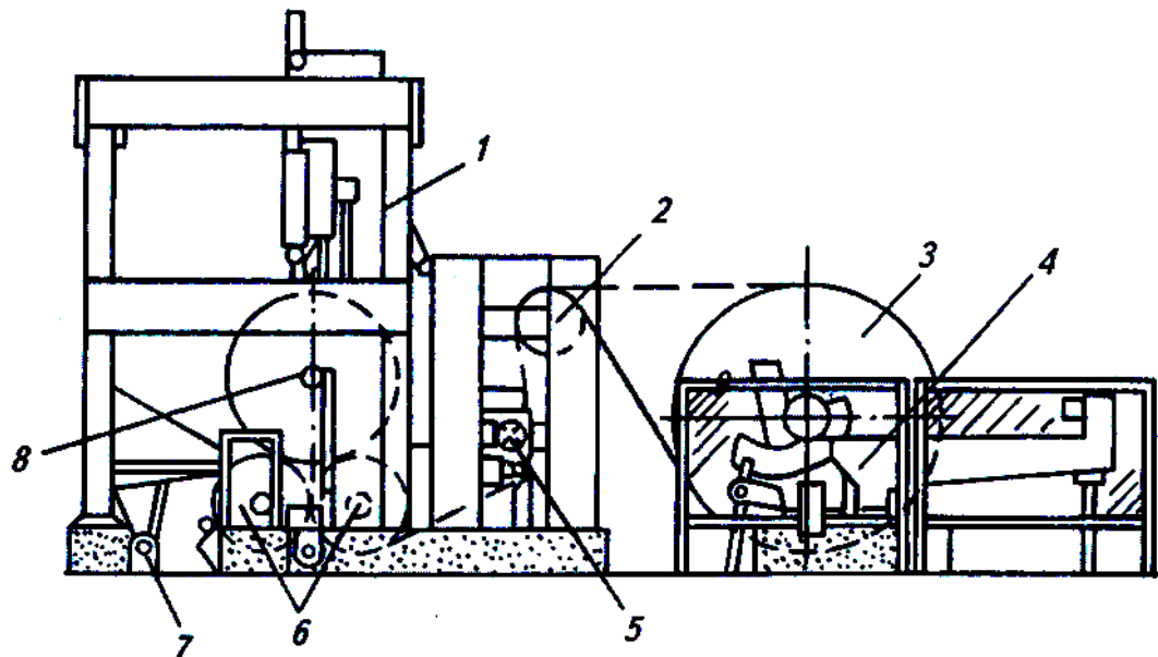
12-расм. Узунасига қирқиш дастгоҳ (полотнони пастдан вертикал узатилганда) схемаси:
