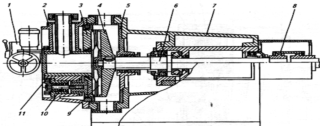
7-расм. МД-14 маркали дискали тегирмон
