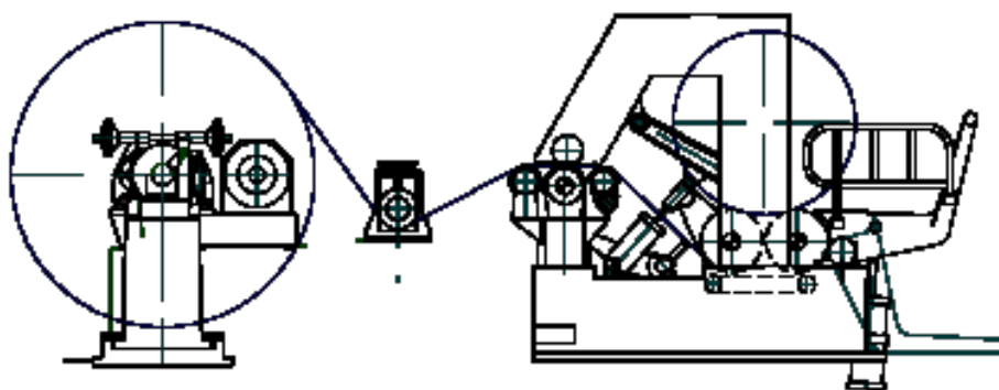
18-расм. C5-201 маркали қоғозни узунасига кесиш дастгоҳининг схемаси.
