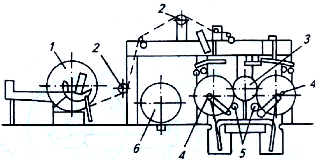
15-расм. Иккиланган узинасига қирқиш дастгоҳ схемаси:
