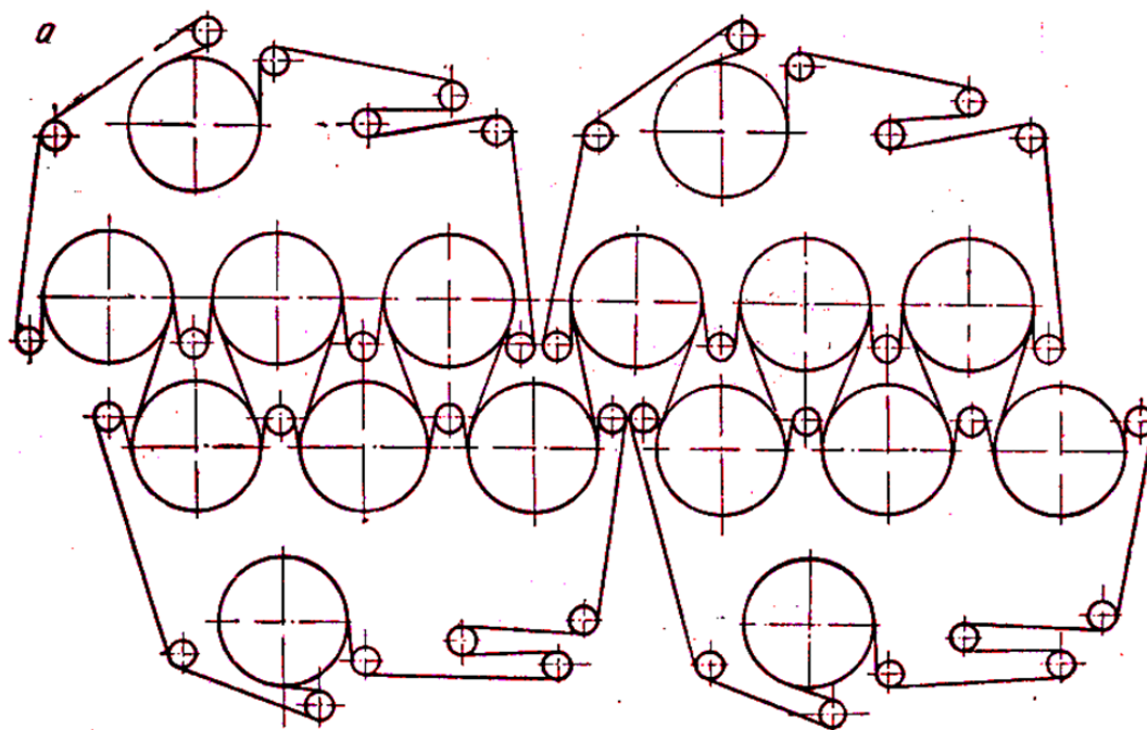
23-расм. Қоғоз қуйиш жихозининг қуритиш қисми
