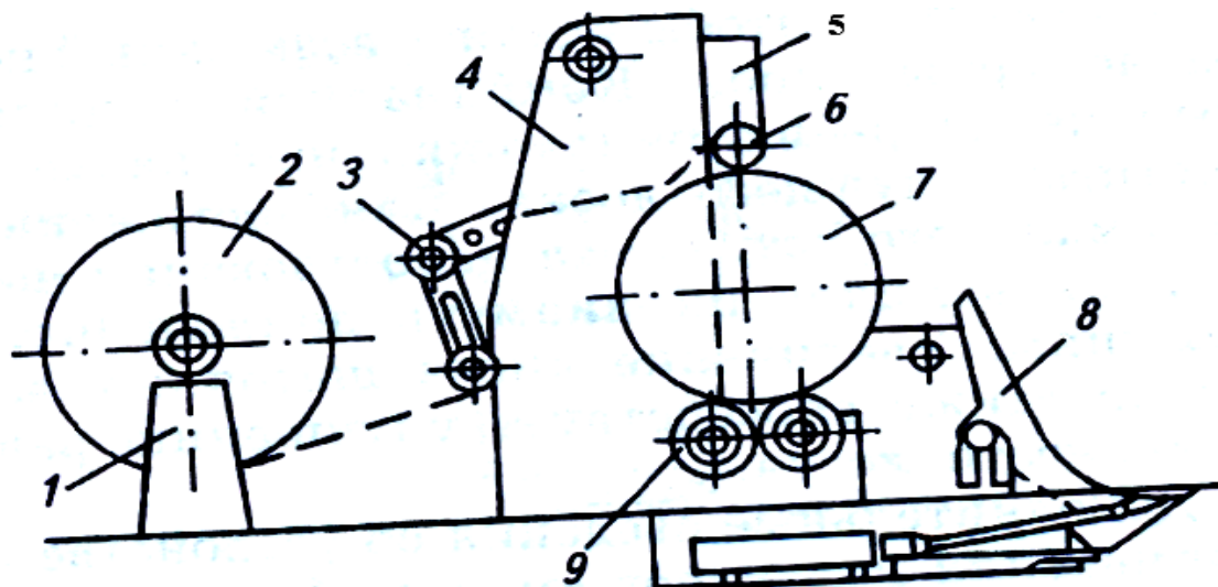
10-расм. Узунасига қирқиш дастгоҳининг (полотнони юқоридан узатилганда) схемаси:
