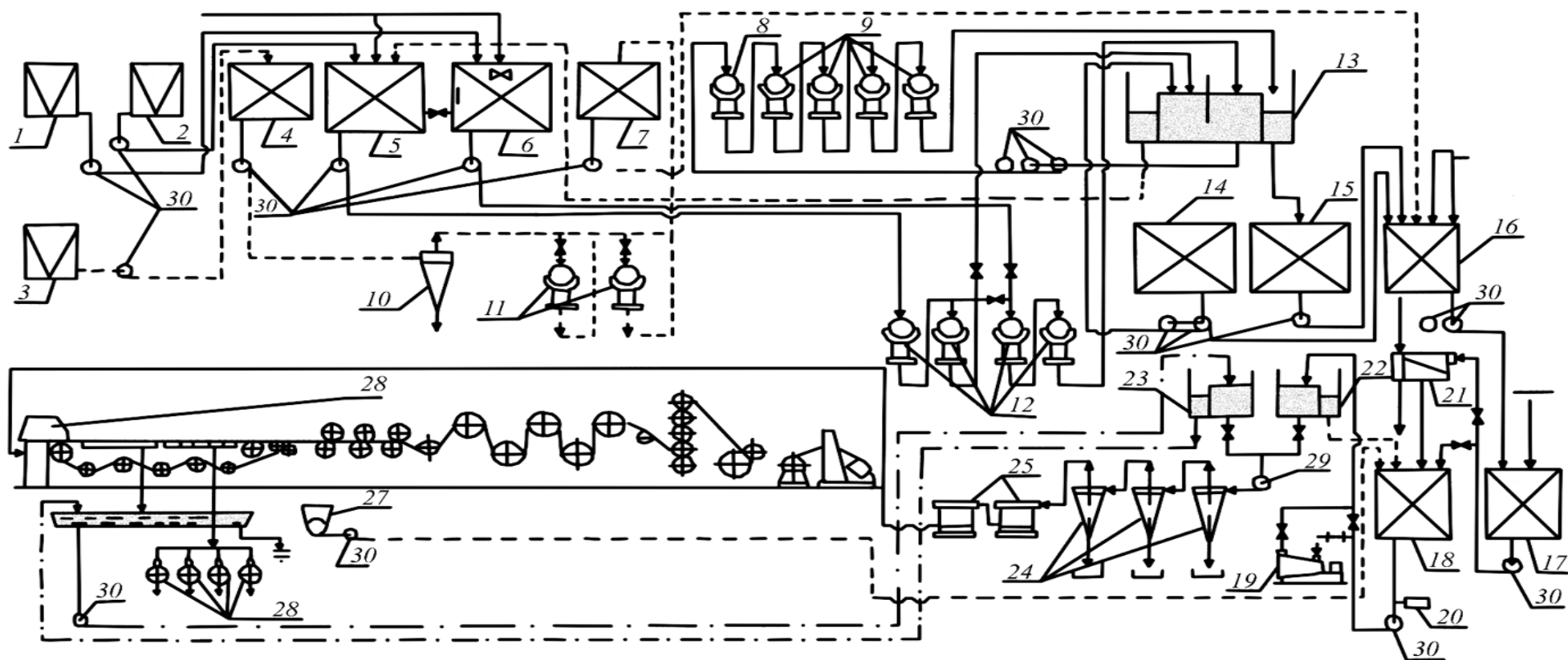
22-расм. Ватман қоғоз ишлаб чиқариш технологиясининг схемаси:
