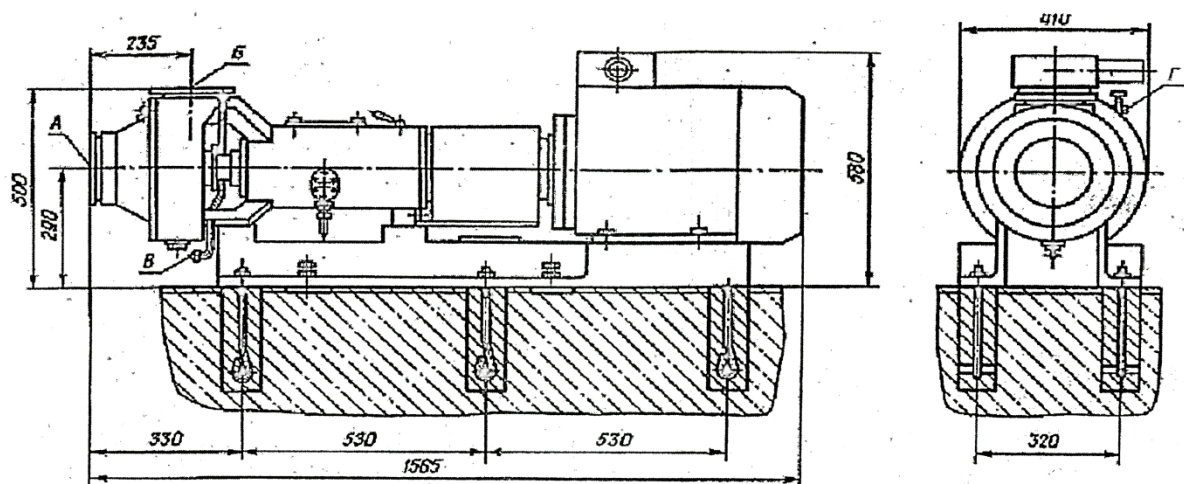
9-расм. МП-00 маркали пульсацияловчи тегирмоннинг чизмаси ва габарит ўлчамлари
