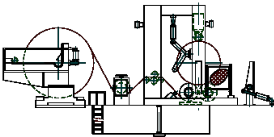
17-расм. C5-303 маркали қоғозни узунасига кесиш станогининг схемаси
