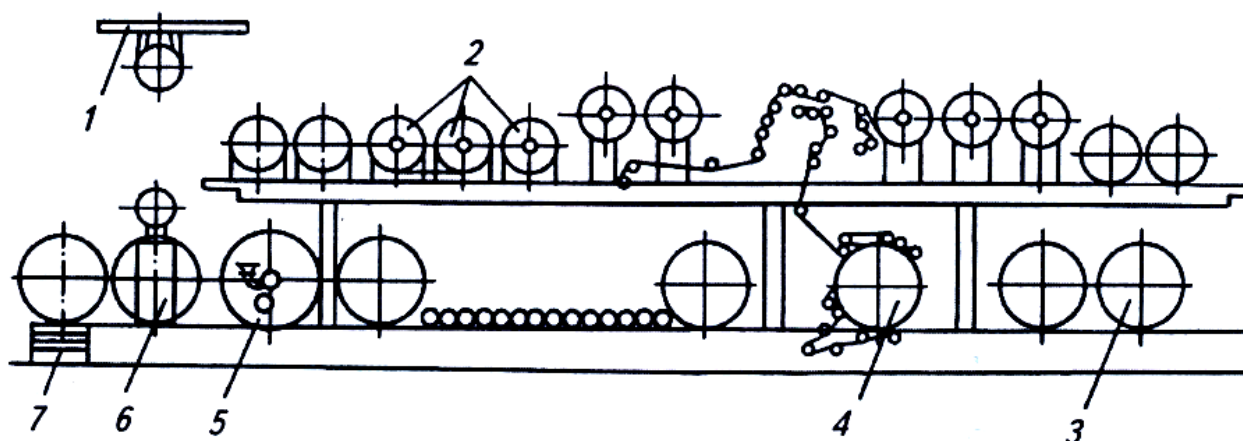
21-расм. Рулон ўрагич линиясининг схемаси:
