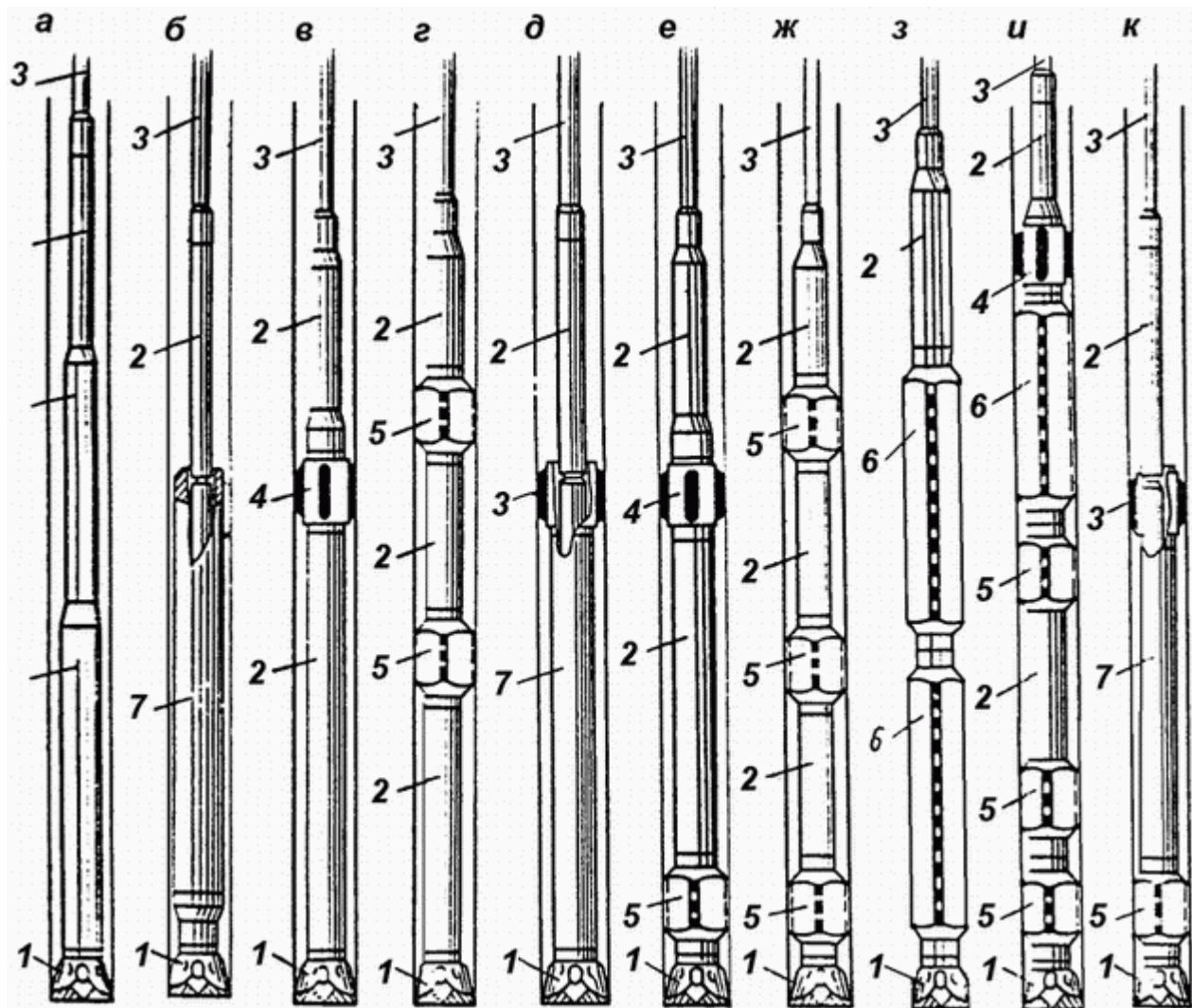
42-rasm. Quduqni qiyshayishiga qarshi kurashish uchun burgʻilash tizmasining ostki qismi jamlamasi.
