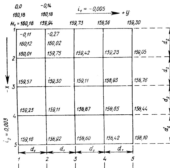
2-расм. қия текислик лойихалашга доир схема
