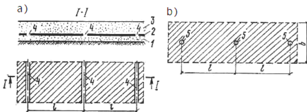
3.12-rasm. Uzluksizligi buzilgan bir qavatli plyonkali ekran; a-uzluksiz tirqishlar ko'rinishida; b-alohida teshiklar ko'rinishida;
