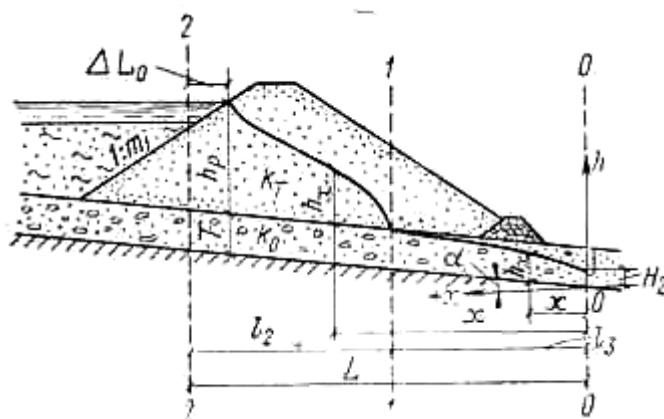
5.5 —rasm. Ekranli lentasimon drenajli to'g'ronni zaminida tish yoki oldida gorizontal ekran bo'lganda filtratsiya hisobi sxemasi.
