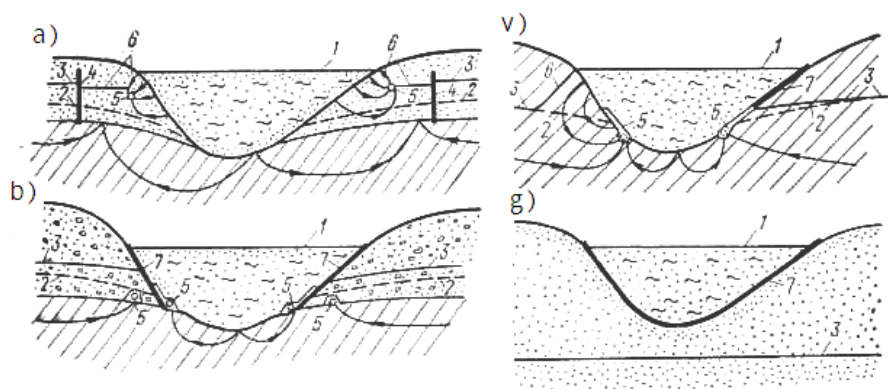
3.2-rasm. Chiqindixona maydonidagi filtratsiyaga qarshi qurilmalar. 1- Chiqindixona loyihadagi yuzasi; 2—mavjud gruntli suvlarni yuzasi; 3-suvlarini ko'tarilish zgri chizig'i; 4—filtratsiyaga qarshi parda; 5-drenalar; 6—depressiya egri chizig'i; 7 —ekranlar.
