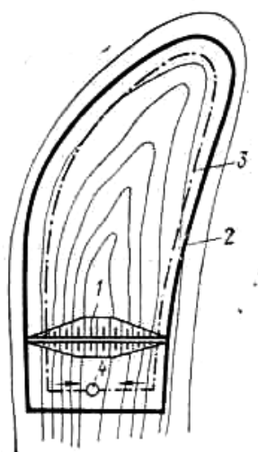
3.3-rasm. Chiqindixonadagi aylanma filtratsiyaga qarshi qurilmani planda joylashishi. 1-to'g'on; 2-filtratsiyaga qarshi parda; 3-aylanma drenaj; 4-nasos stantsiyasi.
