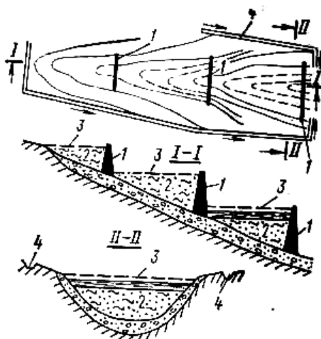
2.4 —rasm. Balka —jdalik tipdagi ko'p pog'onali chiqindixona. 1-to'g'on; 2 — chiqindi-lar to'plami; 3-chn15indixOnani loyihadagi yuzasi; 4—tog' arig'i
