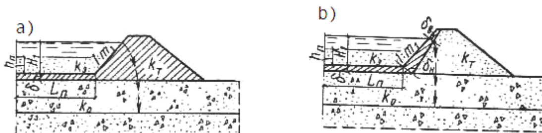
5.11 — rasm. Cheklanmagan qalinlikda suv o'tkazuvchi zamindagi bir qavatli ekranni filtratsiya hisobi sxemasi.
