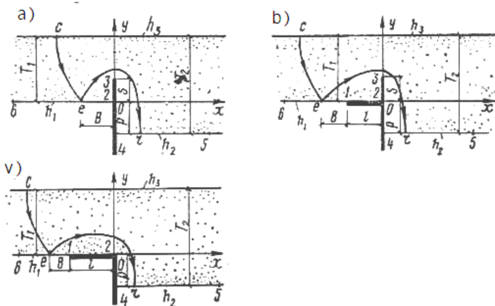
5.9-rasm. To'g'anni qirg'oq bilan tutashgan joyida aylanma filtratsiyani hisoblash sxemasi.
