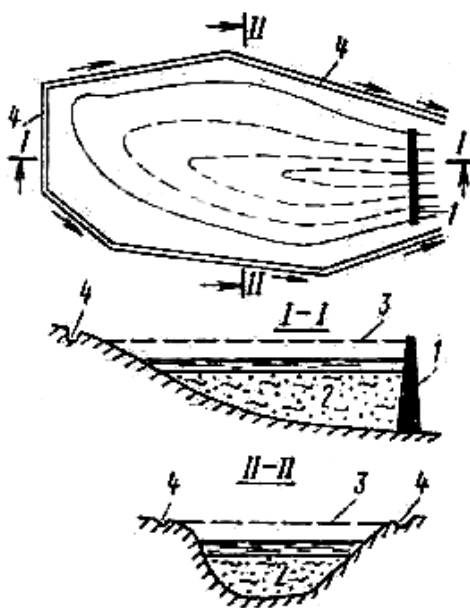
2.3—rasm. Balka—jarlik tipidagi bir pog'onali chiqindixona. 1- to'g'on; 2—chiqindilar to'shmi; 3—chiqindixonani loyihadagi yuzasi; 4-tog' arig'i.
