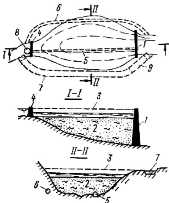
2.9—rasm. Chiqindixonona suv tashlash inshootlarini joylashish sxemasi. 1-to'g'on; 2-chiqindi tplami; Z-chiqindixonani loyihadagi yuzasi; 4-damba; 5,6,7-suv tashlamani tubiagi quvurlar, tunnel va ochiq kanal ko'rinishidagi mumkin bo'lgan variantlari.
