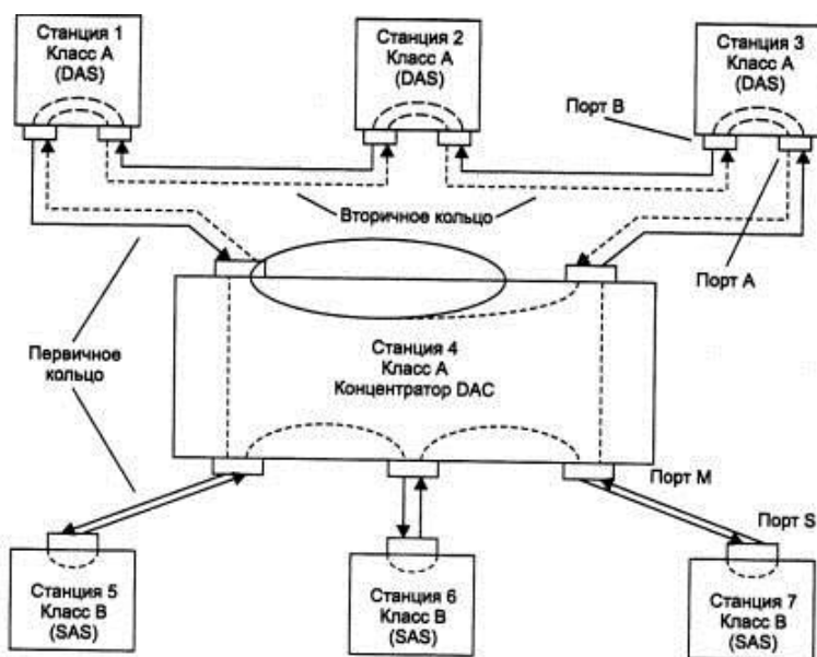
8.2.- расм. Станцияларни FDDI ҳалқаларига уланиши.
