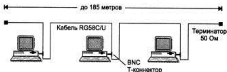
Рис. 4.2. Сеть стандарта 10Base-2.
