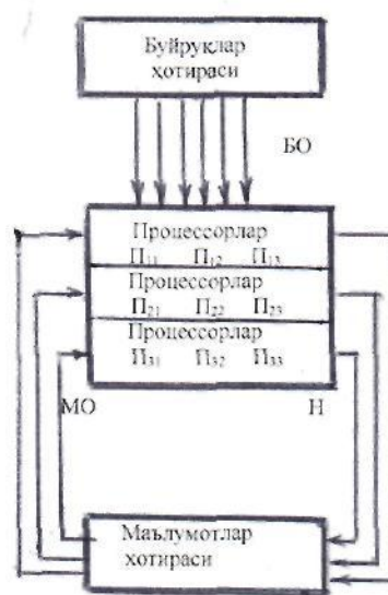
г) MIMD
