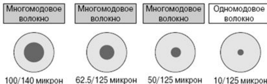
Рис. 2.35. Одномодовое и многомодовое оптические волокна
