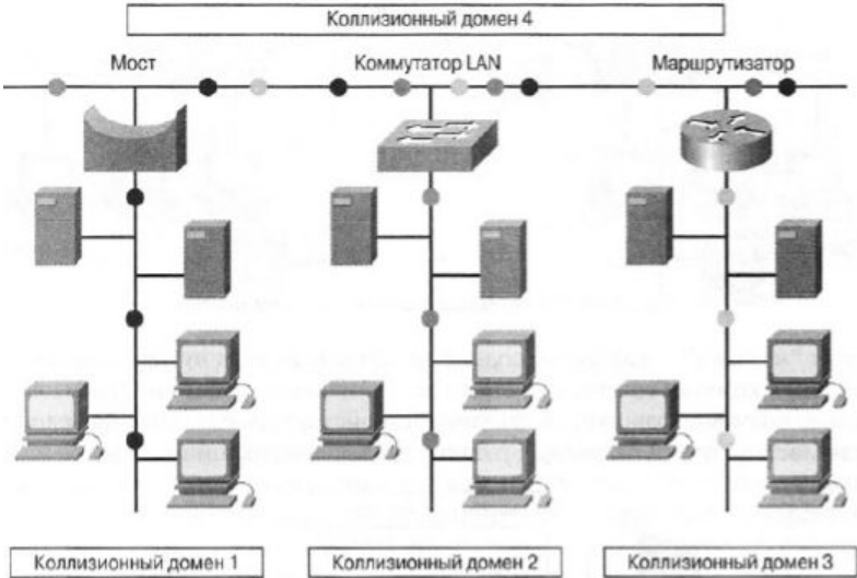
Рис. 5.2. Коллизийные домены
