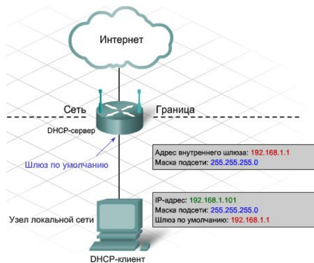
Рис. 3.50. Предоставление адресов DHCP сервером
