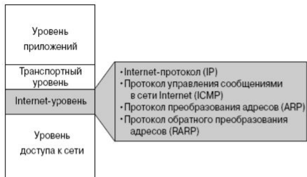
Рис. 3.14. Протоколы Internet-уровня
