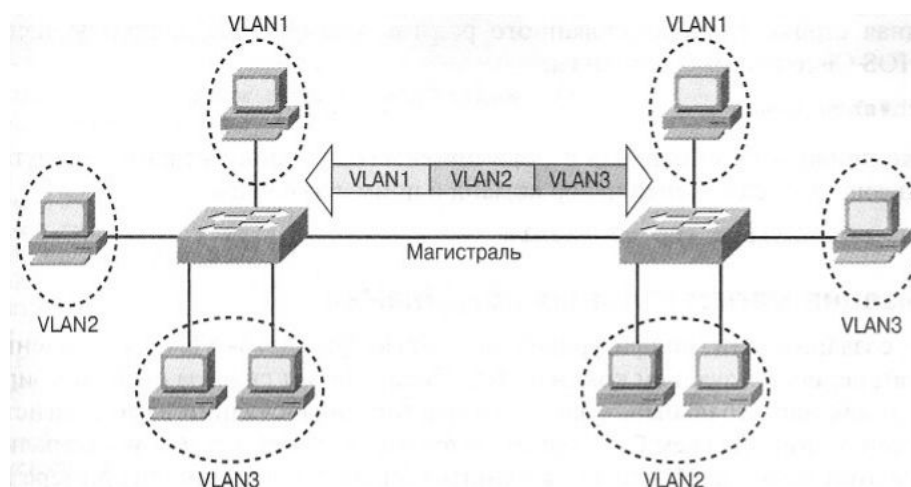
Рис. 6.22. Присвоение тегов
