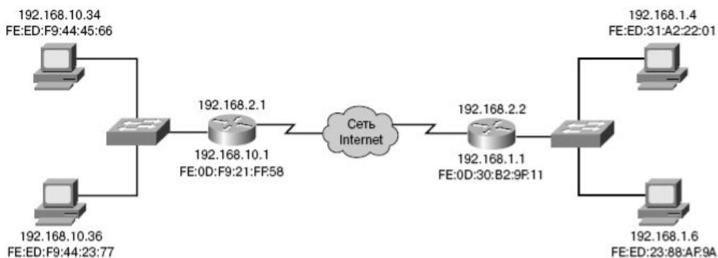
Рис. 3.47. Проблемы преобразования удаленных адресов
