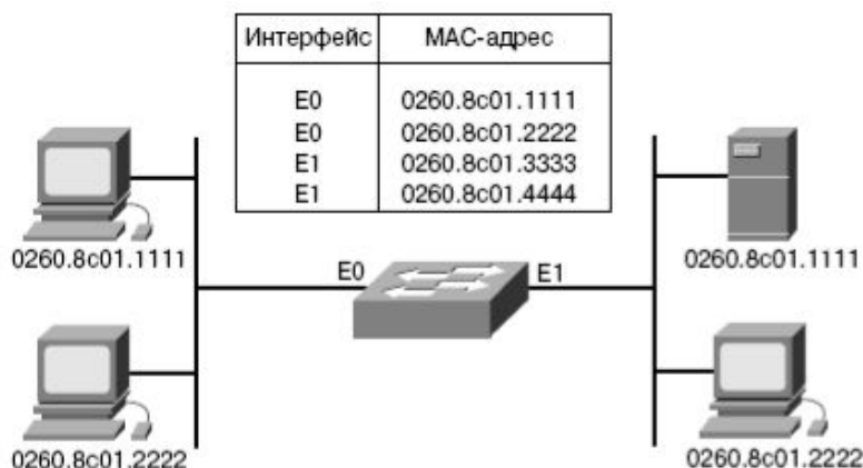
Рис.2.44. Таблица коммутации
