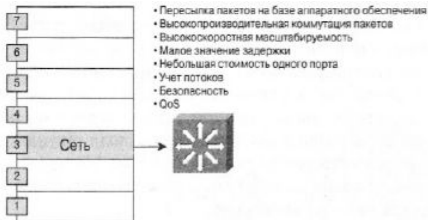
Рис. 15.4. Коммутация на 3-м уровне
