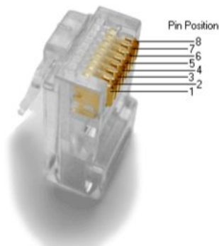
Рис 2.26. Нумерация в штекере 8P8C
