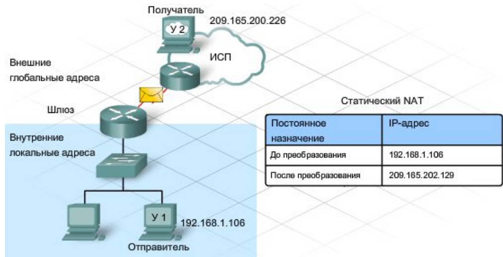
Рис. 9.7. Статическое преобразование NAT
