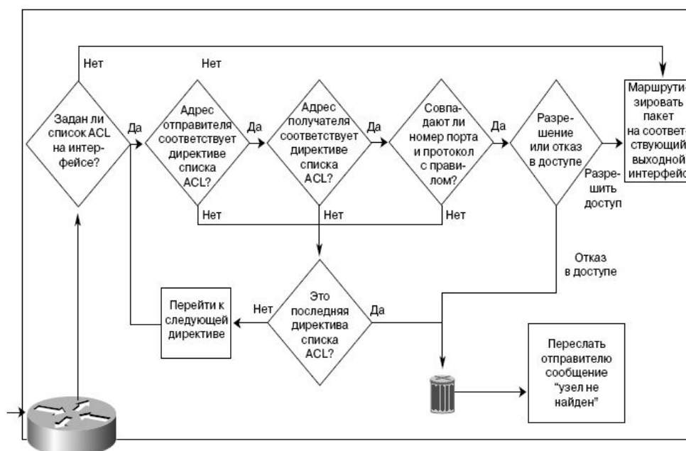
Рис. 8.22. Принцип работы расширенного списка управления доступом
