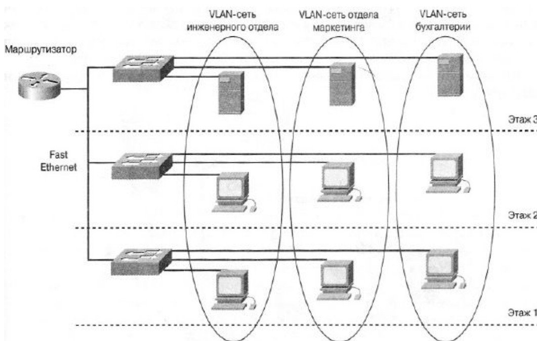
Рис. 6.7. Сети VLAN охватывают определенное физическое пространство
