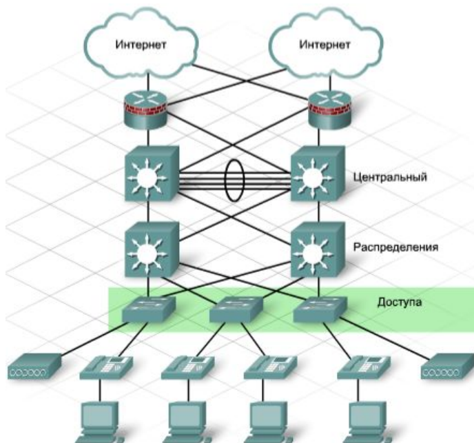
Рис. 11.11. Размещение ACL-списков
