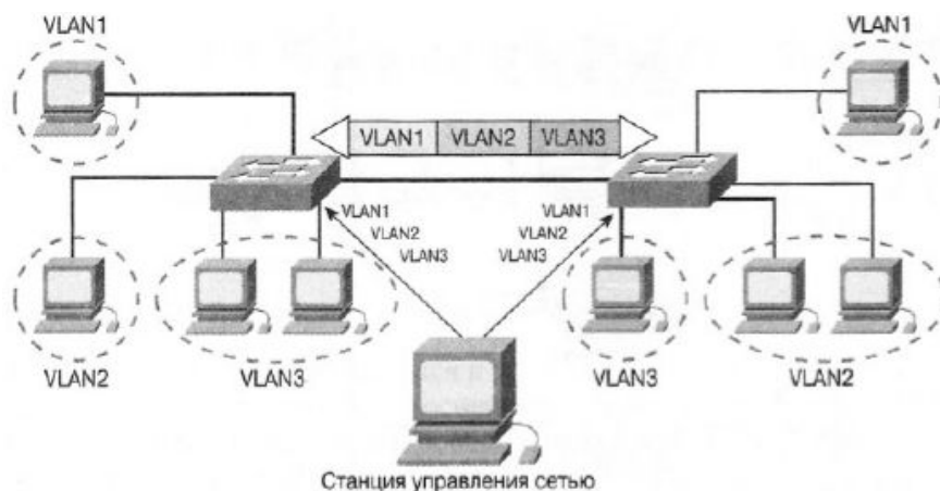
Рис. 6.9. Статические сети VLAN
