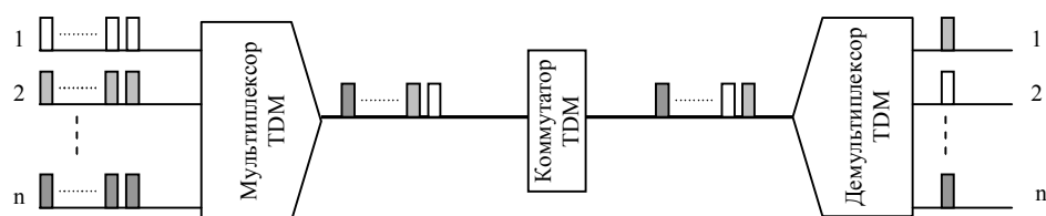
Рис. 3.3. Коммутация на основе разделения во времени
