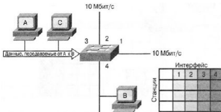
Рис. 5.8. Операции LAN-коммутатора
