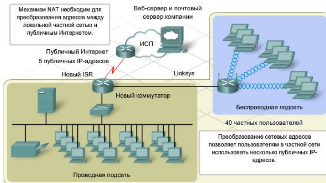
Рис. 9.6. Преобразование сетевых адресов
