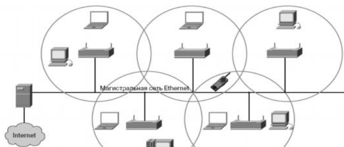
Рис. 10.2. Роуминг
