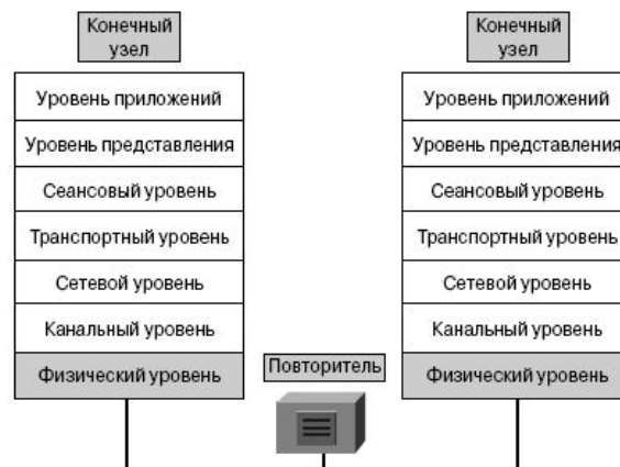
Рис. 2.41. Повторитель соединяет между собой два конечных узла
