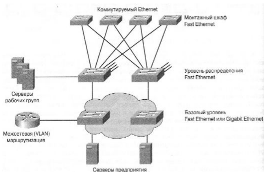
Рис. 6.12. Сквозные VLAN-сети
