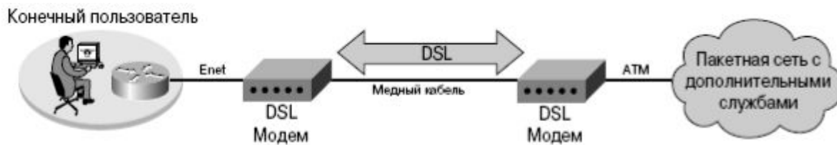
Рис. 7.7. DSL-соединение
