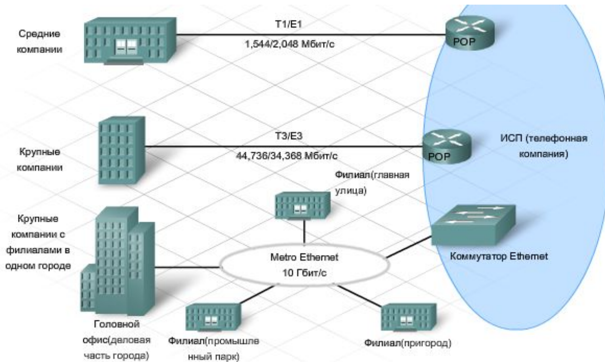
Рис. 9.16. Основные виды подключений с широкой полосой пропускания
