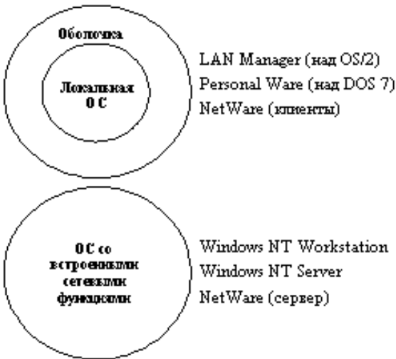
Рис. 2.3. Варианты построения сетевых ОС
