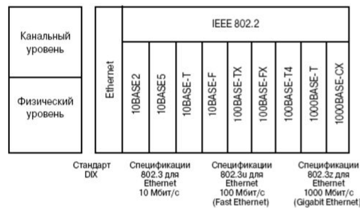
Рис. 2.22. Стандарты LAN-сетей на физическом уровне
