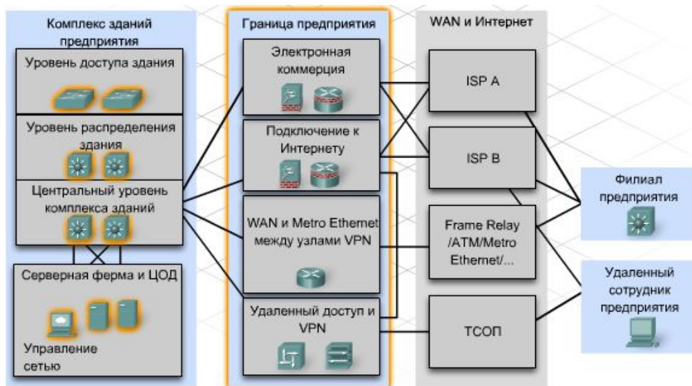
Рис. 11.2. Модульная сетевая архитектура
