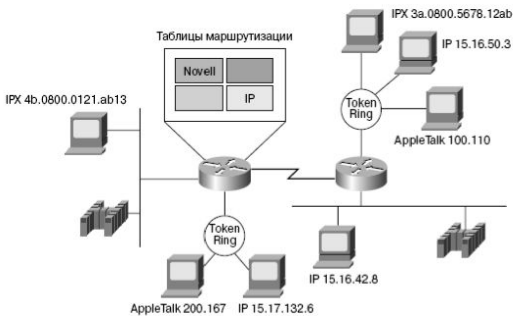
Рис. 8.1. Маршрутизируемые протоколы
