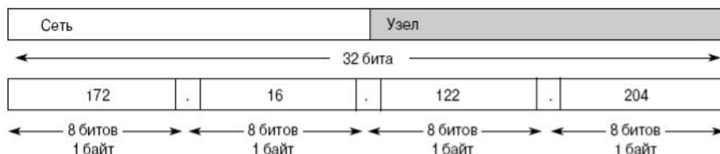
Рис. 3.22. Разделение адреса на сетевую и узловую части
