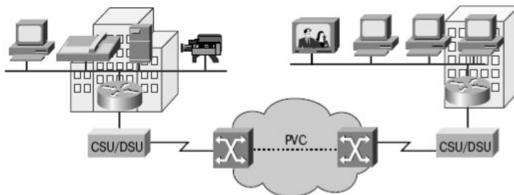
Рис. 7.6. WAN-сеть, в которой используется технология ATM
