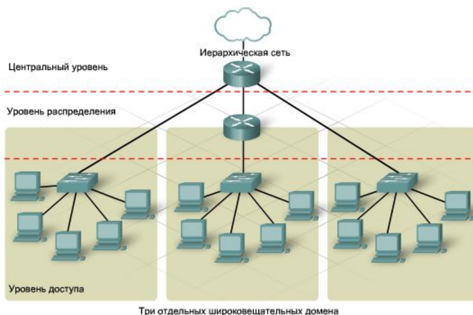
Рис. 3.57. Иерархическая сеть
