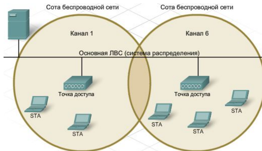
Рис. 10.10. Беспроводные каналы
