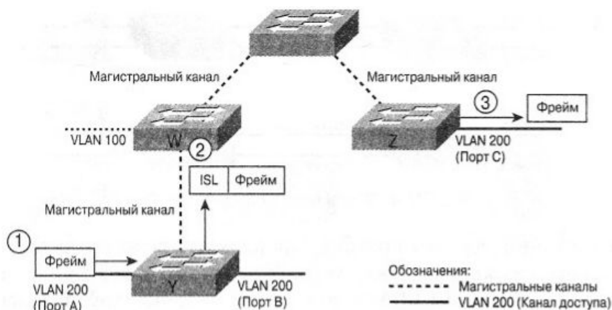
Рис. 6.20. Магистральные каналы
