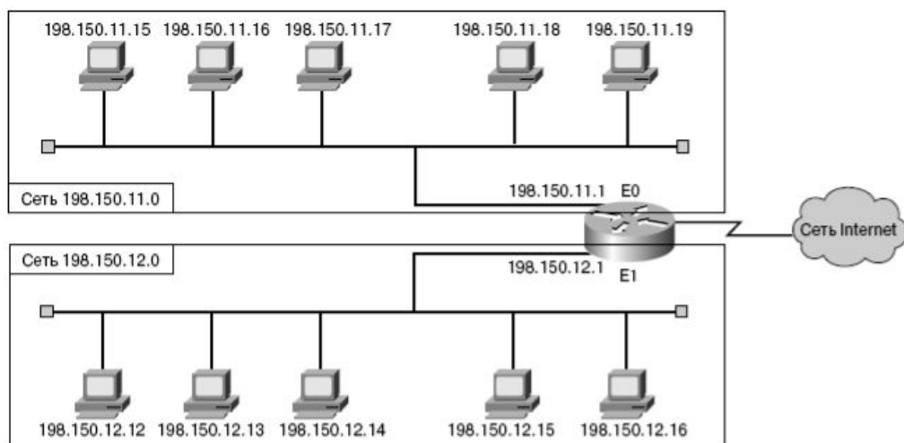
Рис. 3.28. Адрес сети
