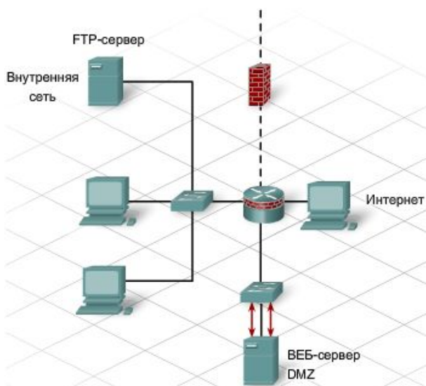
Рис. 12.4. Настройка одного межсетевого экрана
