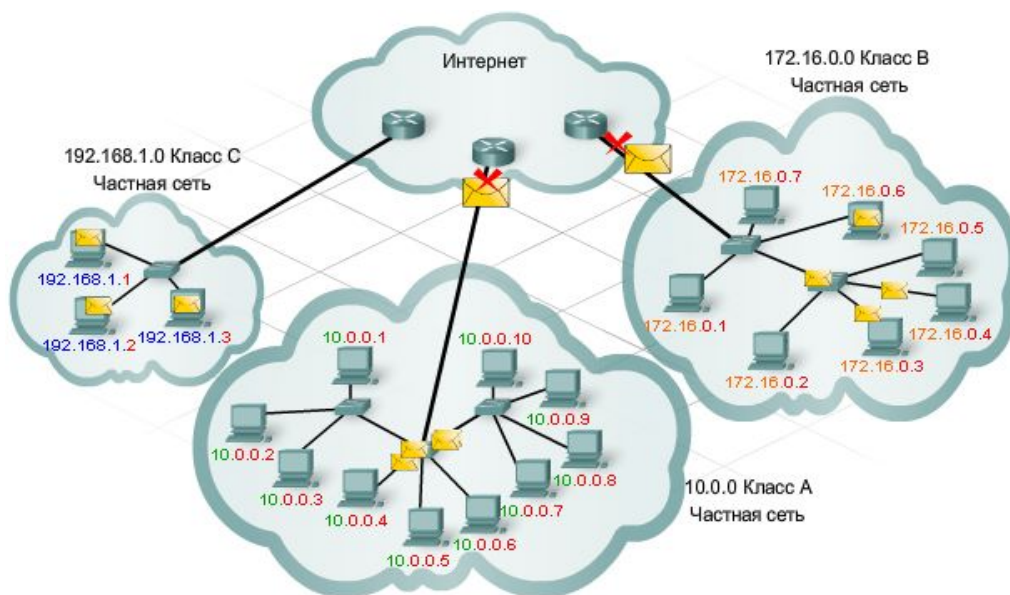
Рис. 3.31. Частные адреса
