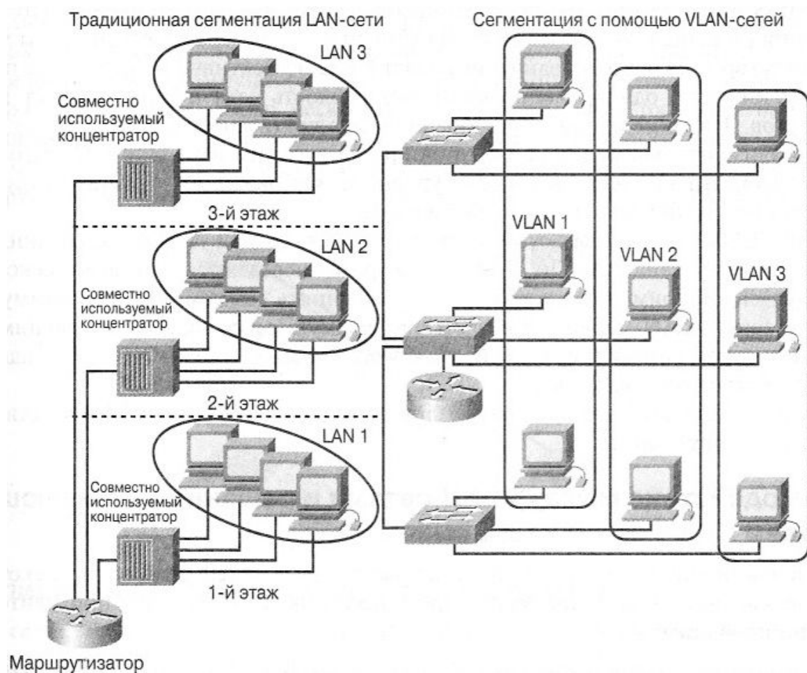
Рис. 6.23. Маршрутизаторы и виртуальные локальные сети VLAN
