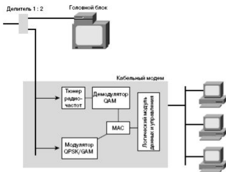
Рис. 7.9. Кабельный модем: двусторонний делитель
