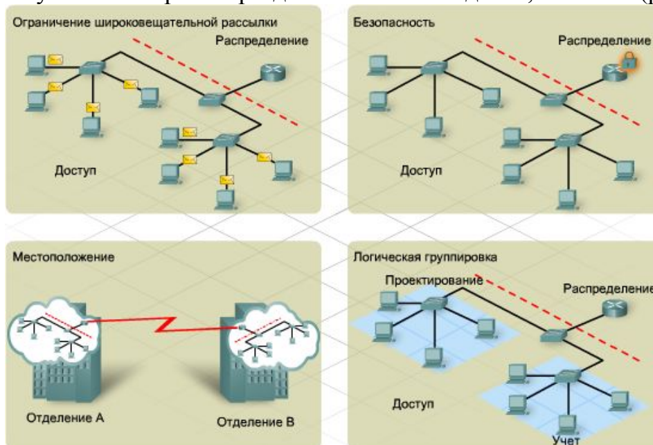
Рис. 3.59. Причины разделения сети на подсети
