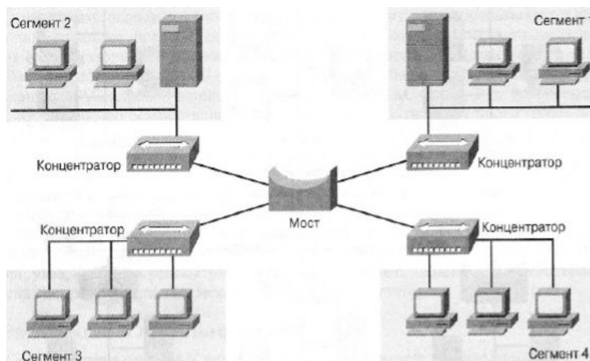
Рис. 5.3. Сегментация с использованием мостов
