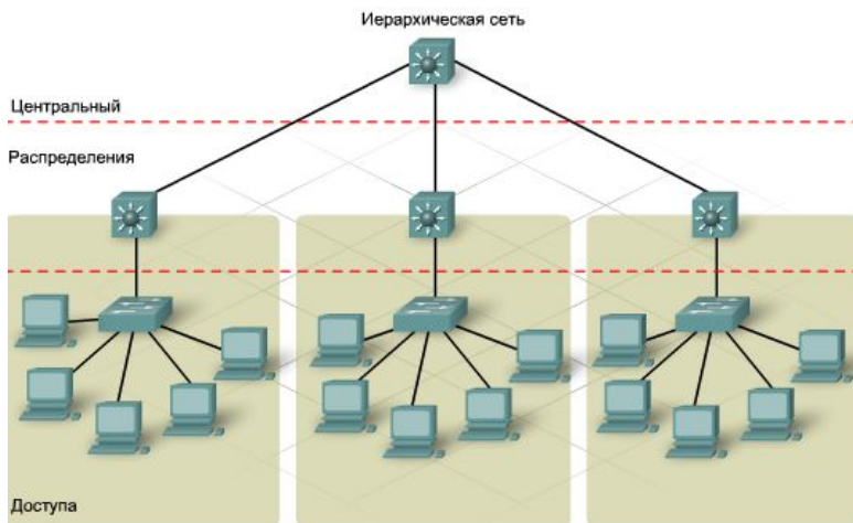
Рис. 11.1. Иерархическая архитектура сети
