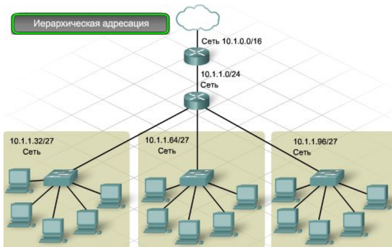
Рис. 3.58. Иерархическая адресация
