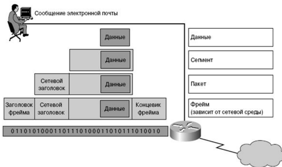
Рис. 8.2. Инкапсуляция
