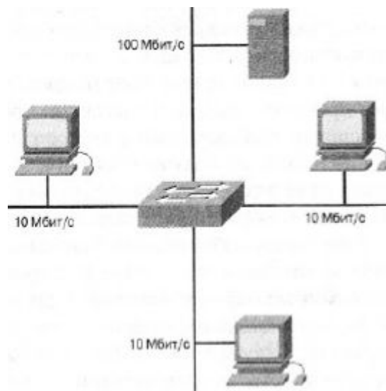
Рис. 5.16. Асимметричная коммутация
