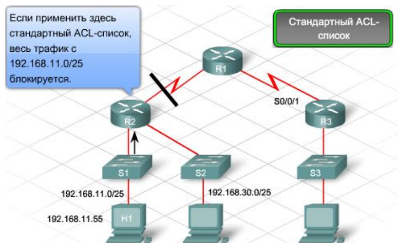
Рис. 11.9. Стандартный ACL-список
