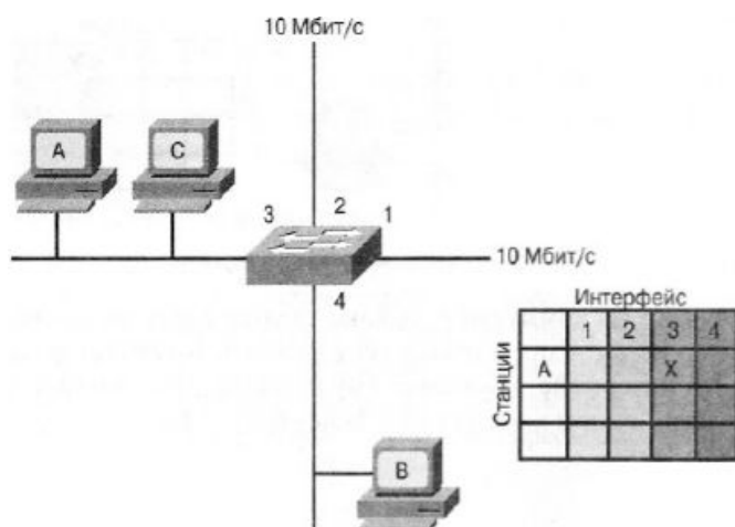
Рис. 5.9. Построение адресной таблицы
