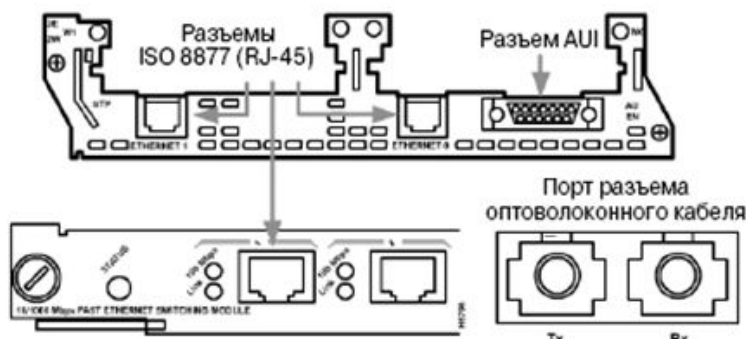
Рис. 2.28. Различные типы разъемов
