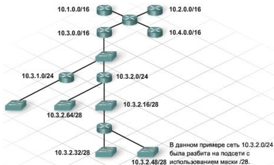
Рис. 3.63. Разбиение на подсети с маской /28
