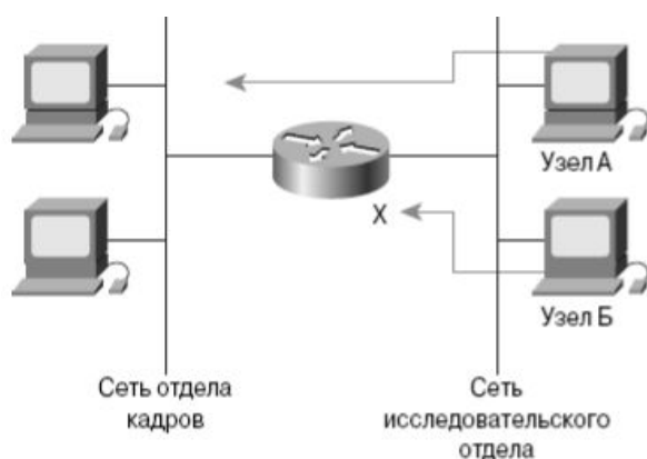
Рис. 8.18. Пример ограничения сетевого трафика
