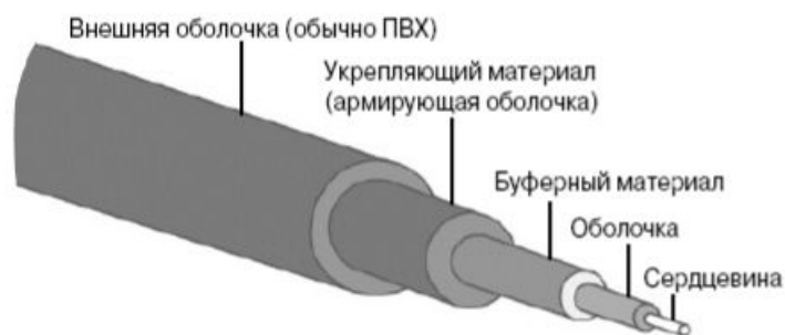
Рис. 2.32. Пять типичных компонентов оптоволоконного кабеля
