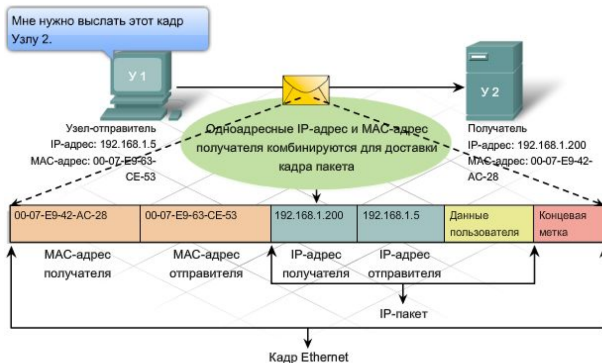
Рис. 3.54. Одноадресная рассылка
