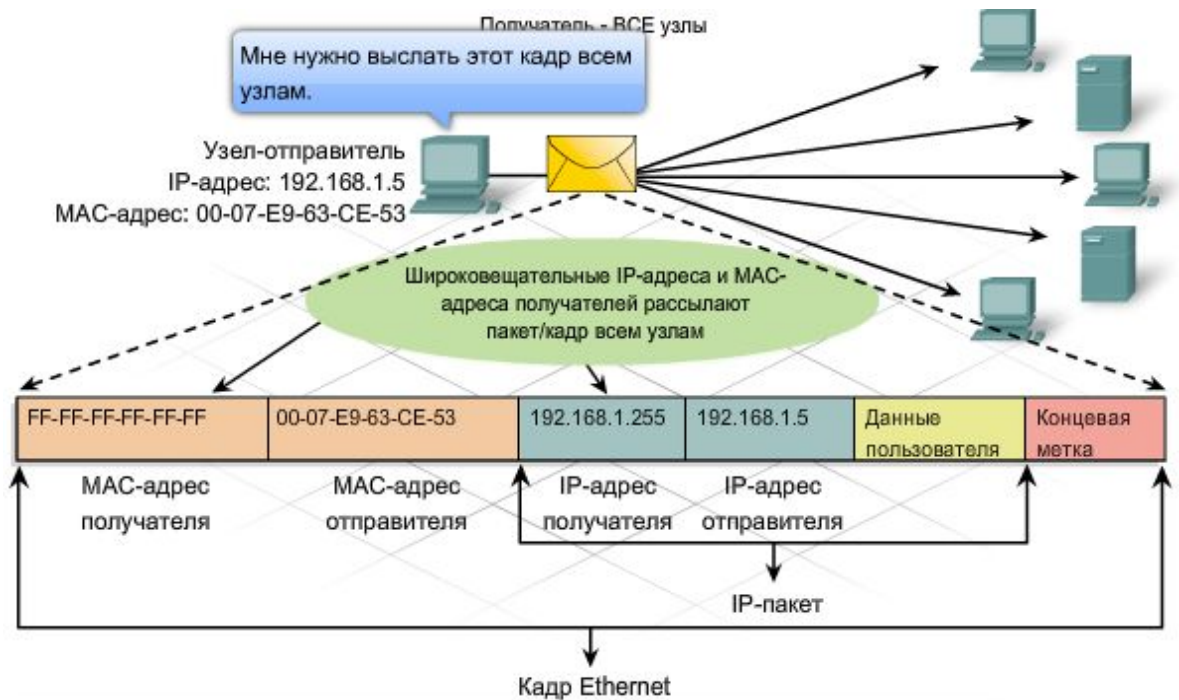
Рис. 3.55. Широковещательная рассылка
