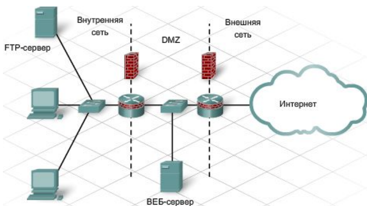
Рис. 12.5. Настройка двух межсетевых экранов
