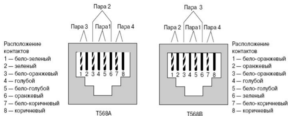
Рис. 2.27. Стандарты Ethernet для разъемов RJ-45
