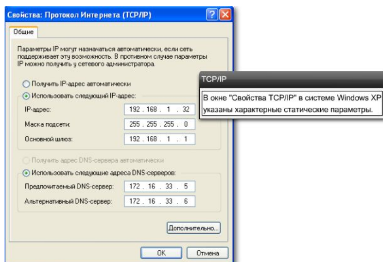
Рис. 3.40. Статическое назначение IP-адресов
