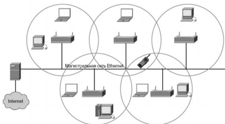
Рис. 2.38. Роуминг
