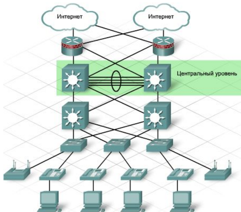
Рис. 11.3. Центральный уровень сети
