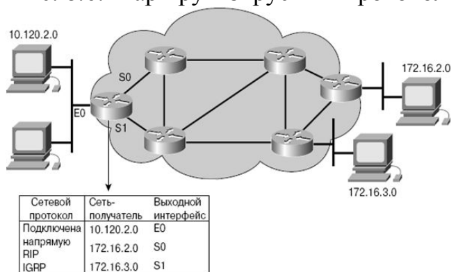
Рис. 8.7. Протокол маршрутизации
