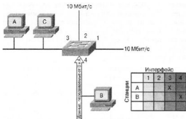
Рис. 5.11. Ответ на лавинную рассылку
