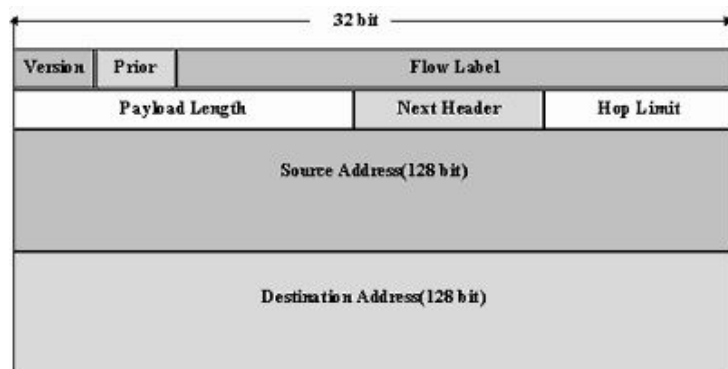
Рис.3.33. Заголовок IPv6
