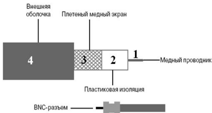
Рис. 2.23. Коаксиальный кабель
