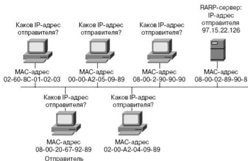
Рис. 3.43. Схема работы протокола RARP
