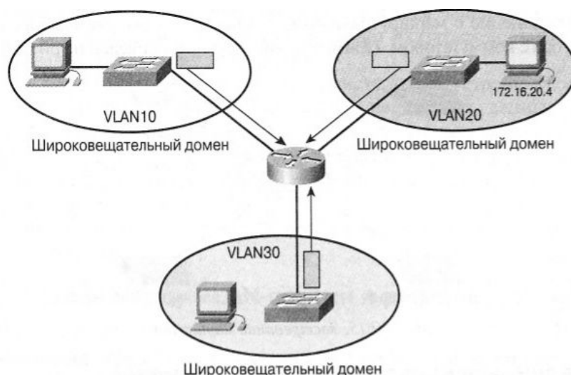
Рис. 6.25. Изолированные широковещательные домены
