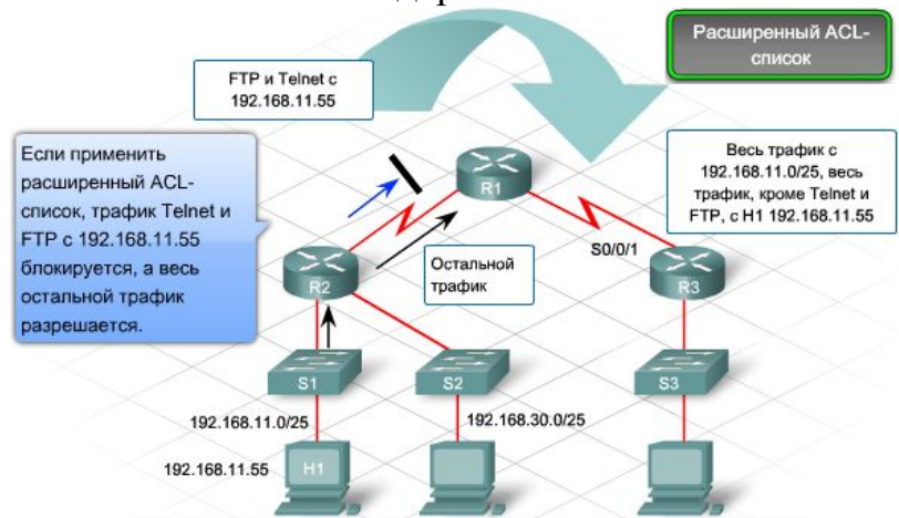
Рис. 11.10. Расширенный ACL-список
