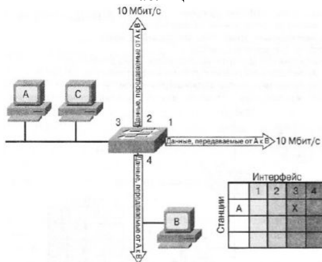
Рис. 5.10. Лавинная рассылка на все порты
