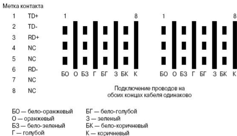
Рис. 2.30. Прямой кабель UTP
