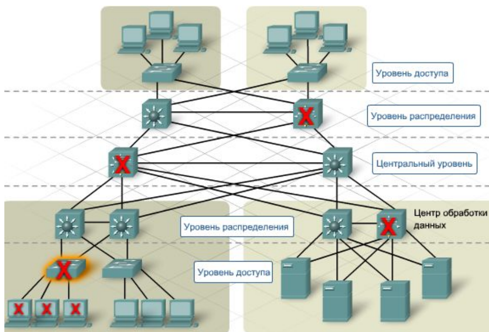
Рис. 11.7. Ограничение размера доменов возникновения сбоя
