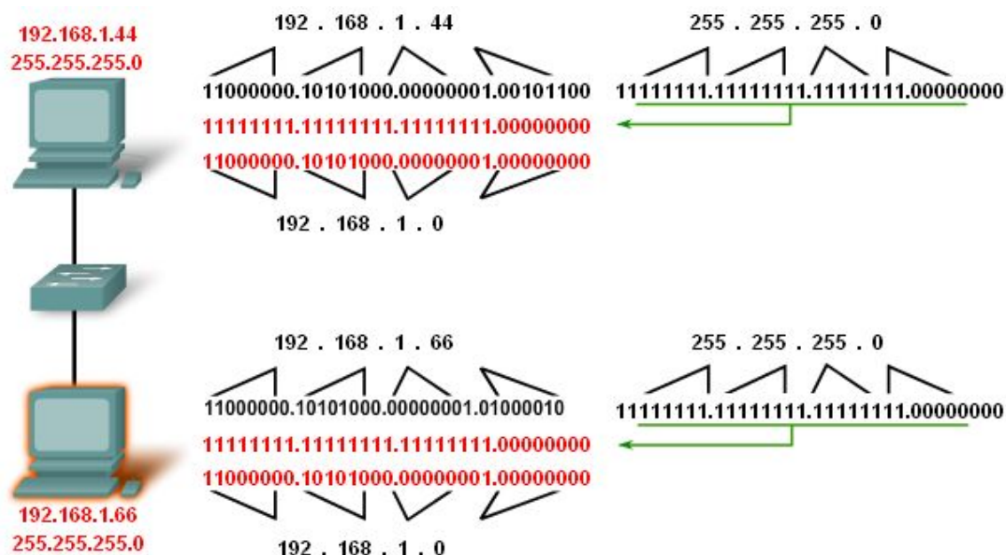
Рис. 3.37. Взаимодействие IP-адресов и масок подсети
