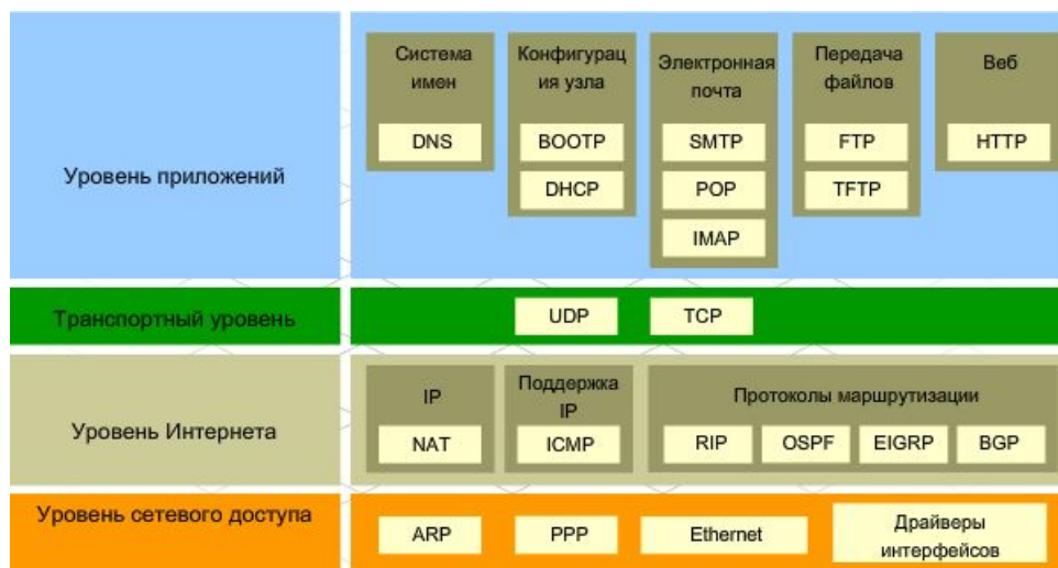
Рис 3.9. Структура стека протоколов TCP/IP
