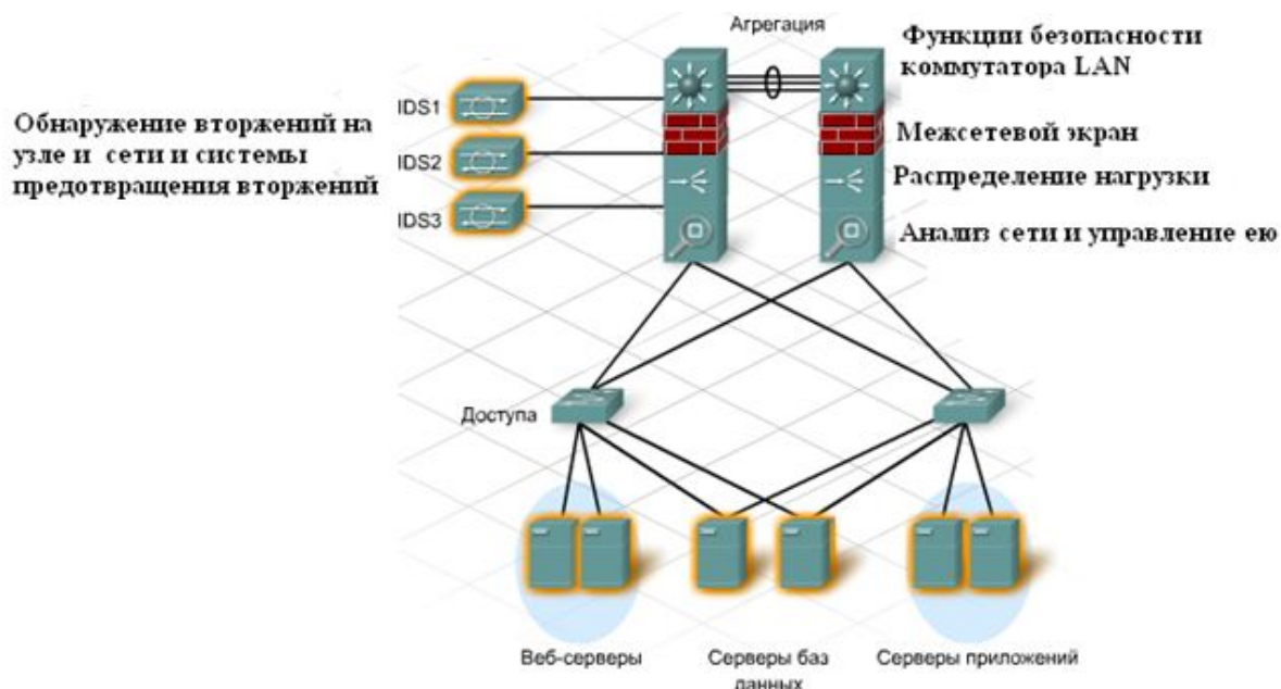
Рис. 12.3. Защита серверных ферм
