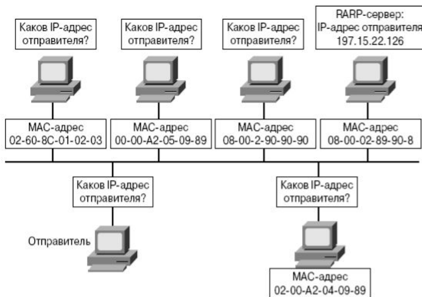
Рис. 3.41. Назначение IP-адресов с помощью протокола RARP
