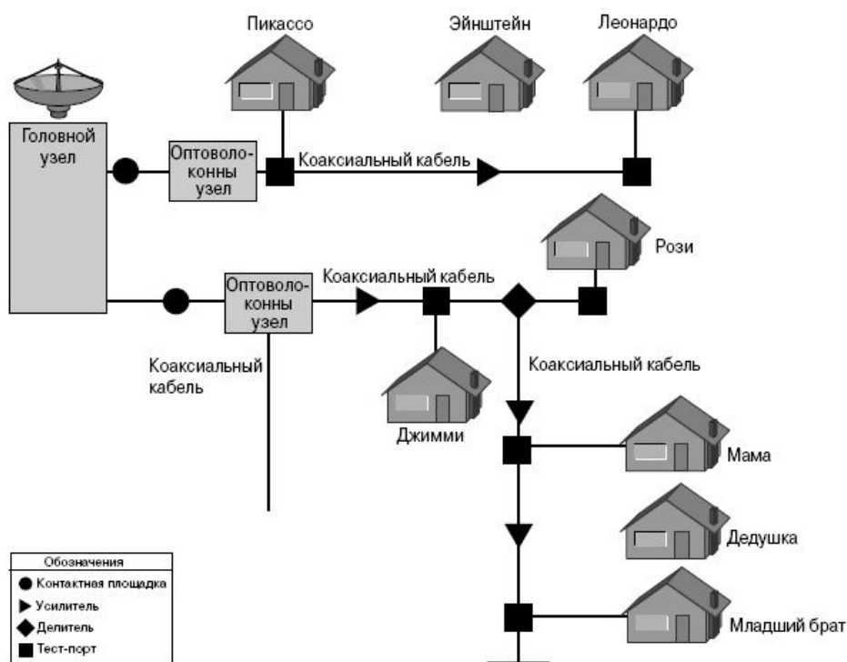
Рис. 7.8. Использование кабельных модемов
