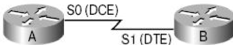
Рис. 2.48. Непосредственное последовательное соединение маршрутизаторов
