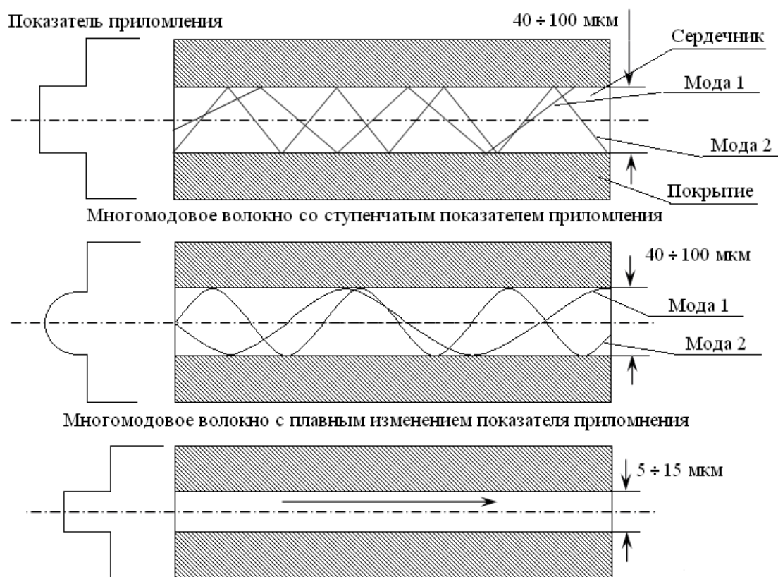
Рис.2.33. Типы оптического кабеля
