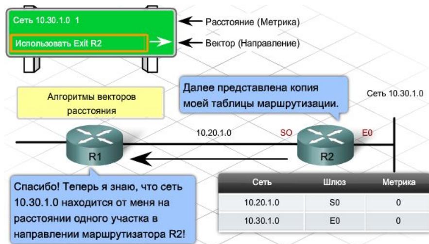
Рис. 8.9. Определение вектора расстояния
