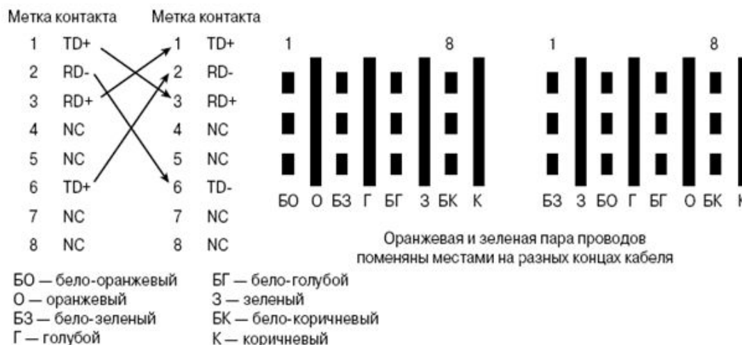
Рис. 2.31. Перекрещенный кабель UTP
