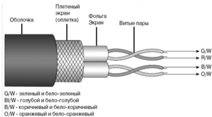
Рис. 2.24. Экранированный кабель на основе витой пары
