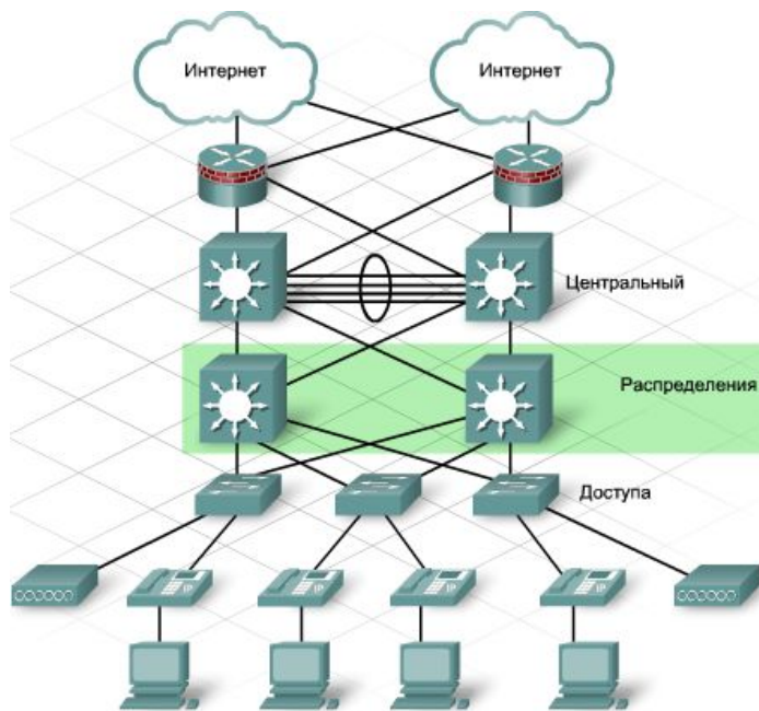
Рис. 11.5. Уровень распределения
