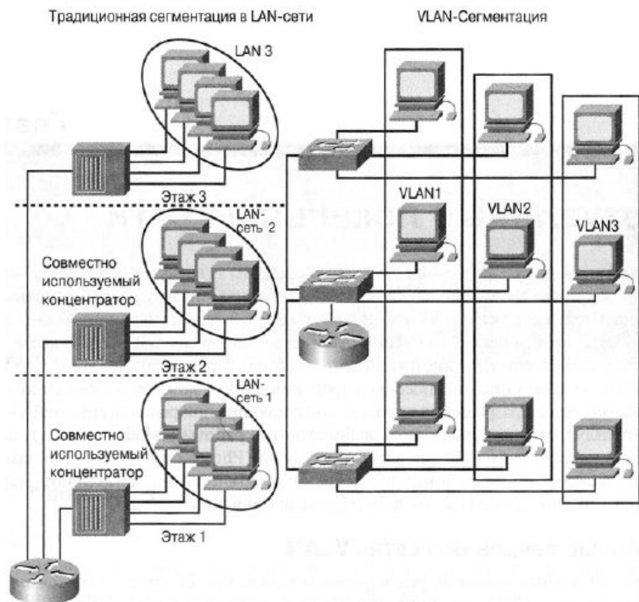
Рис. 6.5. Сети VLAN и физические границы
