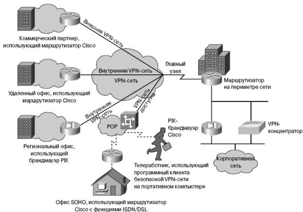
Рис. 2.8. Технологии VPN-сетей
