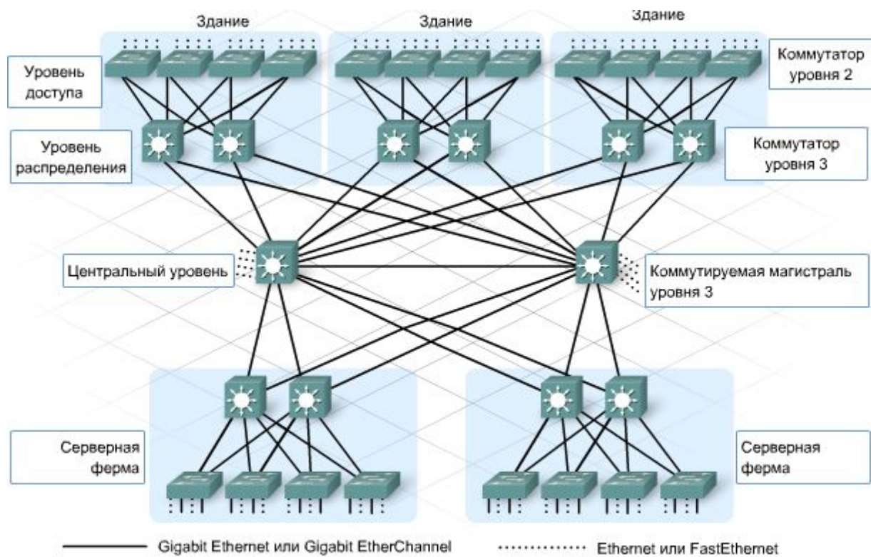
Рис. 11.4. Резервные каналы в ячеистой топологии
