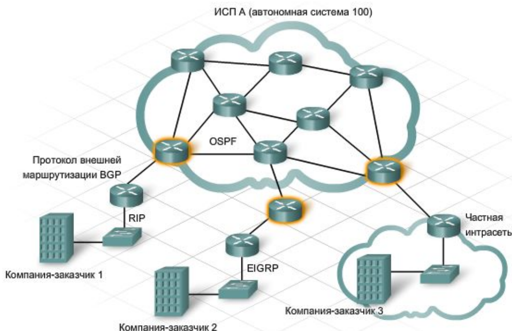
Рис. 8.15. Внешние протоколы маршрутизации и Интернет-провайдеры
