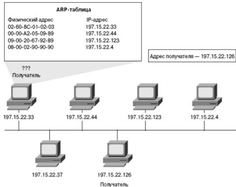
Рис. 3.49. ARP-таблицы
