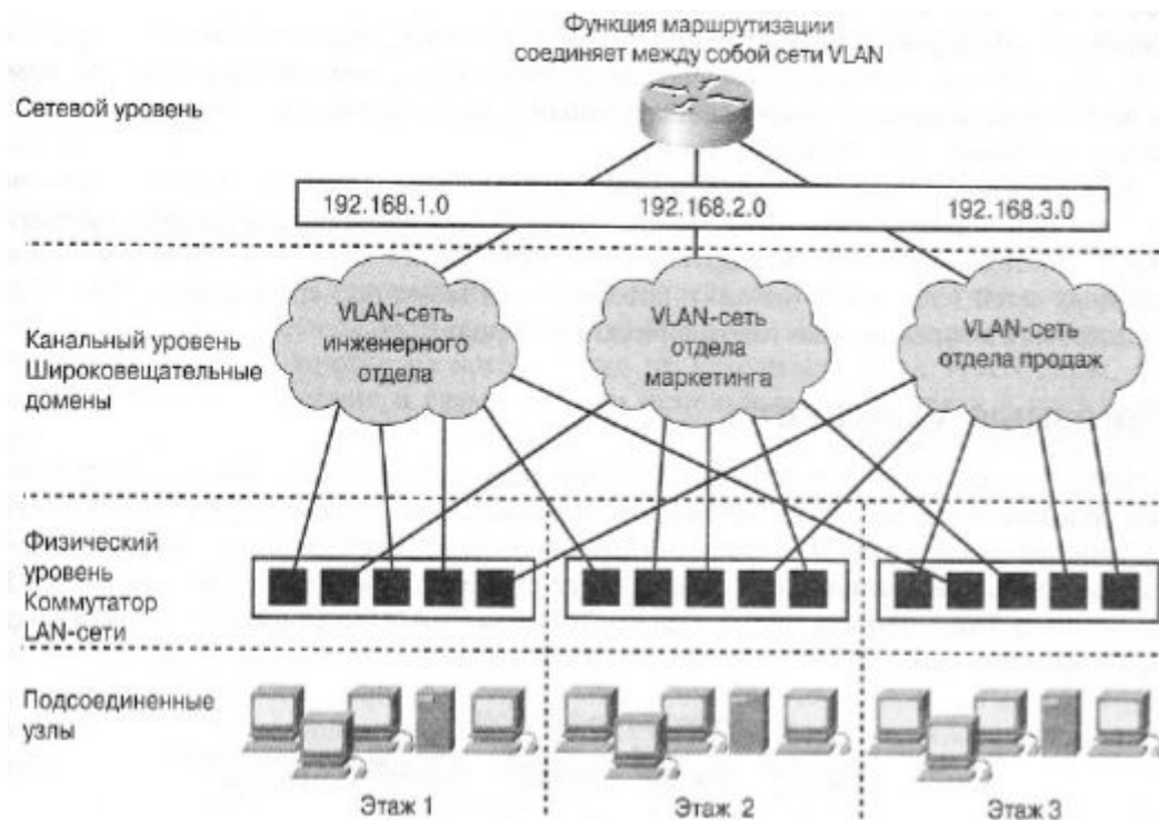
Рис. 6.11. Статические виртуальные сети на основе портов
