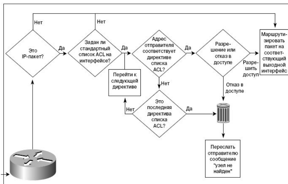
Рис. 8.21. Принцип работы стандартных списков управления доступом
