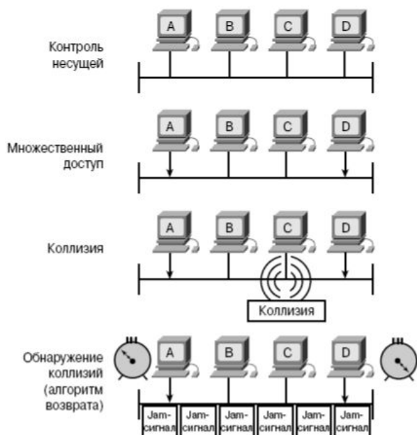
Рис. 4.6. Метод доступа CSMA/CD
