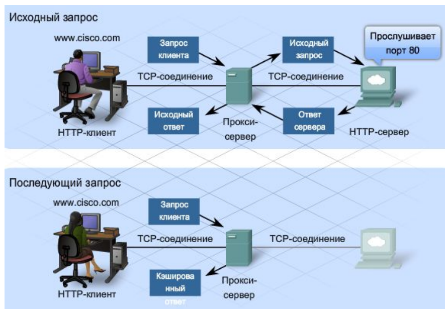
Рис. 9.28. Типы запросов
