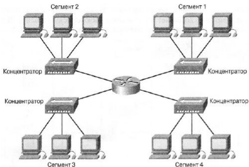
Рис. 5.6. Сегментация с использованием маршрутизаторов
