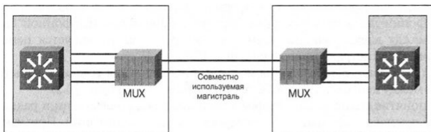
Рис. 6.19. Магистральные каналы, использующие мультиплексирование с разделением фреймов
