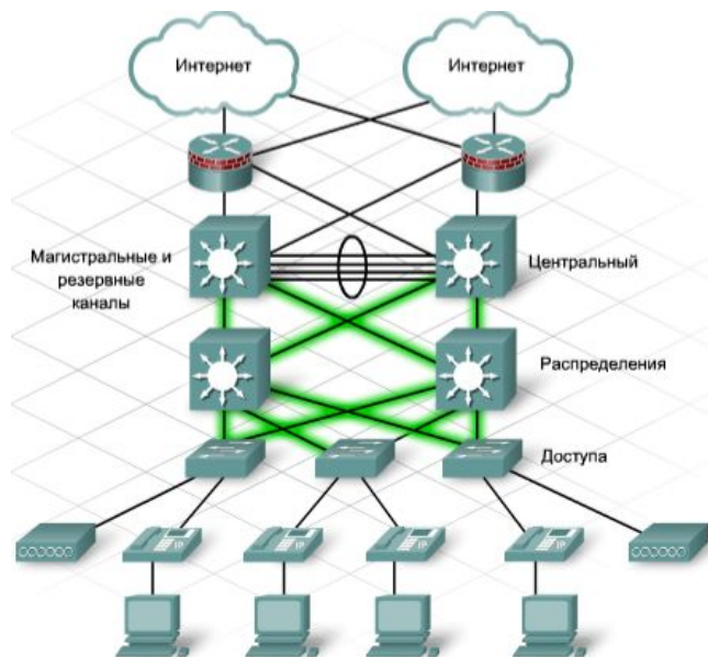
Рис. 11.6. Магистральные каналы
