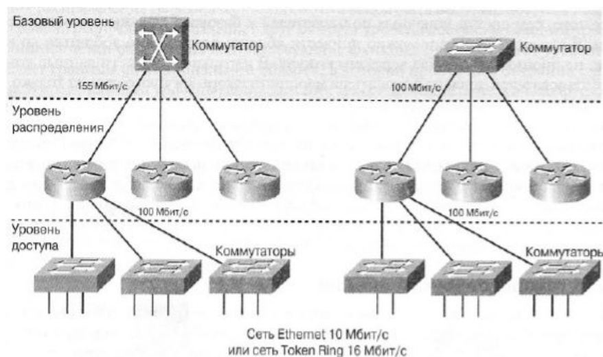
Рис. 6.4. Коммутаторы базового уровня
