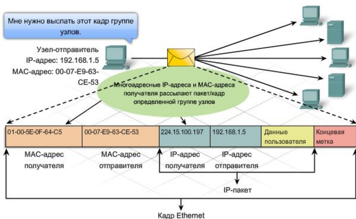
Рис. 3.56. Многоадресная рассылка
