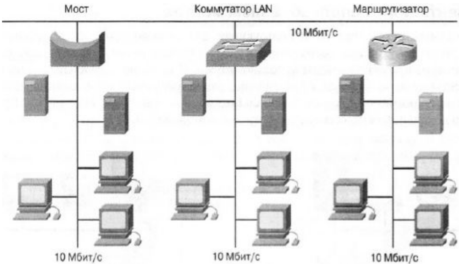
Рис. 5.1. Сегментированная сеть
