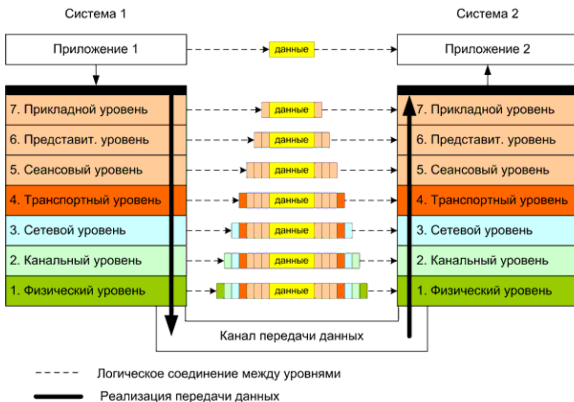
Рис. 3.7. Модель OSI
