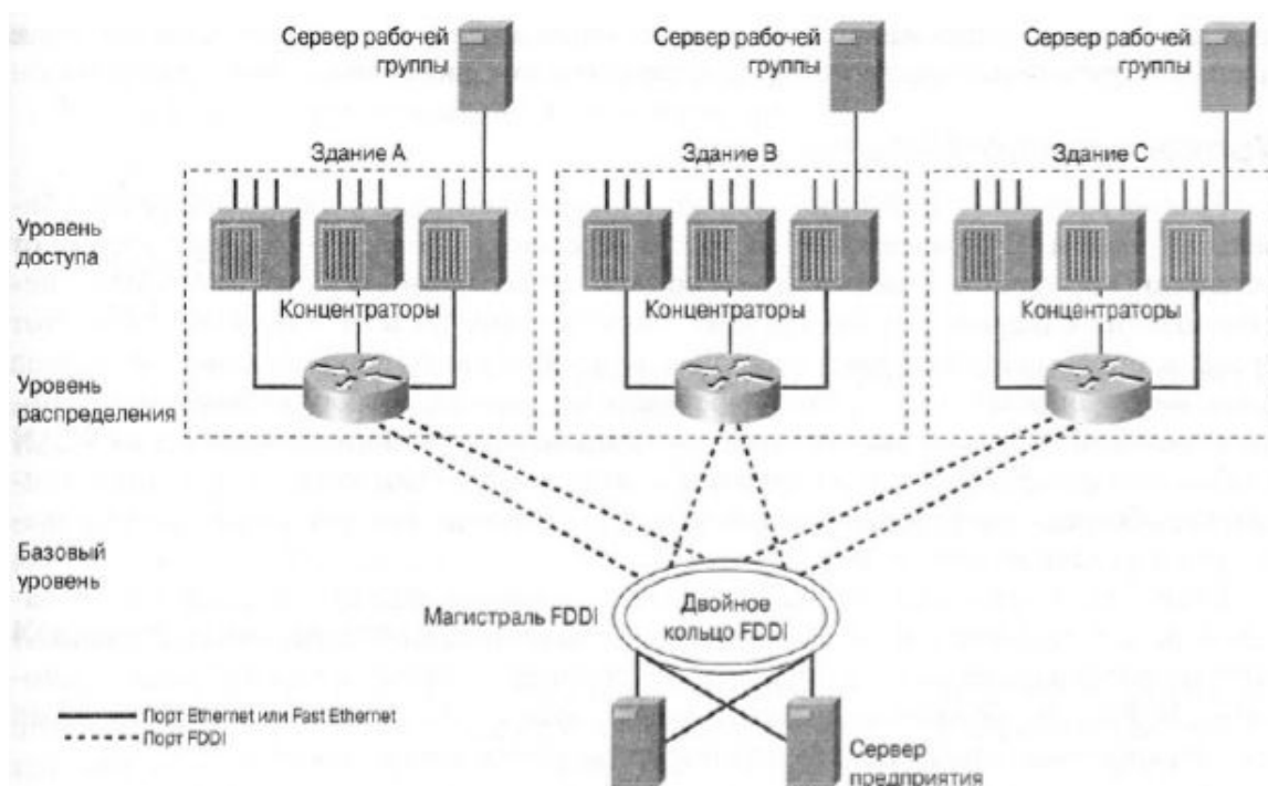
Рис. 6.1. Иерархическая модель проектирования сети
