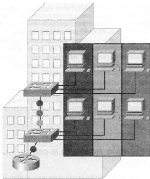
Рис. 6.6. Проектирование виртуальной локальной сети
