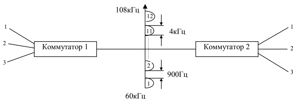
Рис. 3.2. Коммутация на основе частотного уплотнения
