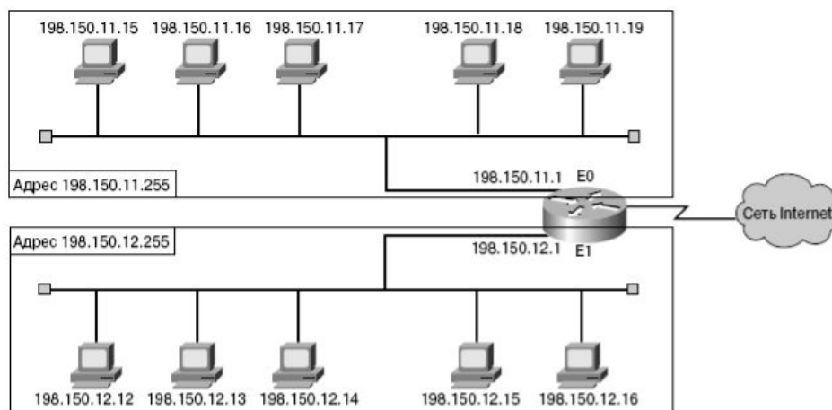
Рис. 3.29. Широковещательный адрес
