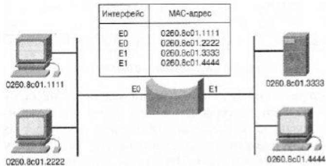
Рис. 5.4. Пример адресной таблицы
