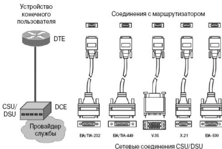
Рис. 2.45. Различные варианты последовательных соединений WAN
