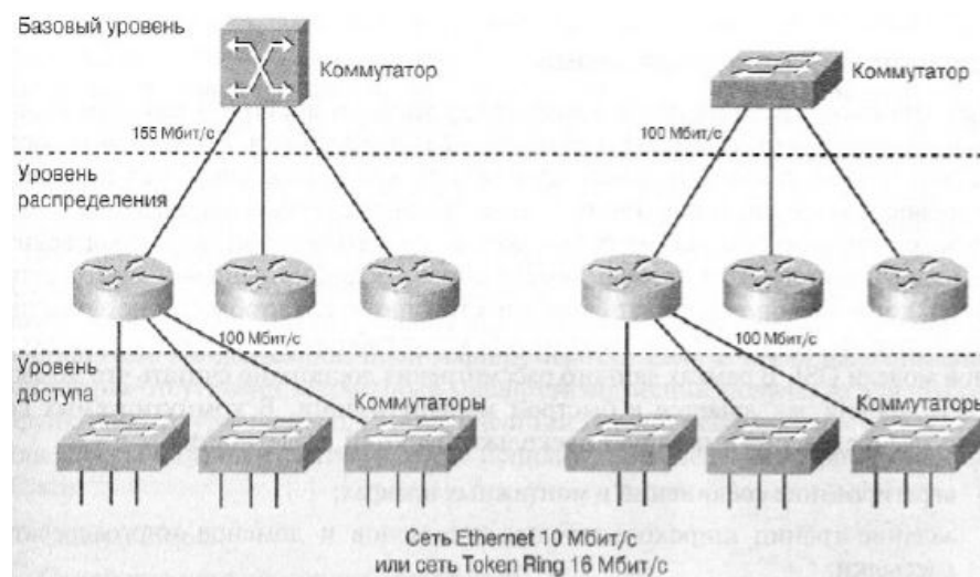
Рис. 6.2. Коммутаторы уровня доступа
