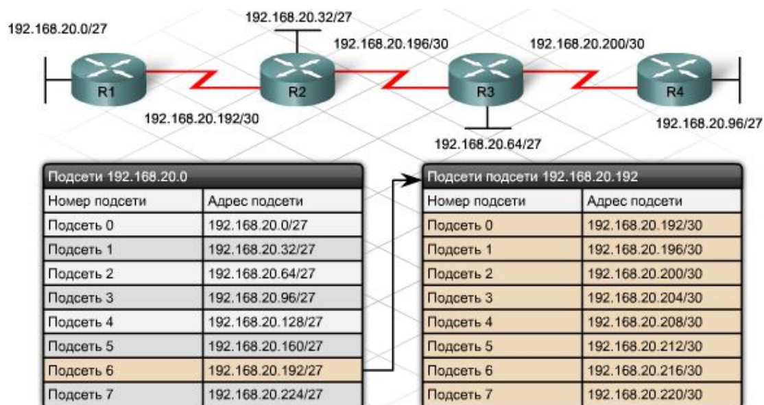
Рис. 3.60. Расбиение на подсети при помощи VLSM
