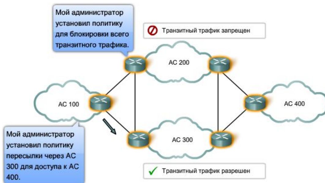
Рис. 8.16. Транзит трафика через автономные системы
