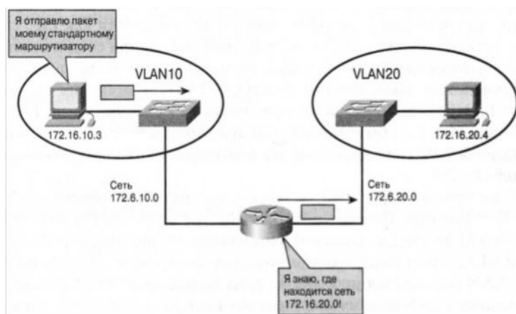
Рис. 6.26. Стандартный шлюз
