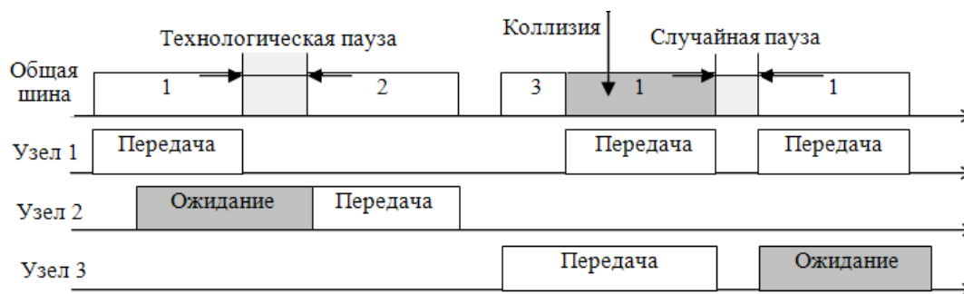
Рис.4.1. Пояснение метода случайного доступа CSMA/CD
