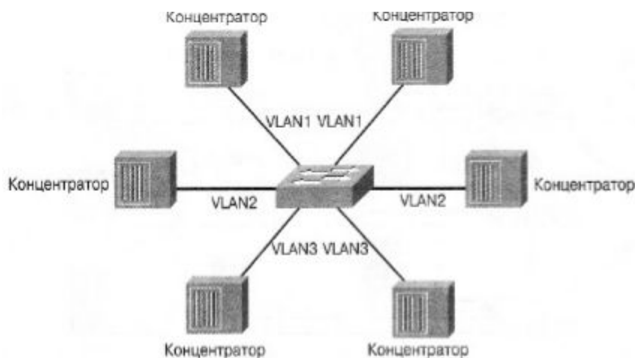
Рис. 6.16. Использование существующих концентраторов в среде коммутации сети VLAN
