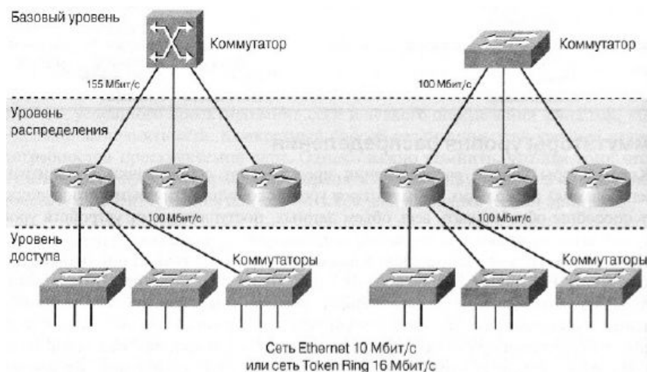
Рис. 6.3. Коммутатор уровня распределения
