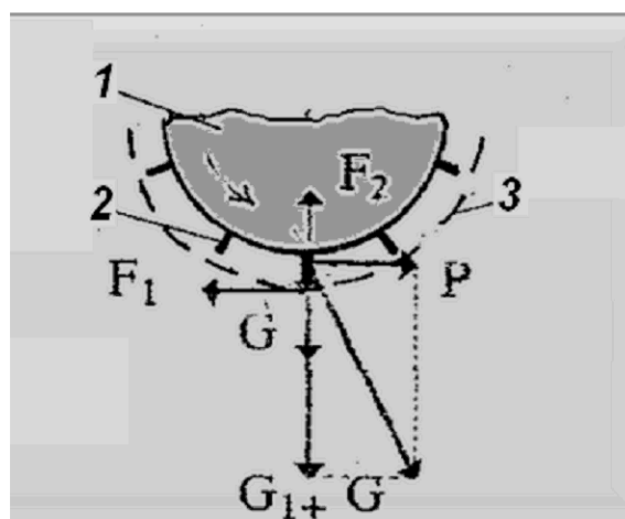
5.2-rasm. Baraban qozig'ning paxta bo'lakchasiga ta'sir qilish sxemasi
