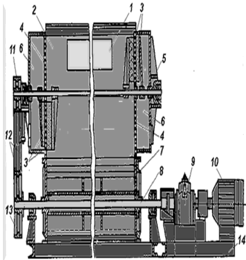
4.1-rasm. CC-15A separatorning bo'ylama kesim ko'rinishi
