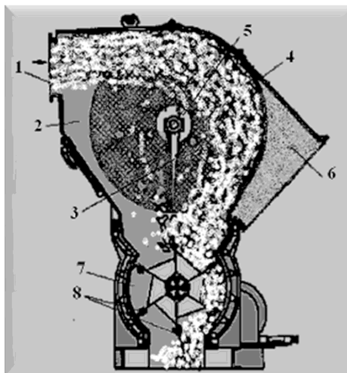
4.2-rasm. CC-15A separatorining ko'ndalang kesim ko'rinishi
