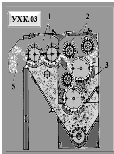
6.4-rasm. YXK agregti YXK.01 va. YXK.03 seksiyasilarining ko'ndalang qirqim ko'rinishi
