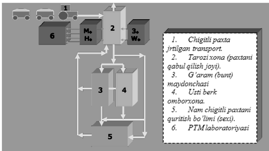
2.5-rasm. Namunaviy (tipovoy) paxta tayyorlash punkting umumiy texnologik jarayon sxemasi
