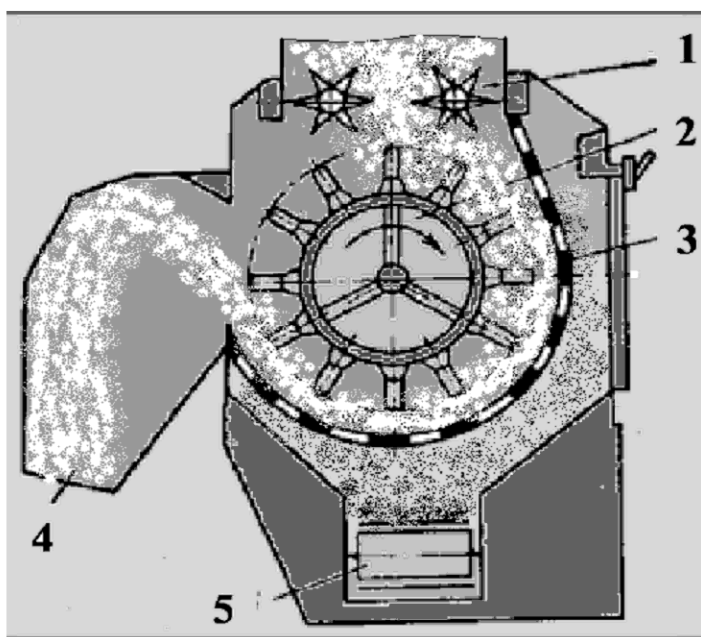
7.1-rasm. ИД - ta'minlagichning ko'ndalang qirgim sxemasi
