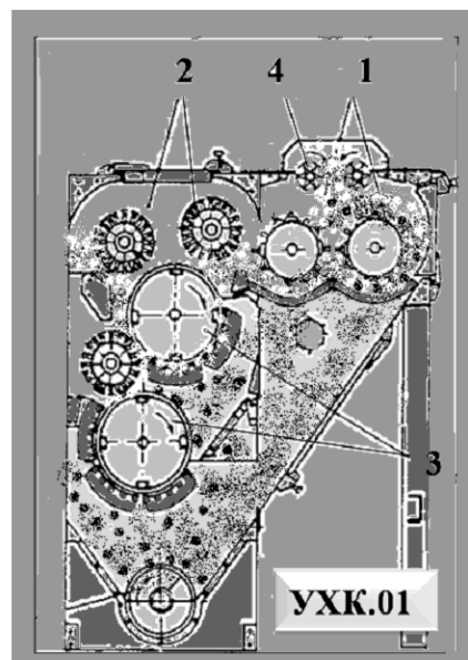
6.4-rasm. YXK agregti YXK.01 va. YXK.03 seksiyasilarining ko'ndalang qirqim ko'rinishi
