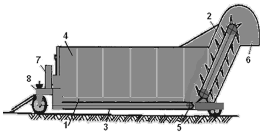
3.8-rasm. XIII qabul qilish - uzatish qurilmasining sxemasi
