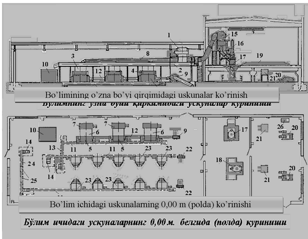
2.2-rasm . Bir qatorli arrali jinlar o'rnatilgan bosh binoda asosiy texnologik uskunalarning joylashish sxemasi
