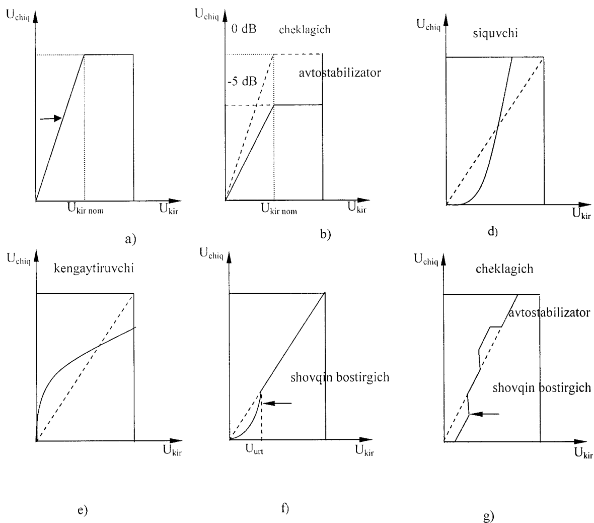
3 - rasm. Kuchaytiruvchi cheklagich (a). avtostabilizator (b). ekspander(d). kompressor (e). bo'sag'a tovush bostirgich (f). murakkab avtoboshqargich (g) larning amplituda tavsiflari.
